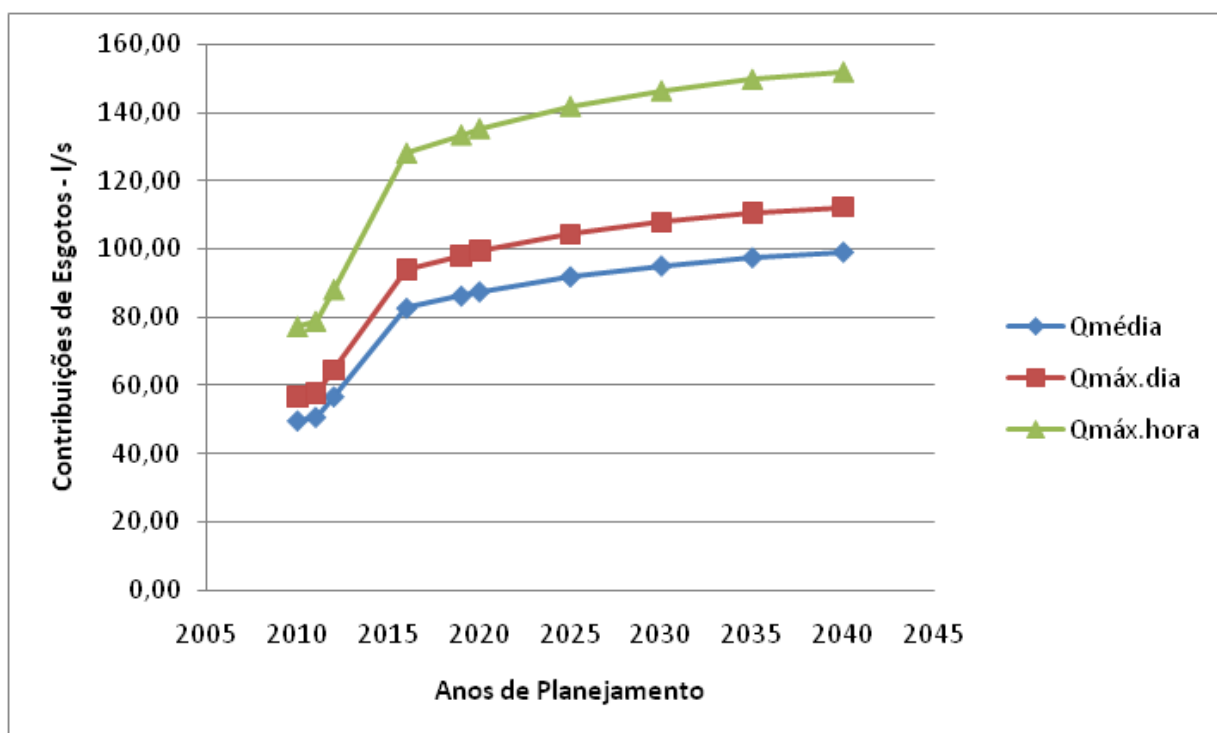
Gráfico 2.5 – evolução das contribuições de esgotos
