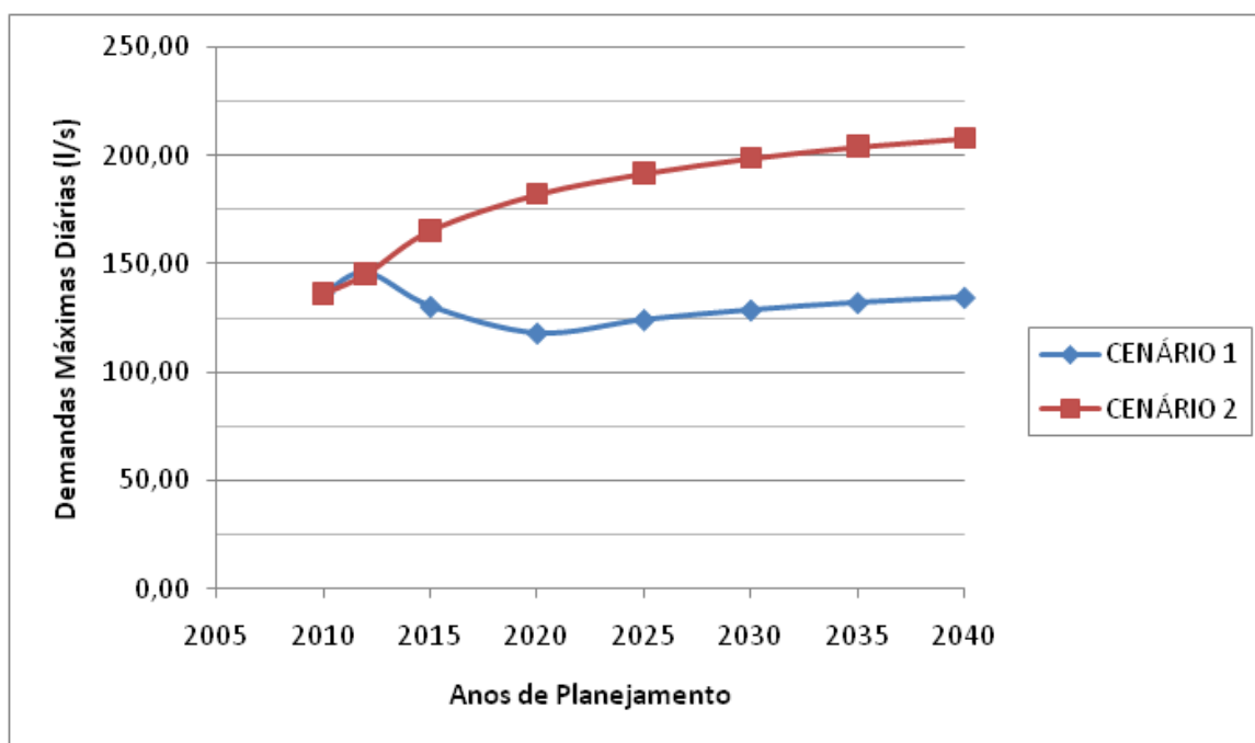
Gráfico 3.1 – comparação das demandas disponibilizadas para a distribuição
