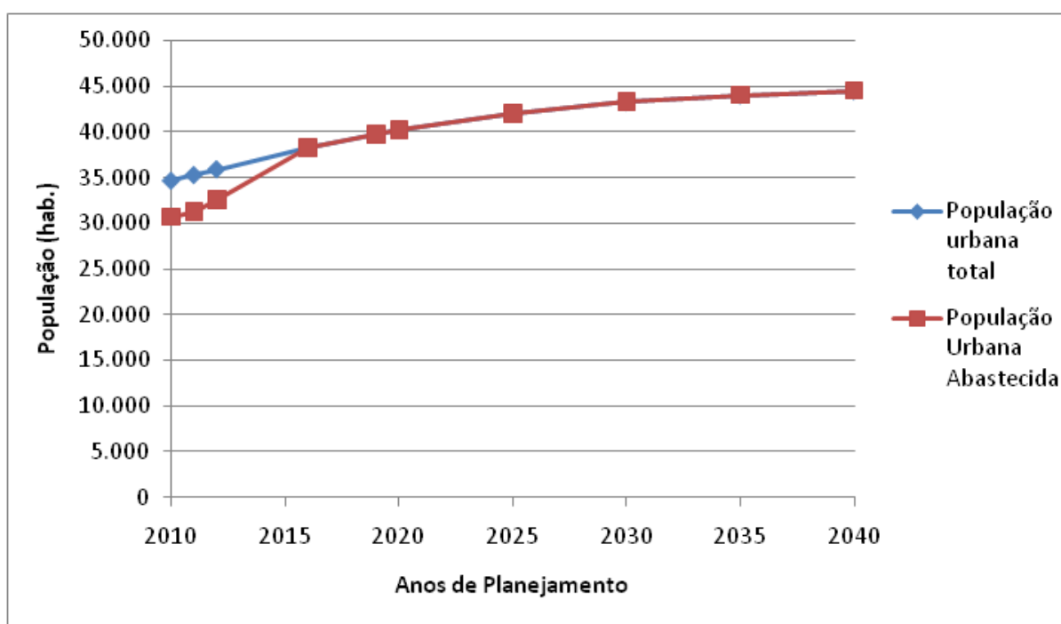
Gráfico 2.1 – Evolução da População Urbana Total X População Urbana Abastecida
