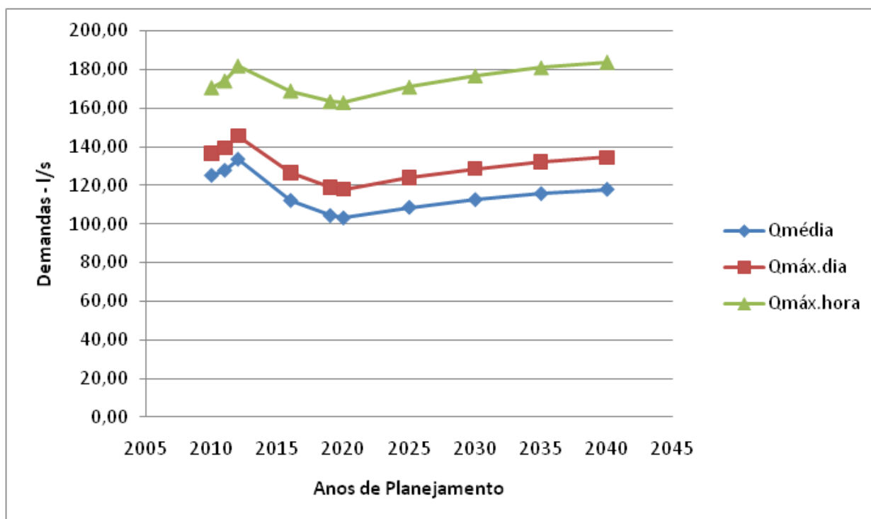
Gráfico 2.2 – Evolução das Demandas/Vazões Disponibilizadas para Distribuição
