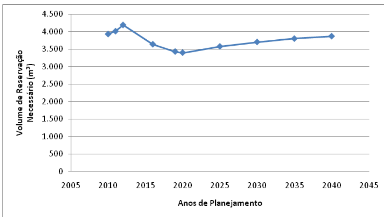
Gráfico 2.3 – Evolução dos Volumes de Reservação Necessários (m³)
