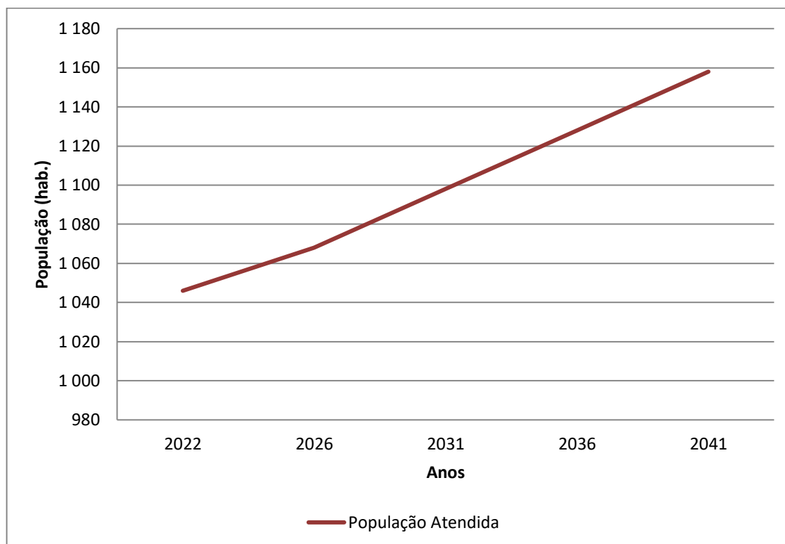
Gráfico 7.10 - População Atendida (hab.) x Anos de Planejamento – Distrito Santa Rita
