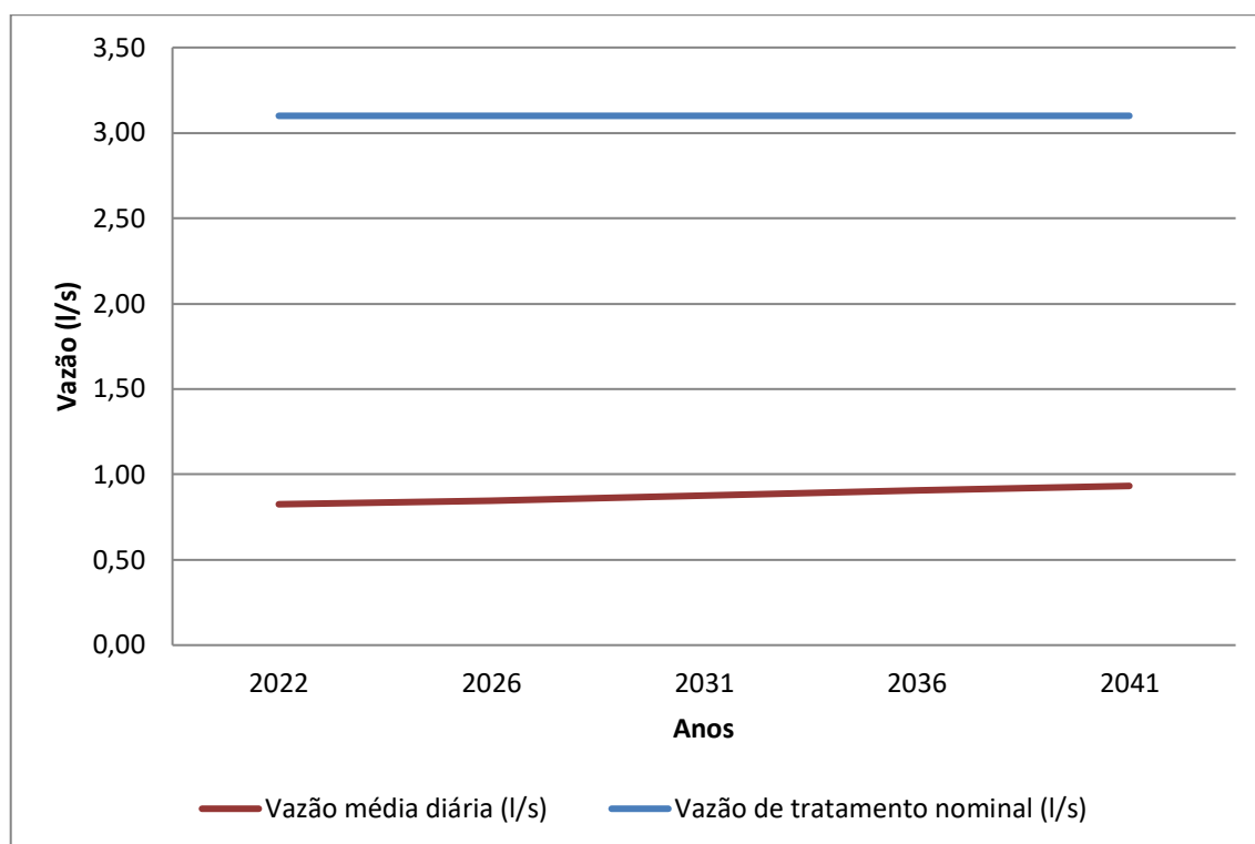
Gráfico 8.16 – Contribuição Média Diária (l/s) x Capacidade nominal da ETE (l/s)
