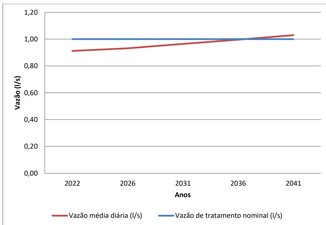
Gráfico 8.24 – Contribuição Média Diária (l/s) x Capacidade nominal da ETE (l/s)
