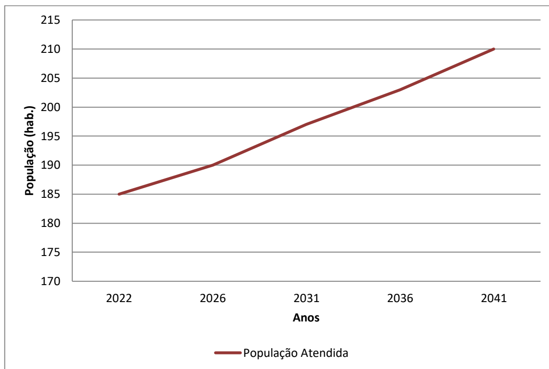
Gráfico 7.14 - População Atendida (hab.) x Anos de Planejamento – Bairro Biguá
