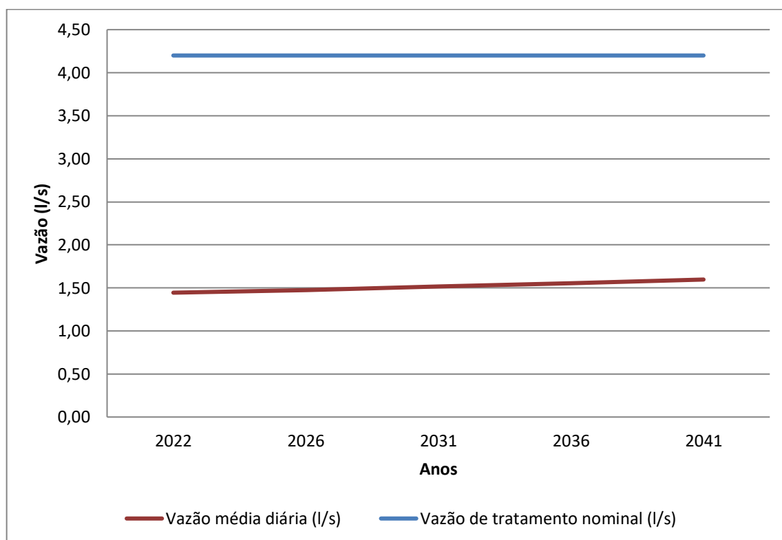
Gráfico 8.14 – Contribuição Média Diária (l/s) x Capacidade nominal da ETE (l/s)
