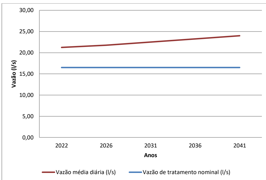
Gráfico 8.10 – Contribuição Média Diária (l/s) x Capacidade Nominal da ETE (l/s)
