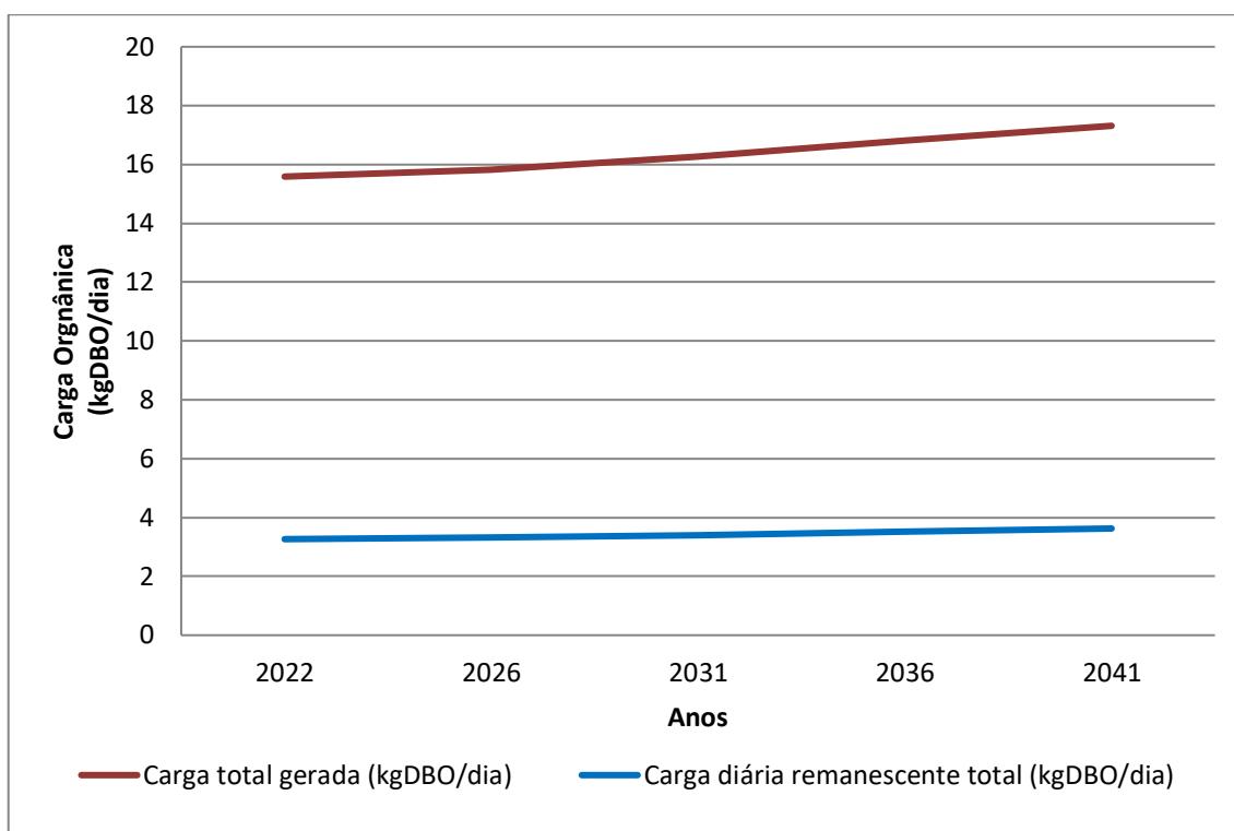
Gráfico 8.21 - Evolução de Cargas Orgânicas (Kg DBO/Dia)
