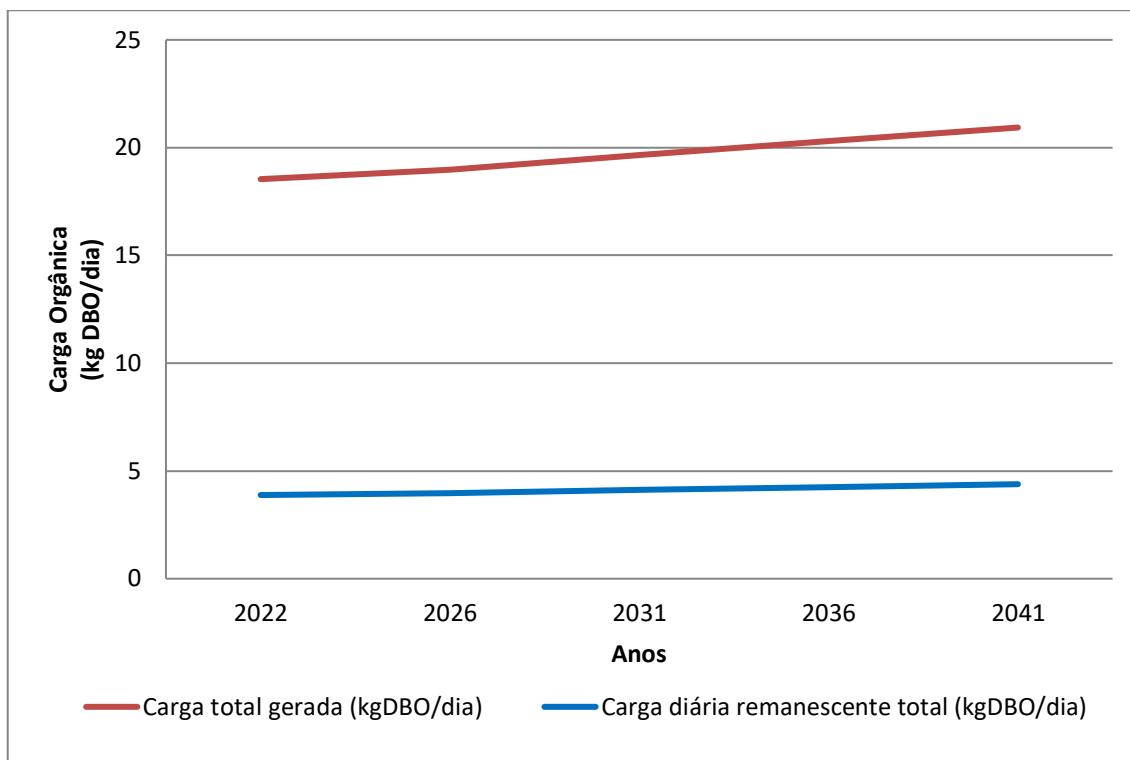
Gráfico 8.17 - Evolução de Cargas Orgânicas (Kg DBO/Dia)
