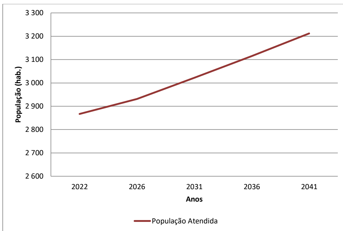
Gráfico 7.3 – População Atendida (hab.) x Anos de Planejamento – Distrito Oliveira Barros e Bairro Biguá
