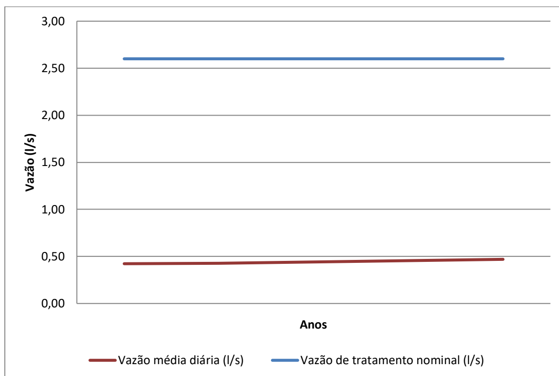
Gráfico 8.20 – Contribuição Média Diária (l/s) x Capacidade nominal da ETE (l/s)
