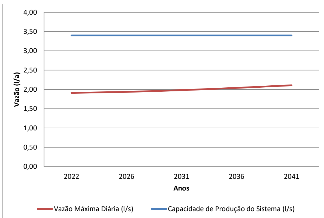
Gráfico 8.7 – Demandas Máximas Diárias (l/s) X Capacidade de Produção do Sistema (l/s)
