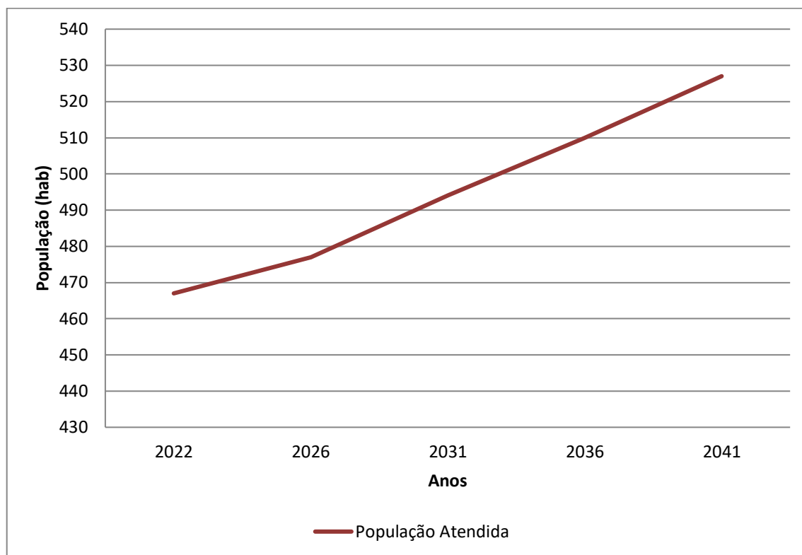
Gráfico 7.15 - População Atendida (hab.) x Anos de Planejamento – Bairro Vila São José
