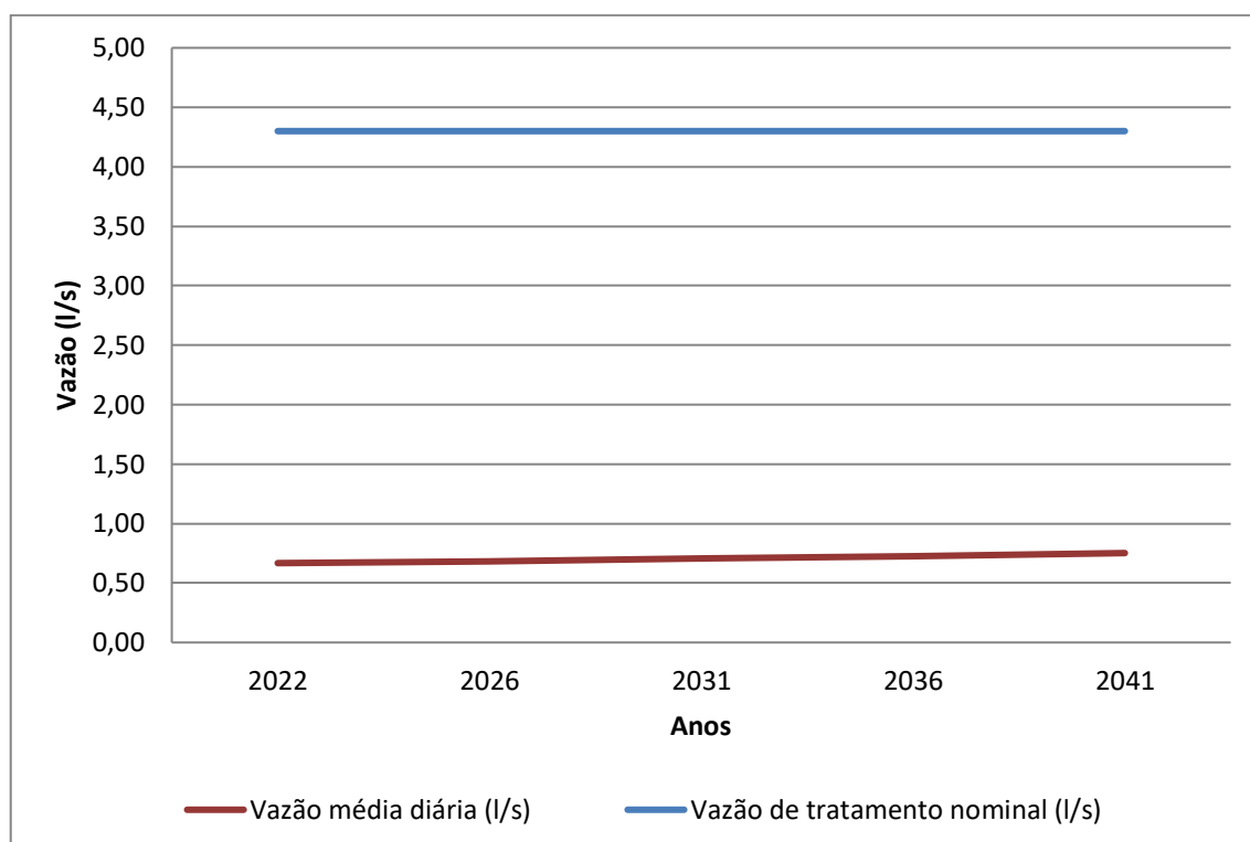
Gráfico 8.22 – Contribuição Média Diária (l/s) x Capacidade nominal da ETE (l/s)
