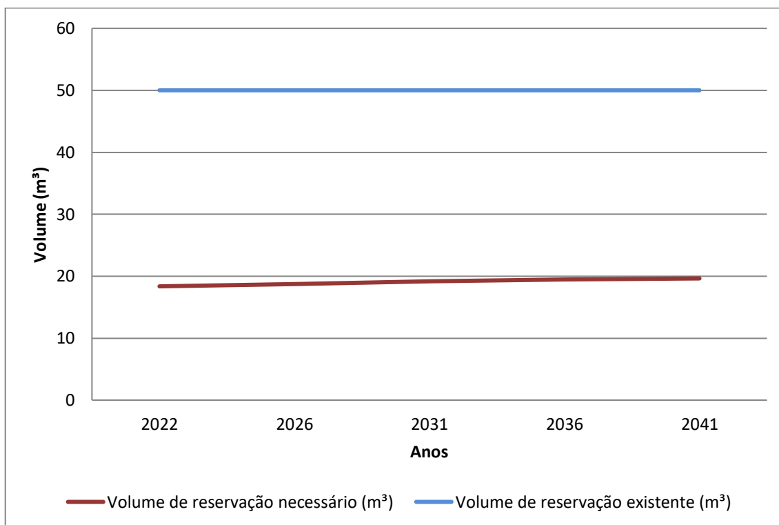
Gráfico 8.9 - Volume de Reservação Necessário (m³) x Volume de Reservação Atual (m³)
