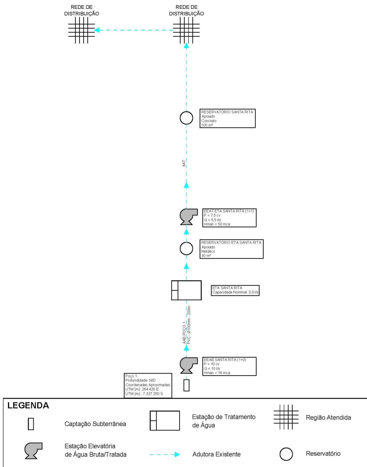
Figura 4.3 – Croqui do Sistema de Abastecimento de Água Existente – Distrito Santa Rita
