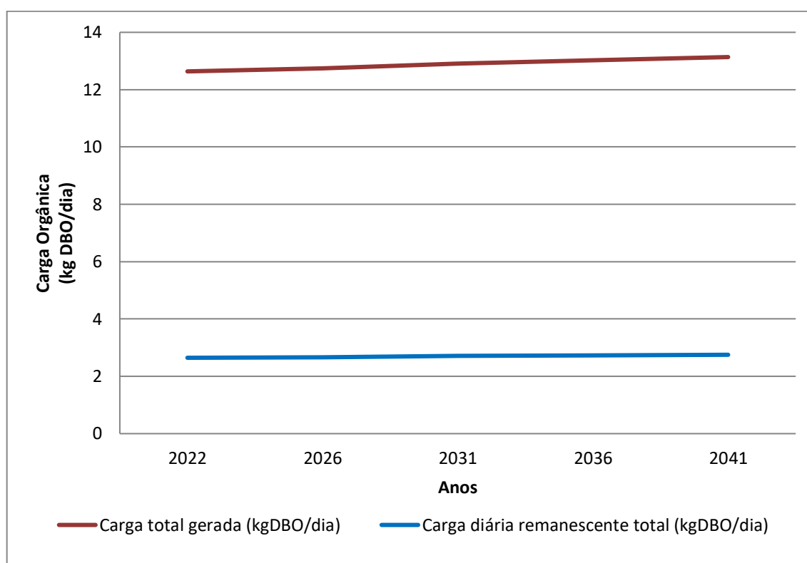
Gráfico 8.19 - Evolução de Cargas Orgânicas (Kg DBO/Dia)
