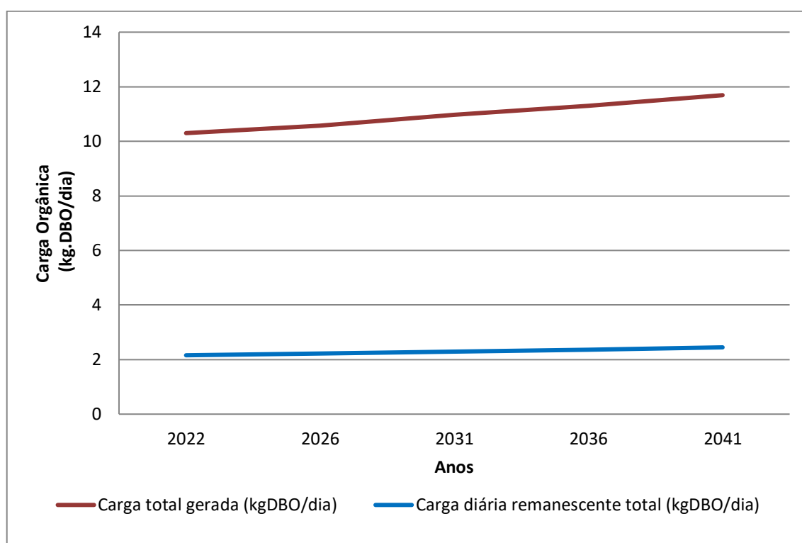
Gráfico 8.23 - Evolução de Cargas Orgânicas (Kg DBO/Dia)
