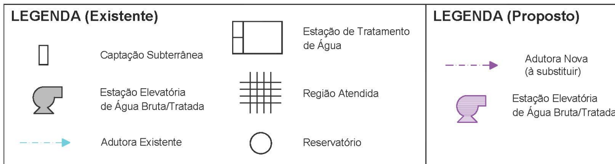
Figura 10.3 – Croqui do Sistema de Abastecimento de Água Proposto para o Sistema Santa Rita
