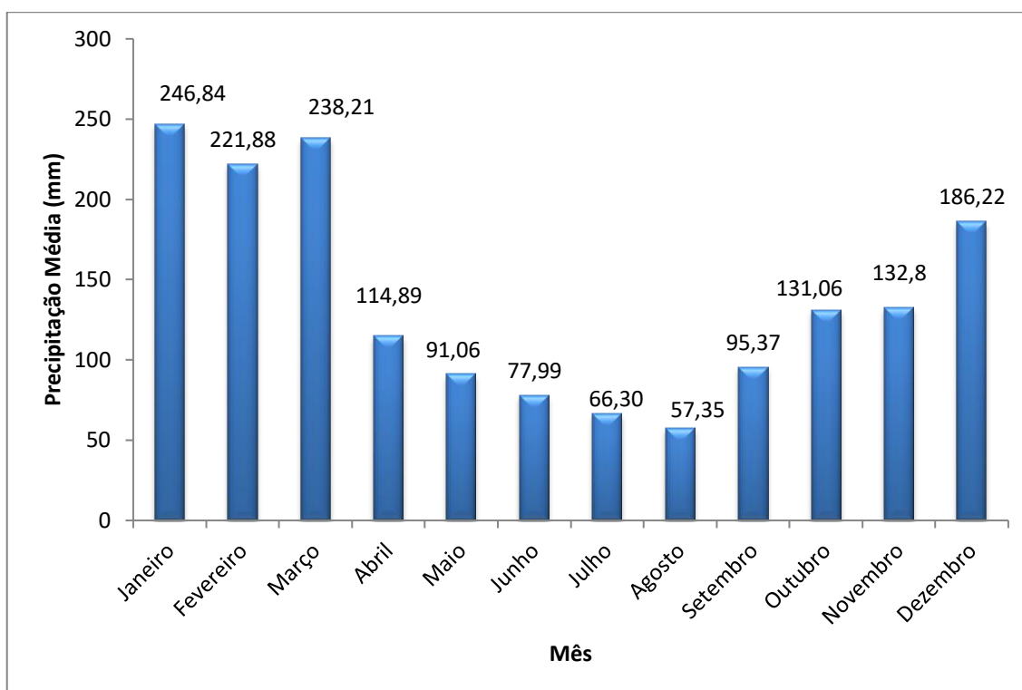
Gráfico 3.1 – Precipitação Média Mensal no Período de 1965 a 2017, Estação F4 012
