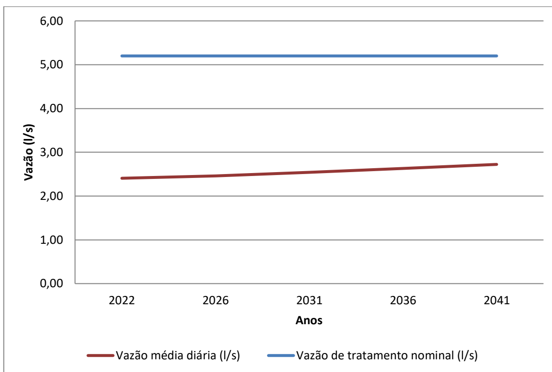
Gráfico 8.12 – Contribuição Média Diária (l/s) x Capacidade nominal da ETE (l/s)
