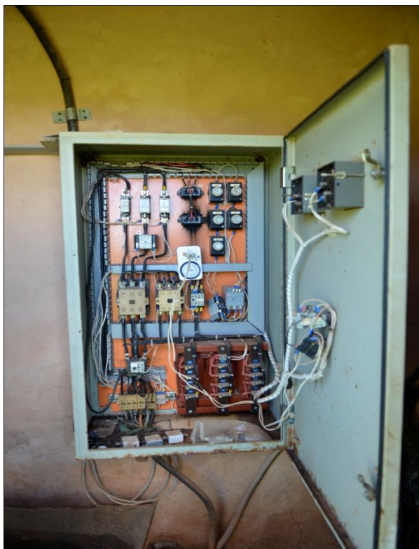
Foto 81: – Painel de Controle de Partida do Poço Profundo - P1 Localização: Jardim Aeroporto.
