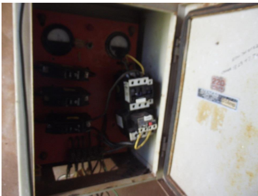
Foto 136: – Painel de Comando – P1 Localização: Bairro Terceira Aliança
