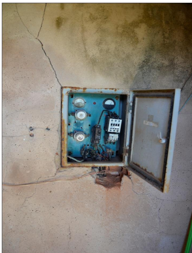
Foto 106: – Painel de Comando do Poço P9 Localização: – Colina Verde
