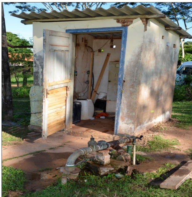
Foto 93: – Poço P5 e ao Fundo Dosadores para o Tratamento Localização: Conj. Habitacional Agostinho Franco
