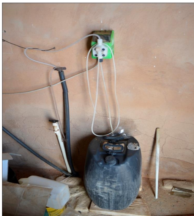
Foto 115: – Produtos Químicos e Bombas Dosadoras – Poço P13
