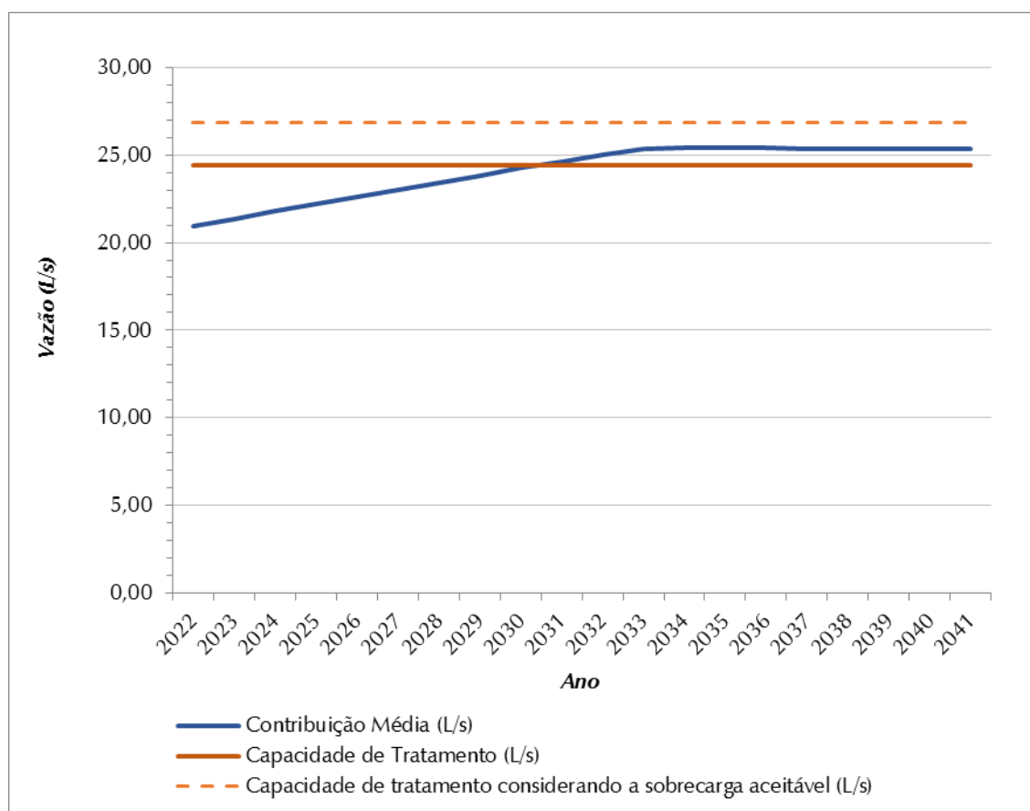
Figura 8.7 – Contribuição Média Total (L/s) x Capacidade de Tratamento de Esgoto (L/s) – SES Sede
