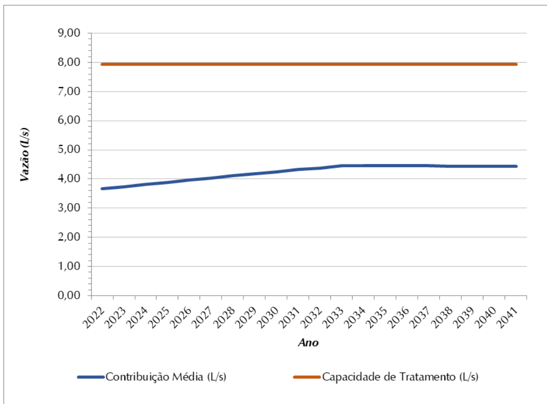
Figura 8.9 – Contribuição Média Total (L/s) x Capacidade de Tratamento de Esgoto (L/s) – SES Costa Machado
