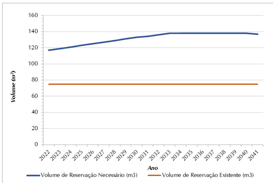
Figura 8.4 - Volume de Reservação Necessário (m³) x Volume de Reservação Atual (m³) SAA Costa Machado
