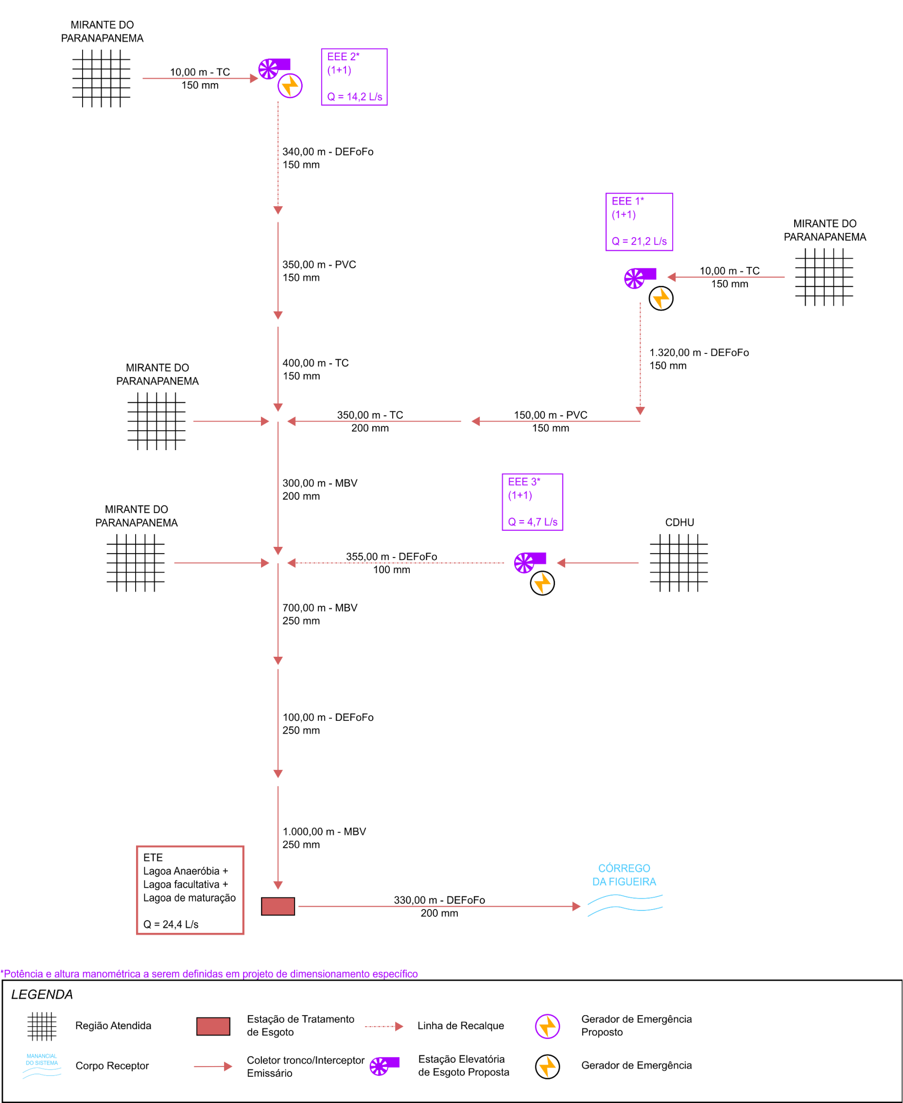
Figura 10.4 – Croqui das intervenções propostas para o sistema de esgotamento sanitário Sede
