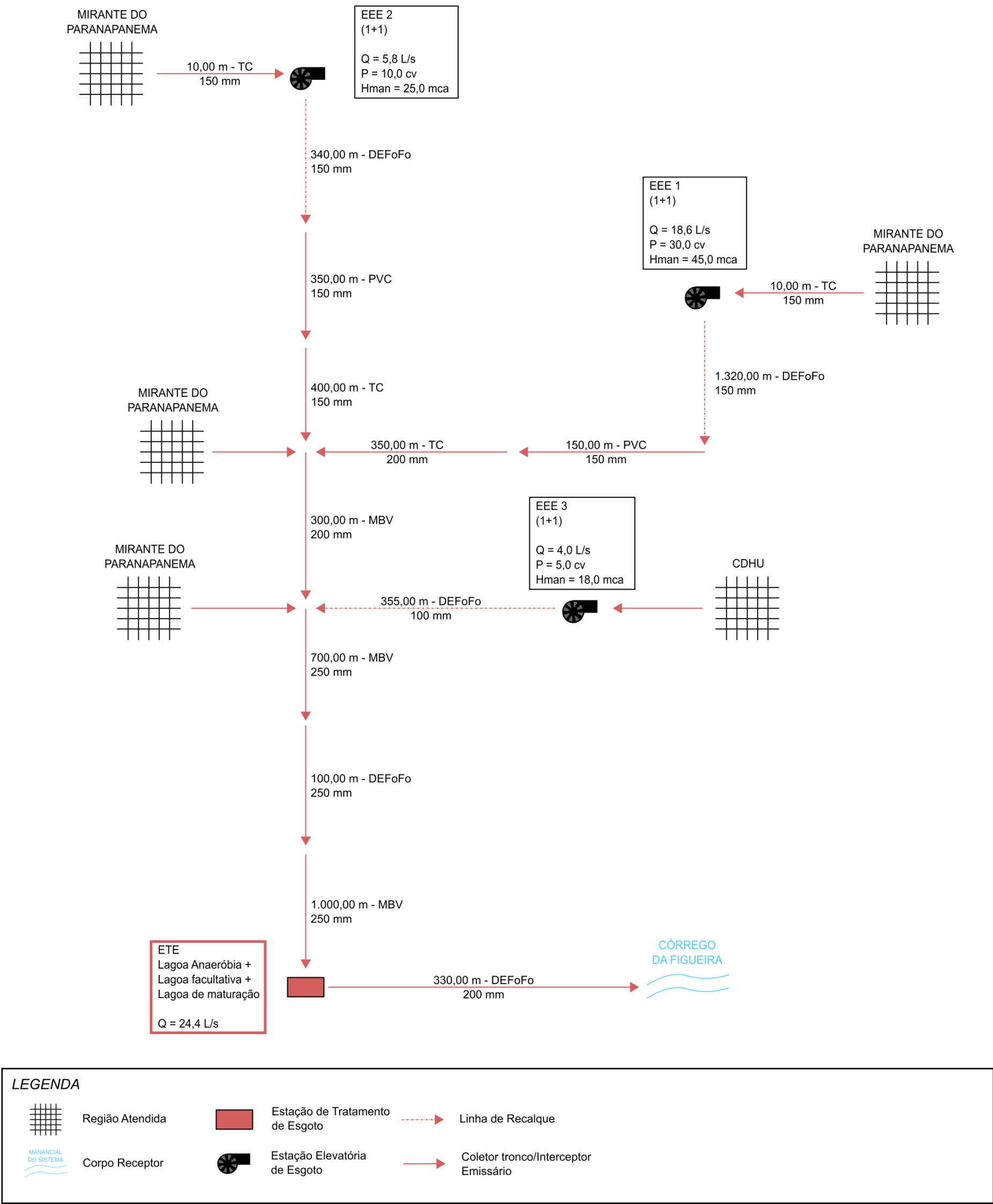
Figura 4.4 – Croqui do Sistema de Esgotamento Sanitário da Sede de Mirante do Paranapanema Fonte: SABESP, 2020.
