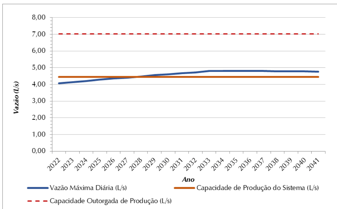
Figura 8.3 – Demandas Máximas Diárias (L/s) X Vazão Captada (L/s) – SAA Costa Machado
