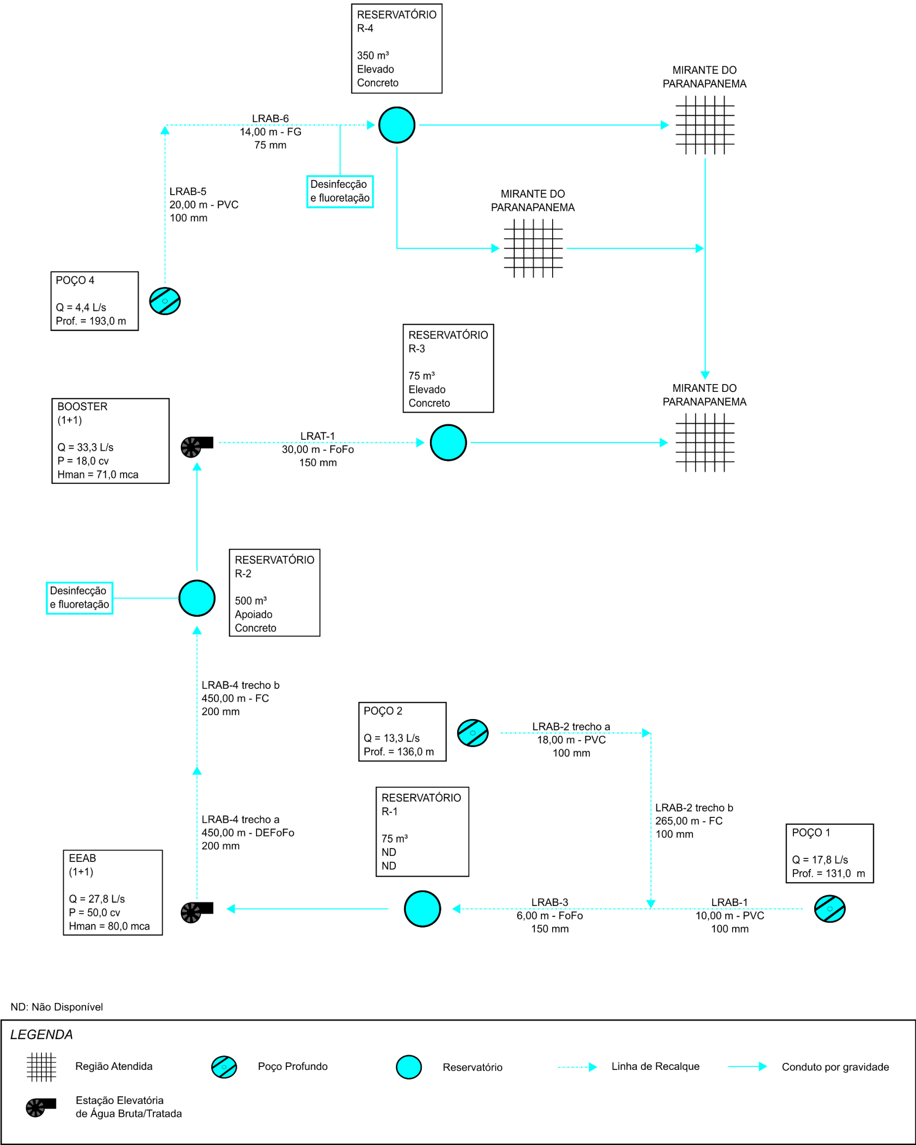
Figura 4.1 – Croqui do Sistema de Abastecimento de Água Sede
