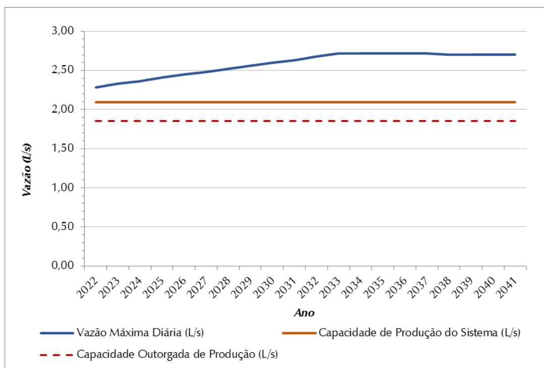
Figura 8.5 – Demandas Máximas Diárias (L/s) X Vazão Captada (L/s) – SAA Cuiabá Paulista
