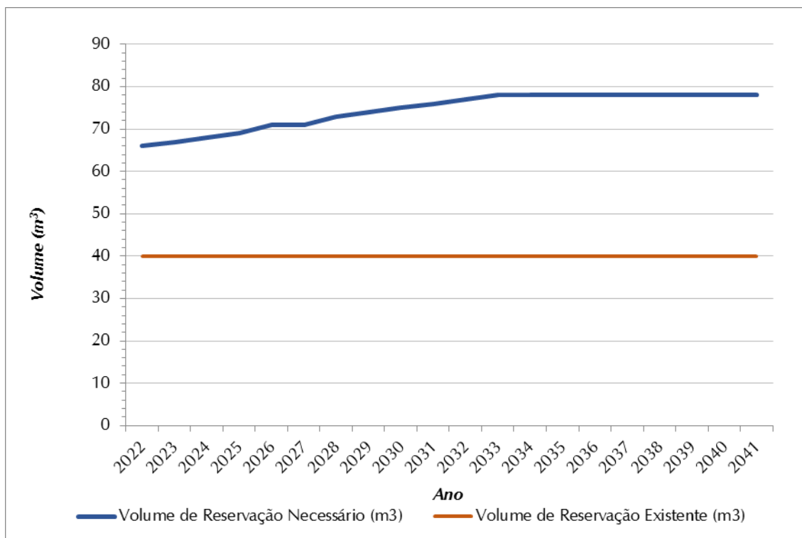
Figura 8.6 - Volume de Reservação Necessário (m³) x Volume de Reservação Atual (m³) SAA Cuiabá Paulista
