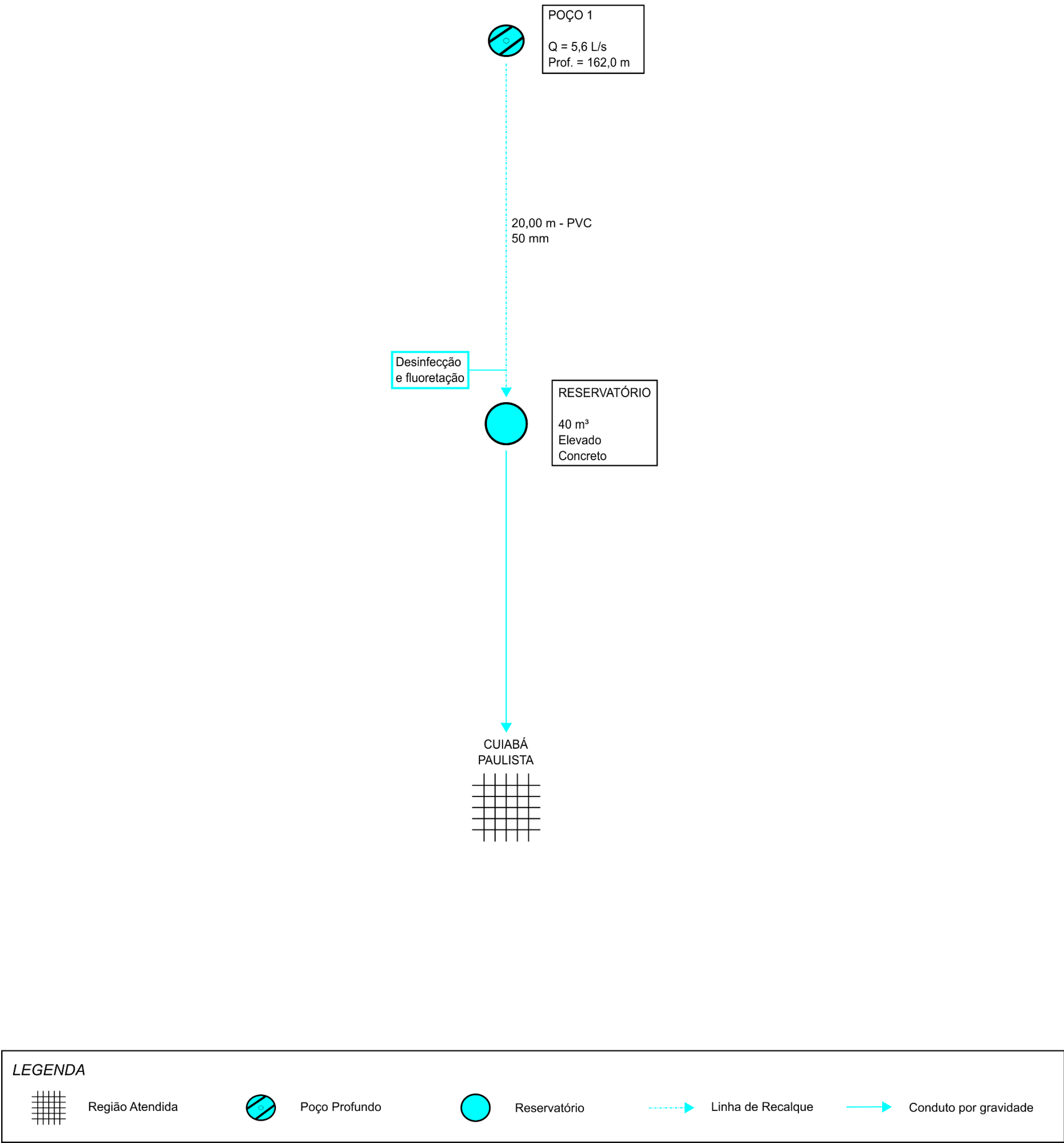
Figura 4.3 – Croqui do Sistema de Abastecimento de Água Cuiabá Paulista
