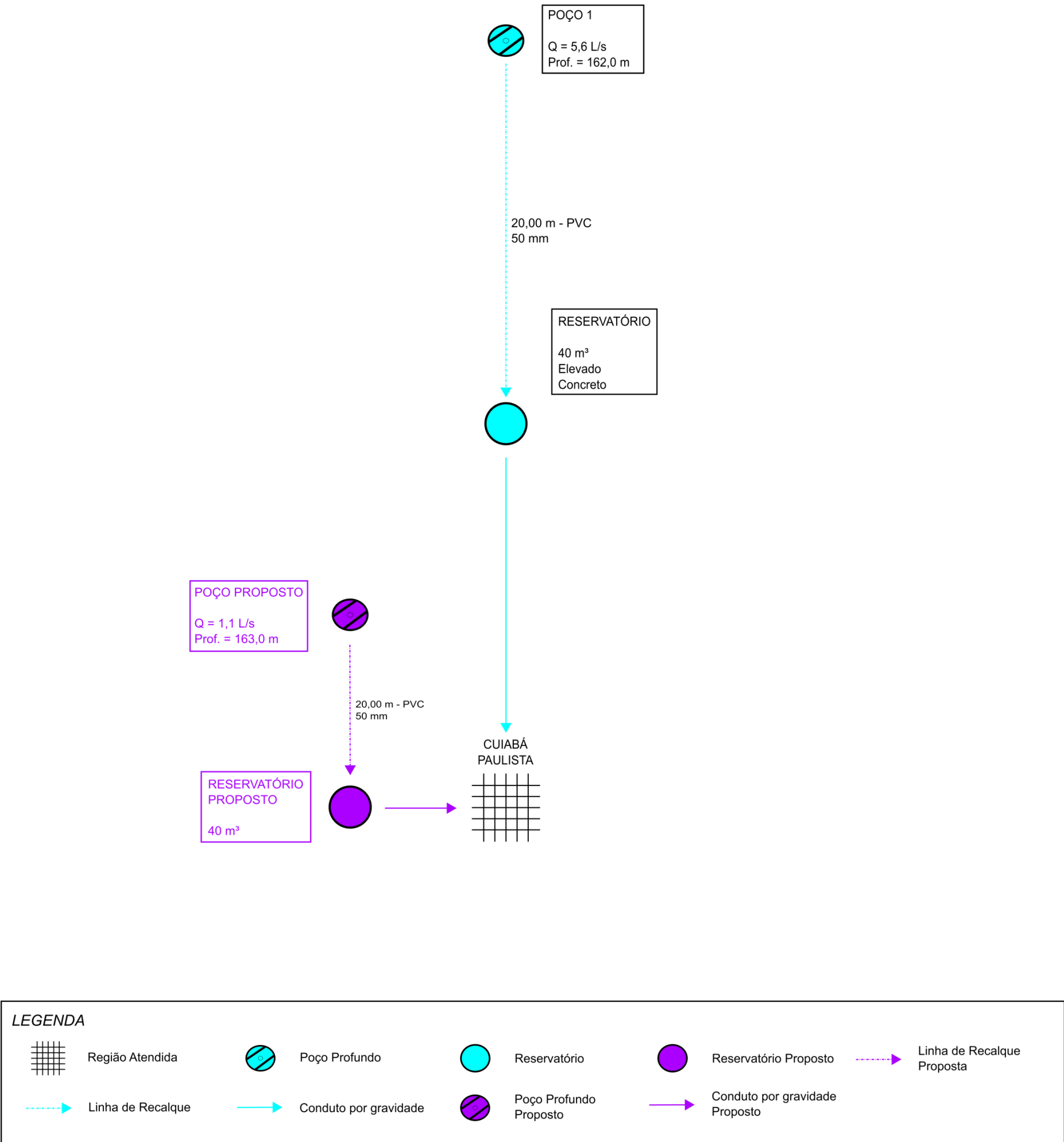
Figura 10.3 – Croqui das intervenções propostas para o sistema de abastecimento de água Cuiabá Paulista
