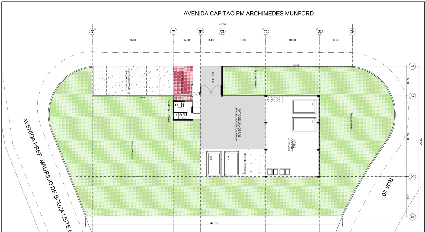
Figura 4 Lay out ECOPONTO Parque Olimpico
