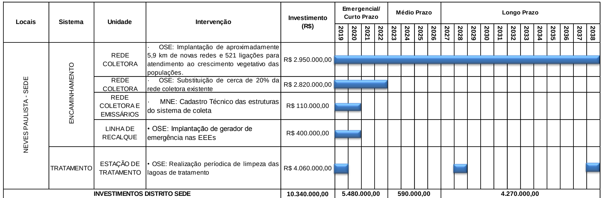
Figura 10.4 - Cronograma de Implantação das Intervenções Propostas no Sistema de Esgotos Sanitários - Sede
