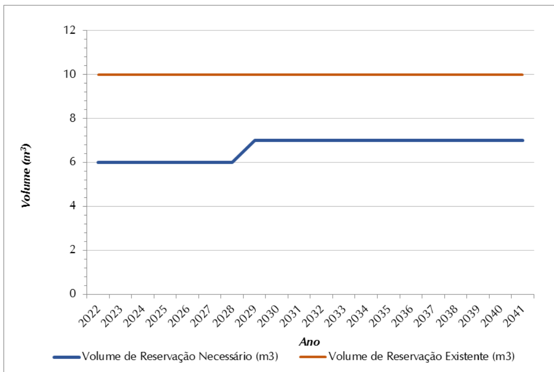
Figura 8.4 - Volume de Reservação Necessário (m³) x Volume de Reservação Atual (m³) SAA Nova Brasília
