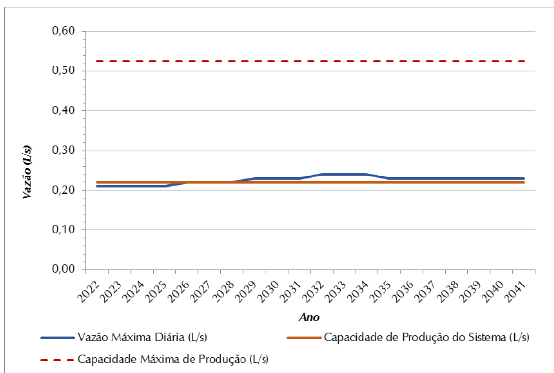
Figura 8.3 – Demandas Máximas Diárias (L/s) X Vazão Captada (L/s) – SAA Nova Brasília
