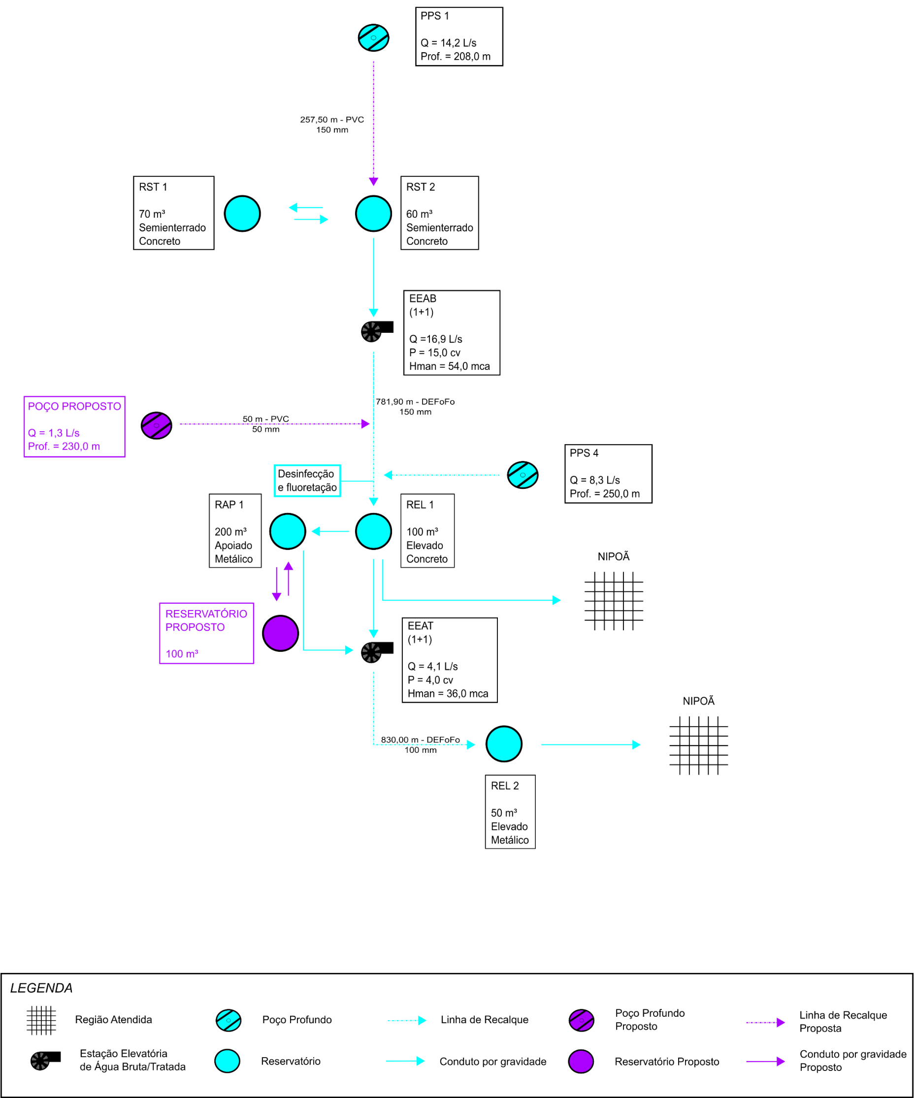
Figura 10.1 – Croqui das intervenções propostas para o sistema de abastecimento de água Sede
