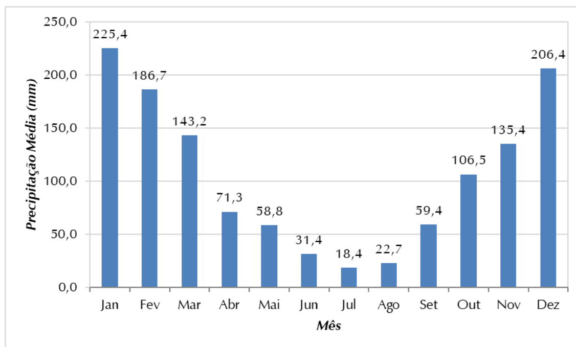
Figura 3.2 - Precipitação Média Mensal no Período de 1959 a 2021, Estação B6-034
