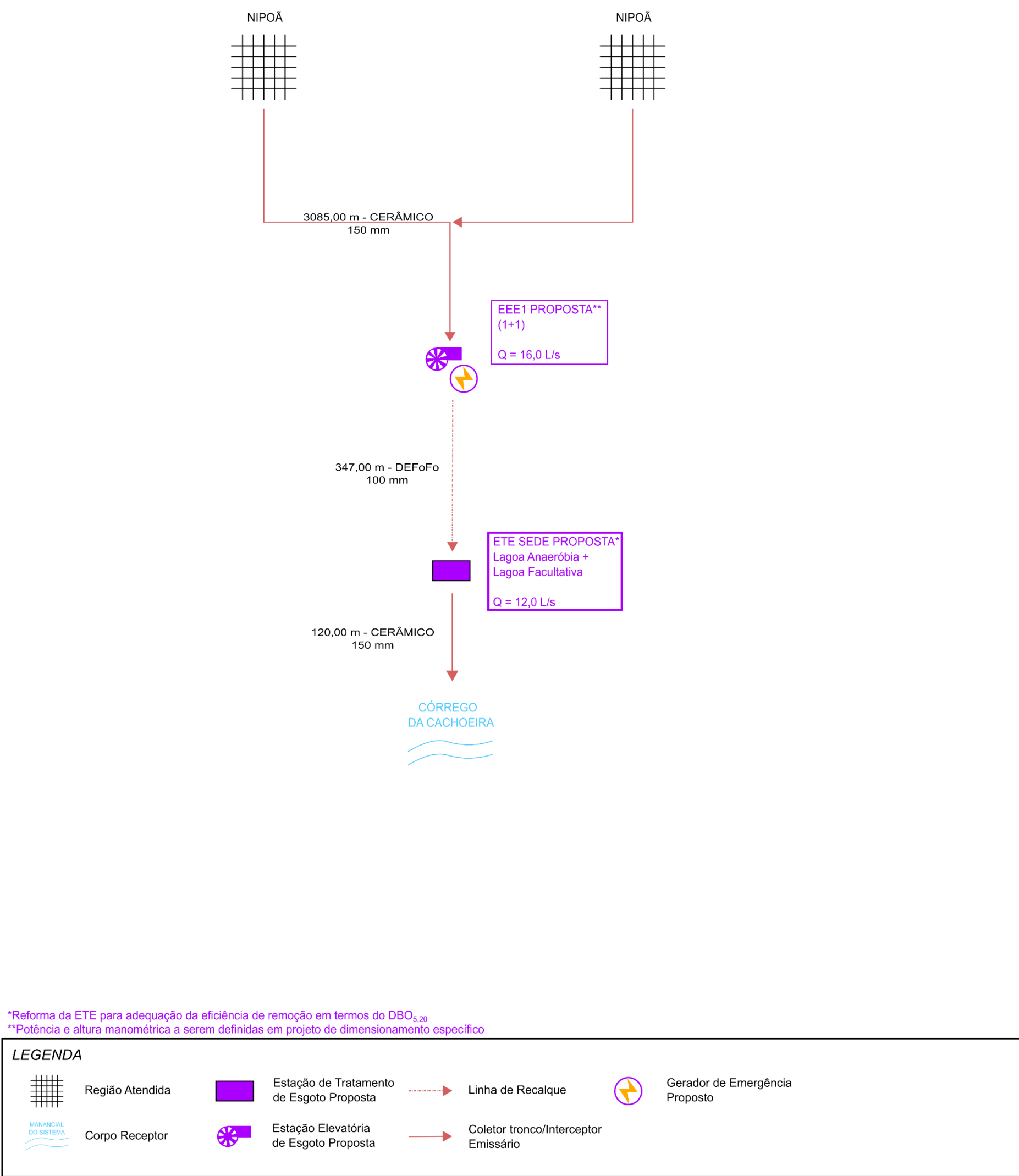
Figura 10.2 – Croqui das intervenções propostas para o sistema de esgotamento sanitário Sede
