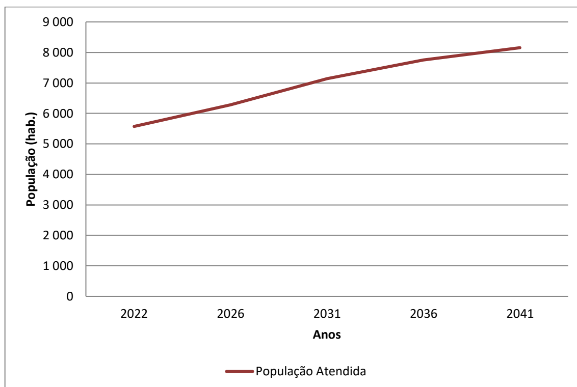
Gráfico 7.6 - População Atendida (hab.) x Anos de Planejamento – Sede Urbana
