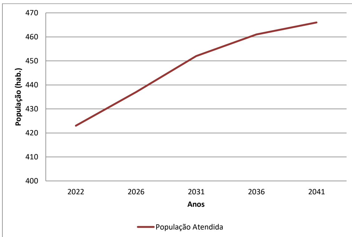
Gráfico 7.4 – População Atendida (hab.) x Anos de Planejamento – Distritos Ingás e Mangaratu
