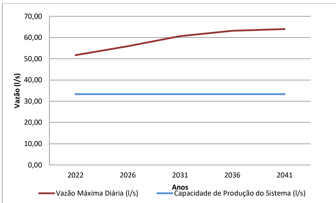
Gráfico 8.1 – Demandas Máximas Diárias (l/s) X Capacidade de Produção do Sistema (l/s)
