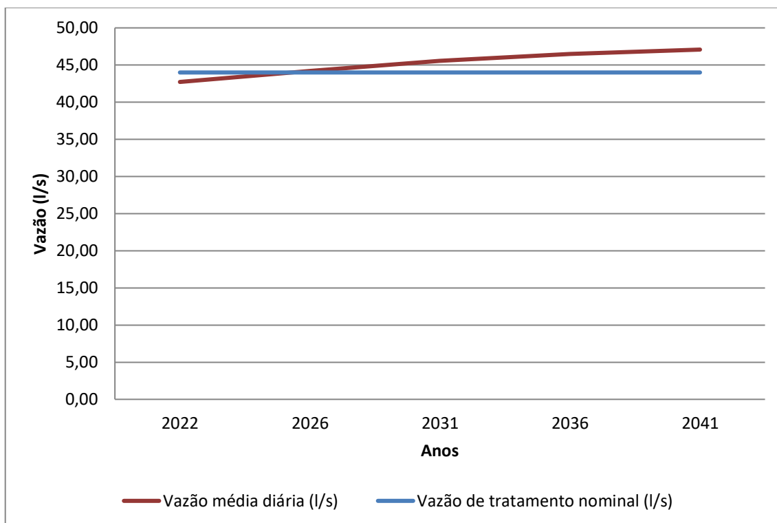
Gráfico 8.5 – Vazão Média Diária (l/s) x Vazão de Tratamento Nominal da ETE (l/s)
