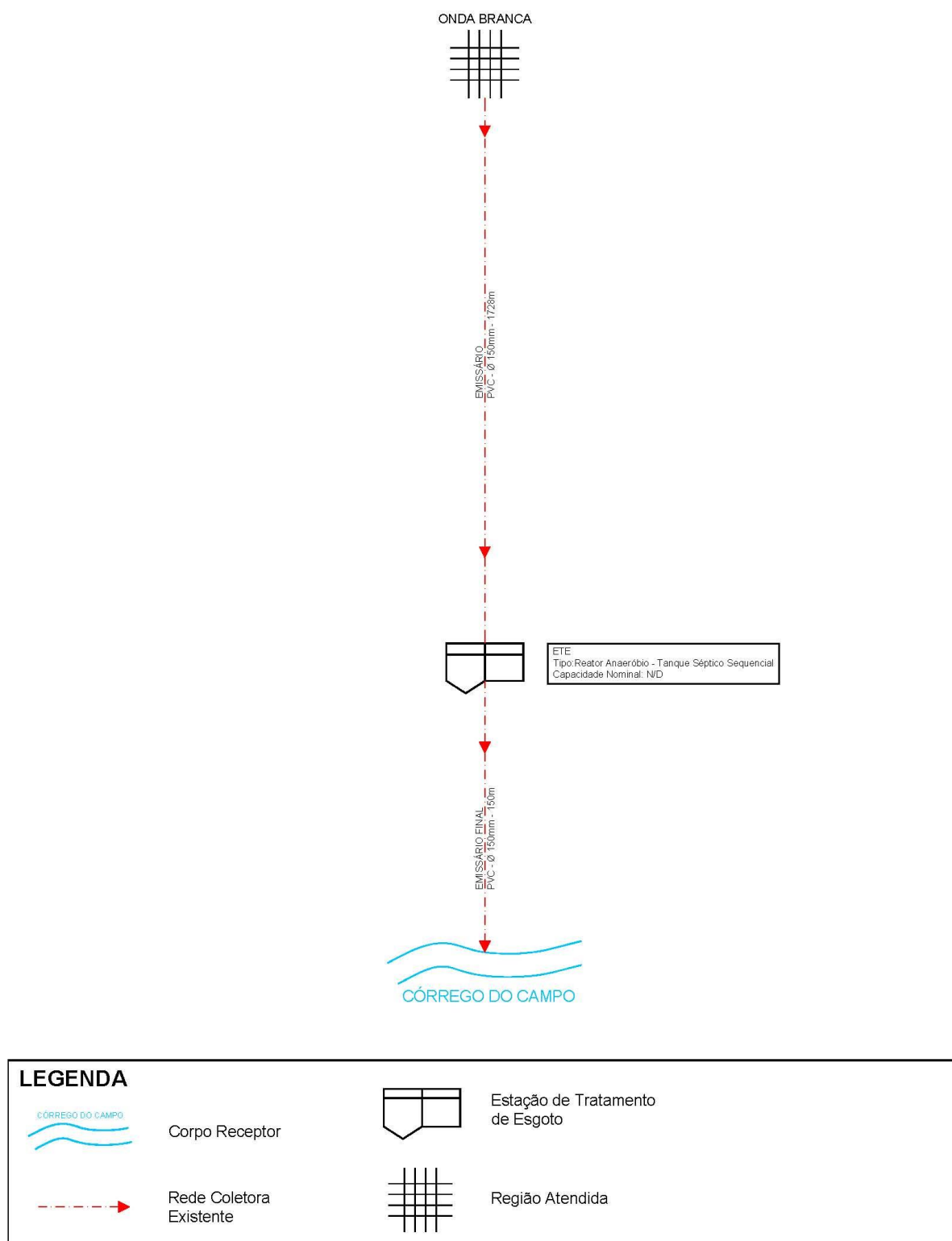
Figura 4.5 – Croqui do Sistema de Esgotamento Sanitário Existente – Distrito Onda Branca
