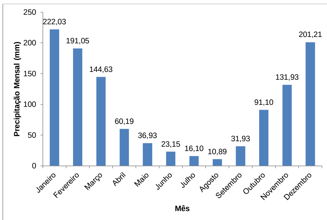
Gráfico 3.1 – Precipitação Média Mensal no Período de 1943 a 1966, Estação B6-024
