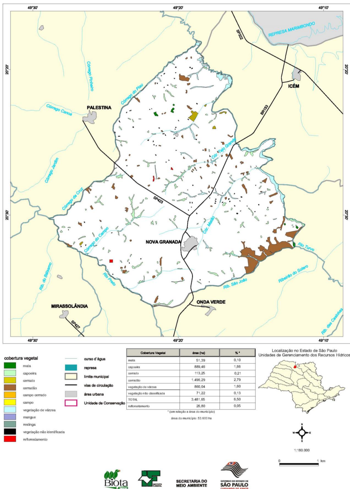
Figura 3.2 – Cobertura Vegetal no Município de Nova Granada
