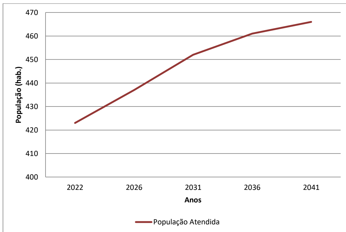
Gráfico 7.7 - População Atendida (hab.) x Anos de Planejamento – Distritos Ingás e Mangaratu
