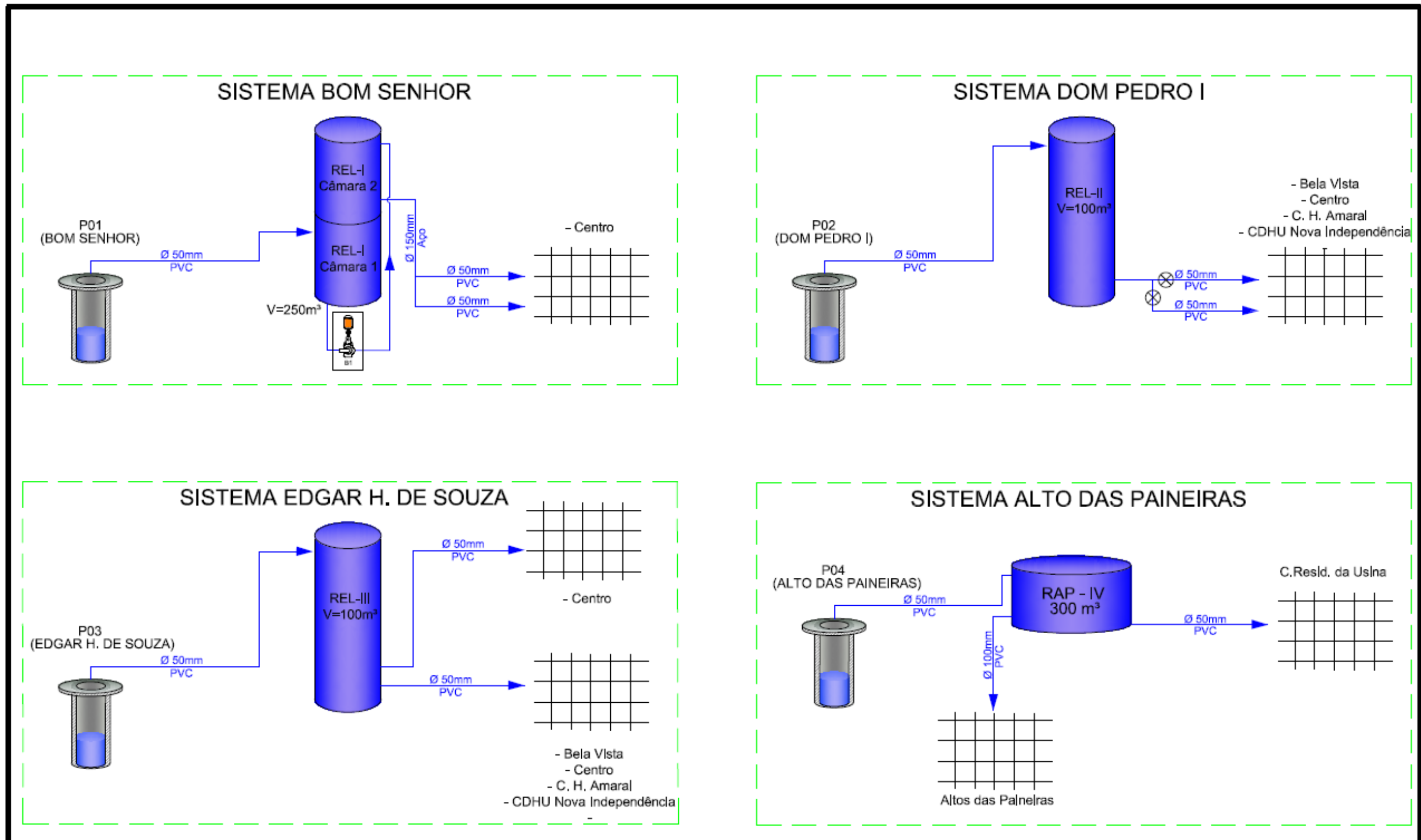
Ilustração 3.1 - Desenho do Sistema de Abastecimento de Água
