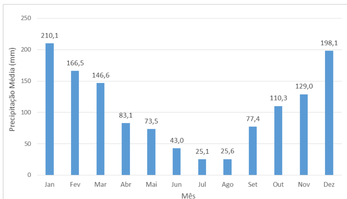
Gráfico 2.1 - Precipitação Média Mensal no Período de 1970 a 2000, Estação C8-045
