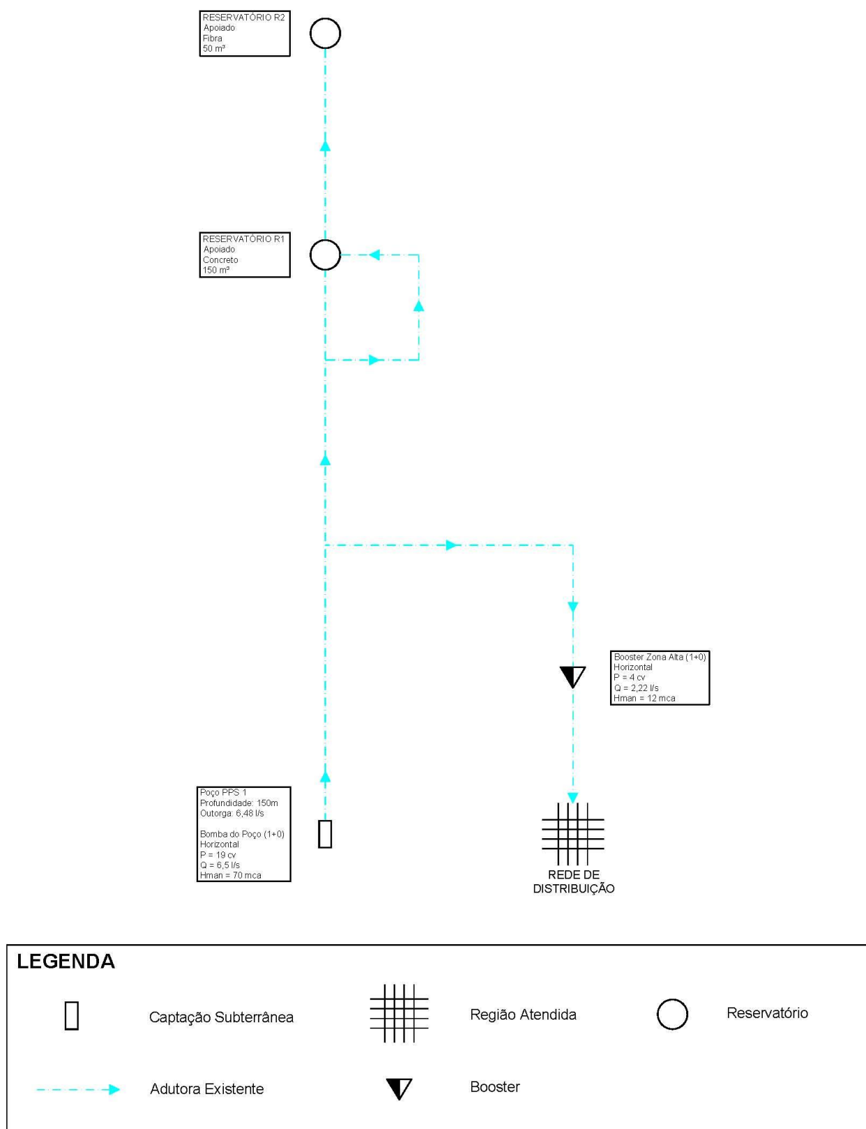
Figura 4.1 – Croqui do Sistema de Abastecimento de Água Existente – Sede Urbana.
