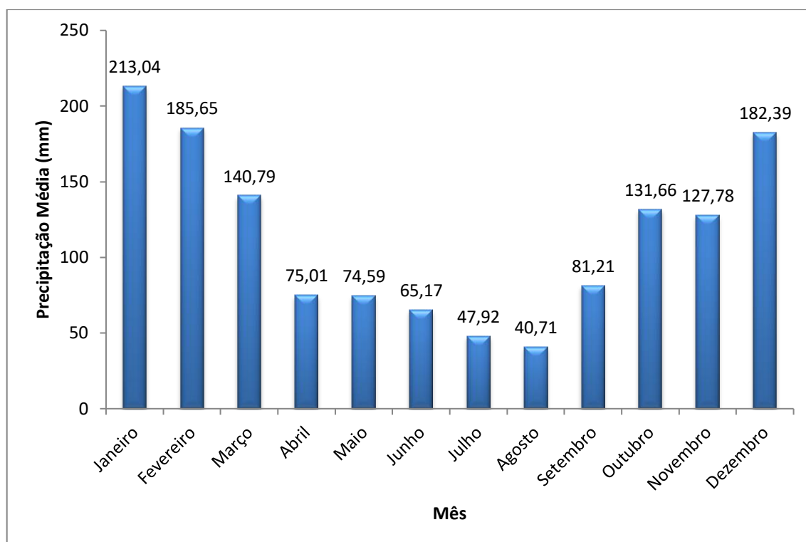
Gráfico 3.1 – Precipitação Média Mensal no Período de 1944 a 2021, Estação D6-003
