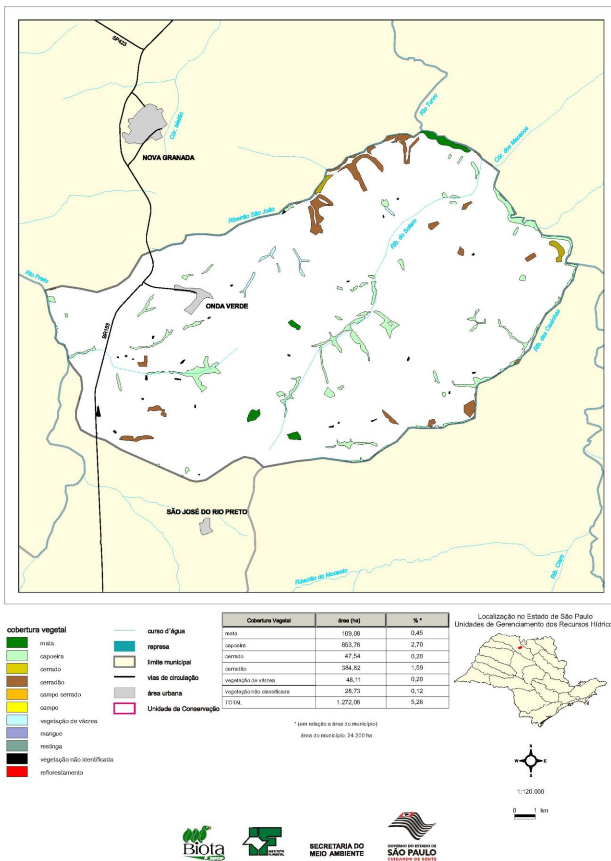
Figura 3.2 – Cobertura Vegetal no Município de Onda Verde
