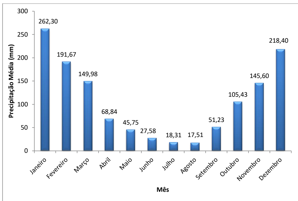
Gráfico 3.1 – Precipitação Média Mensal no Período de 1943 a 2021, Estação B6-026
