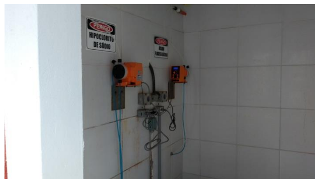
Foto 3.9 – Sistema de desinfecção simples
