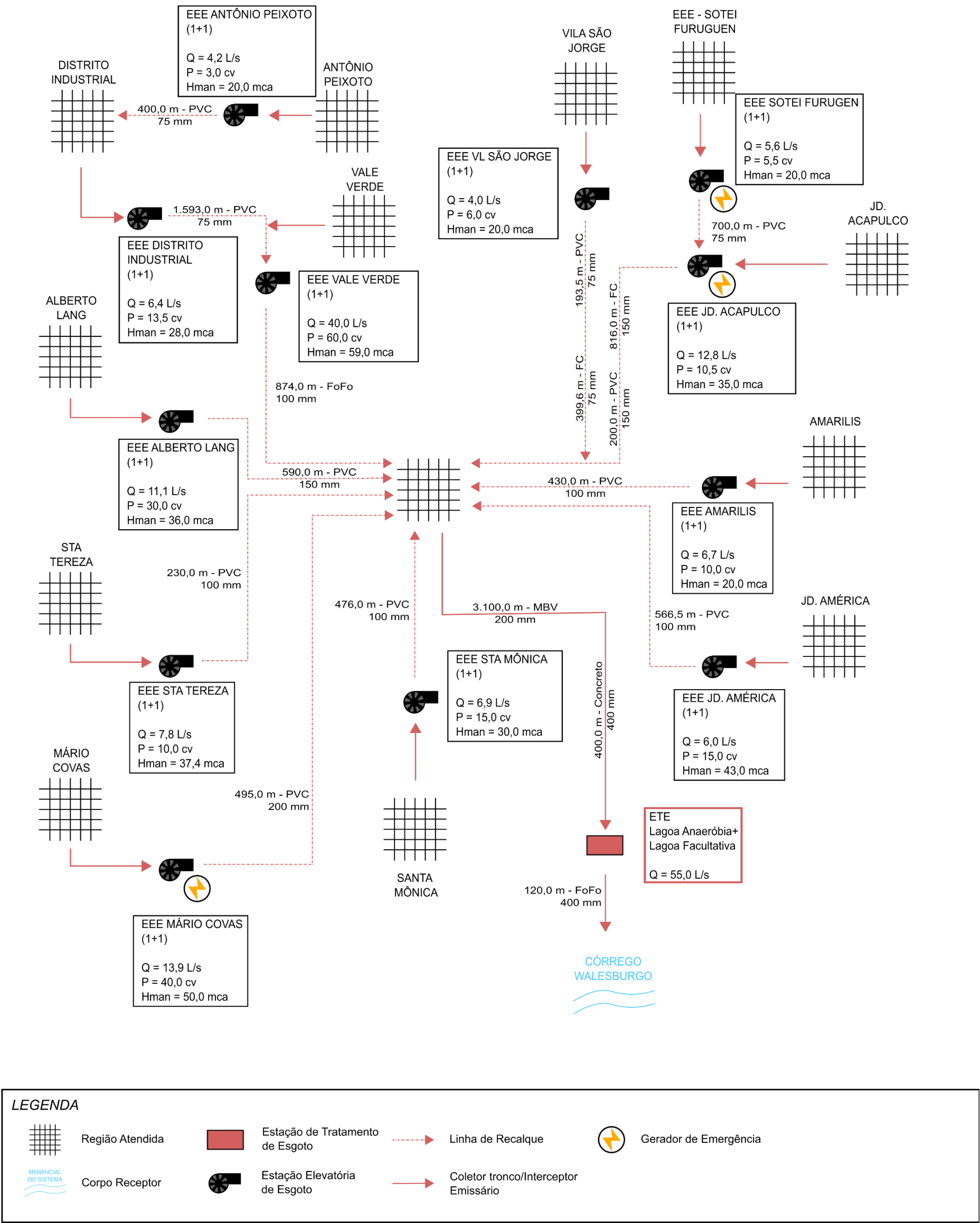
Figura 4.3 – Croqui do Sistema de Esgotamento Sanitário da Sede de Osvaldo Cruz
