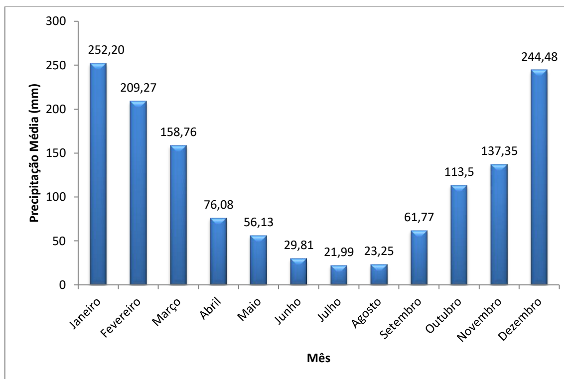
Gráfico 3.1 – Precipitação Média Mensal no Período de 1965 a 1999, Estação C5-089
