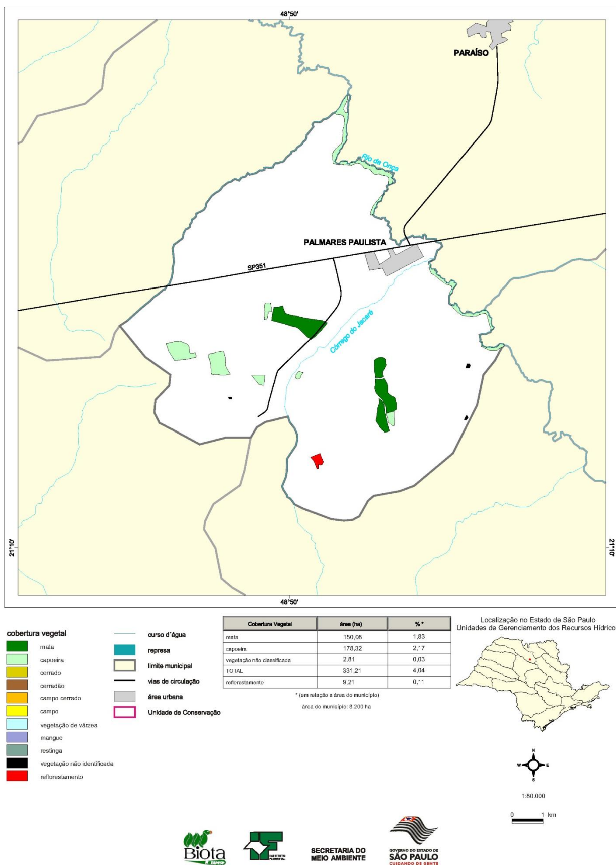
Figura 3.2 – Cobertura Vegetal no Município de Palmas Paulista
