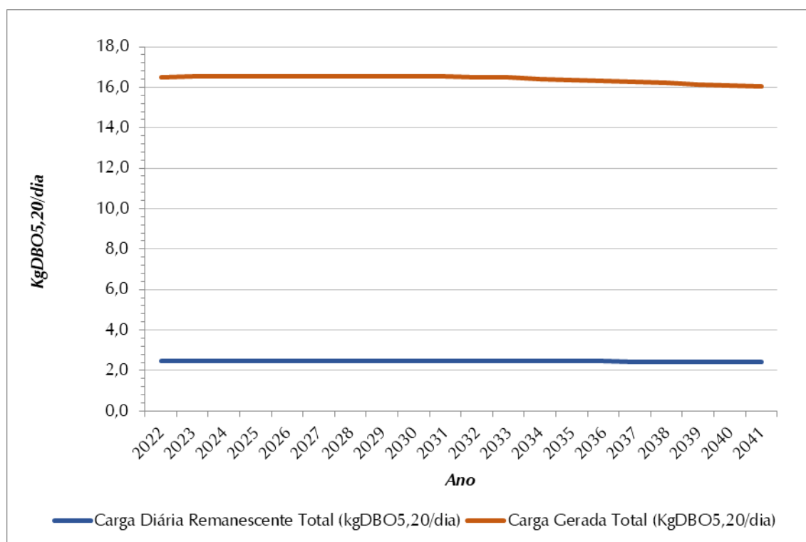
Figura 8.8 - Evolução de Cargas Orgânicas (Kg DBO 5,20 /Dia) – SES Dalas
