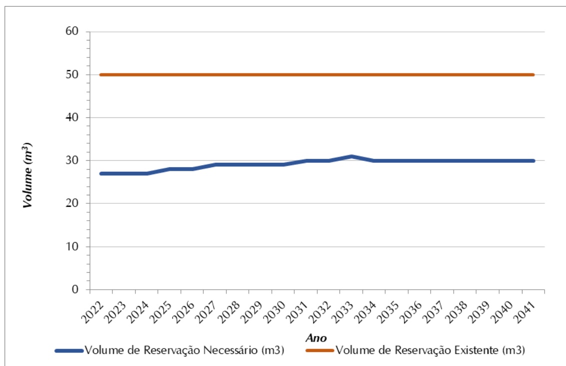
Figura 8.4 - Volume de Reservação Necessário (m³) x Volume de Reservação Atual (m³) – SAA Dalas
