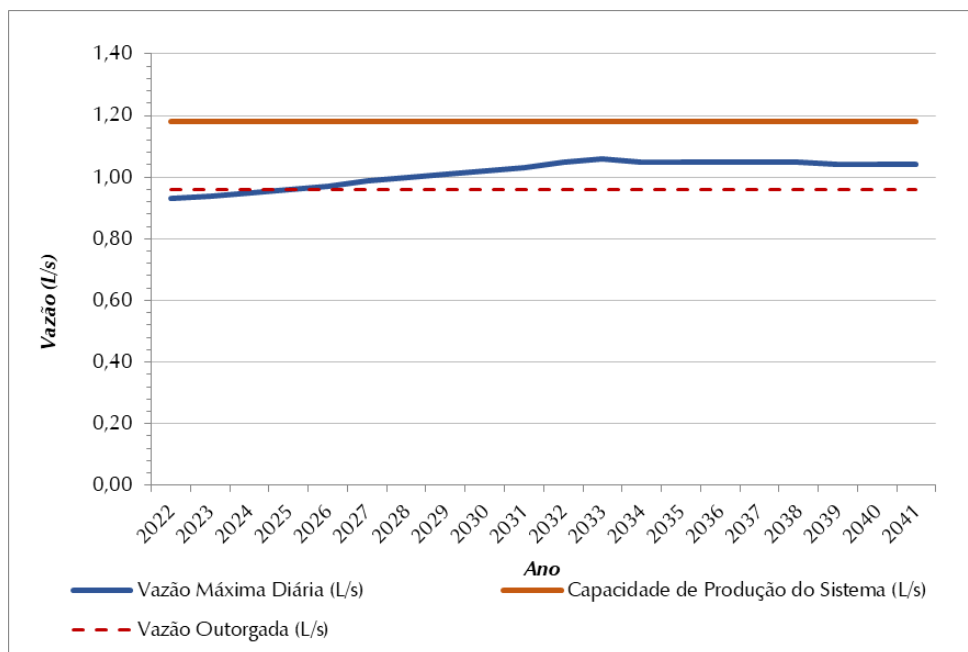
Figura 8.3 – Demandas Máximas Diárias (L/s) X Vazão Captada (L/s) – SAA Dalas
