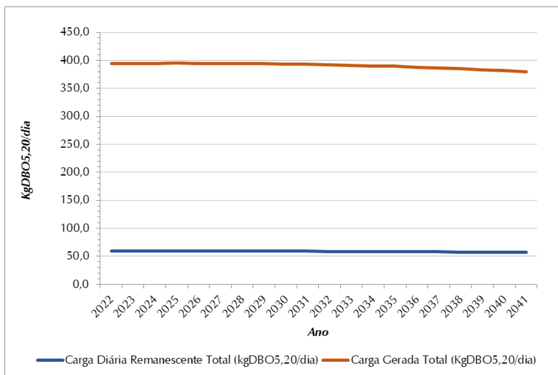
Figura 8.6 - Evolução de Cargas Orgânicas (Kg DBO 5,20 /Dia) – SES Sede
