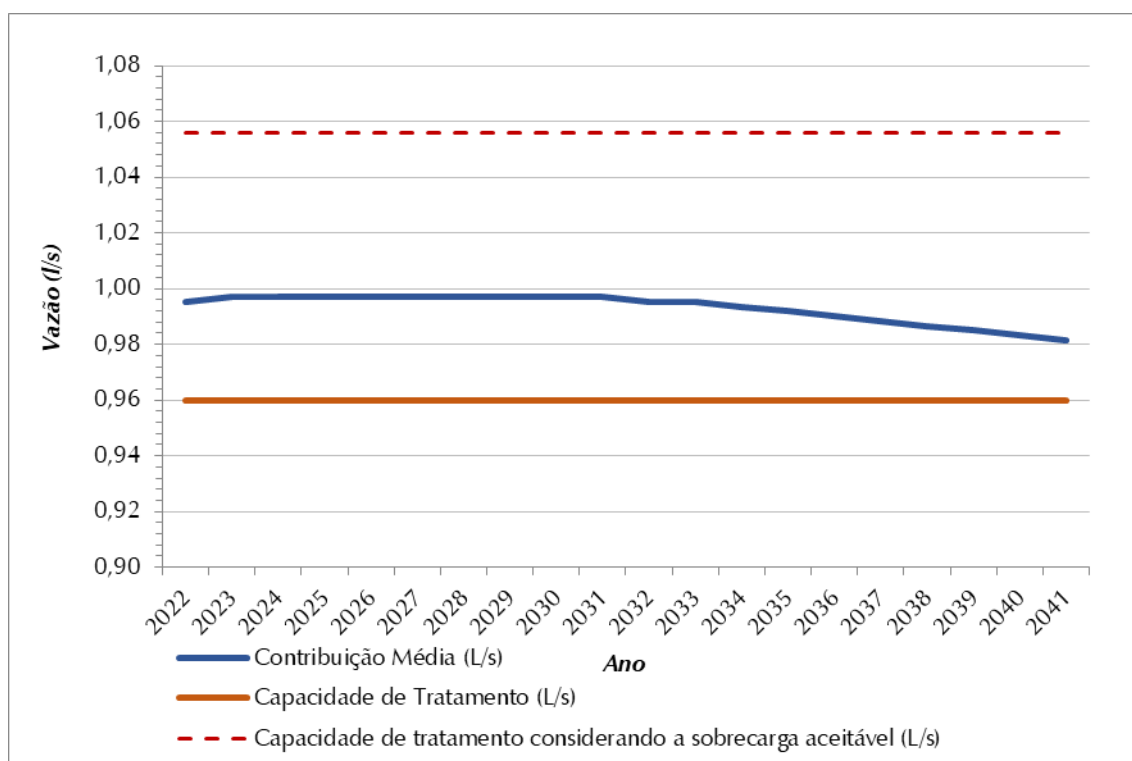
Figura 8.7 – Contribuição Média Total (L/s) x Capacidade de Tratamento de Esgoto (L/s) – SES Dalas
