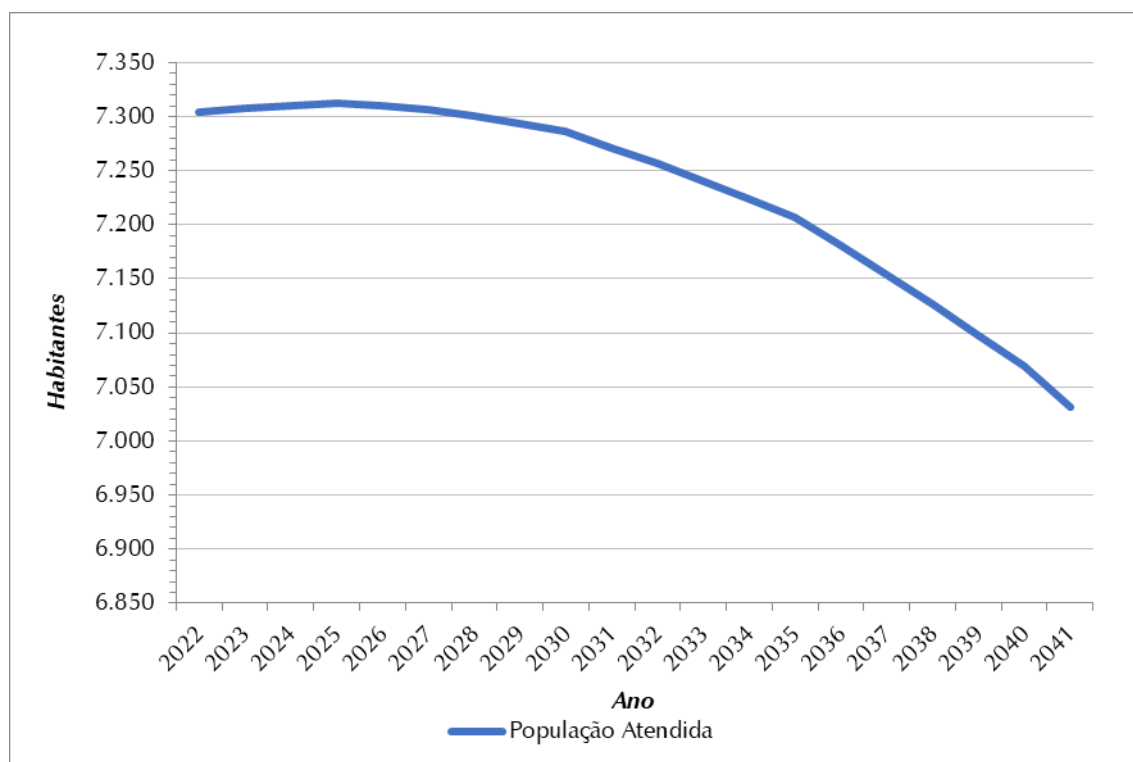
Figura 7.4 - Evolução da População Atendida (hab.) – SES Sede
