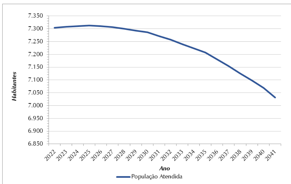
Figura 7.2 – Evolução da População Atendida (hab.) – SAA Sede
