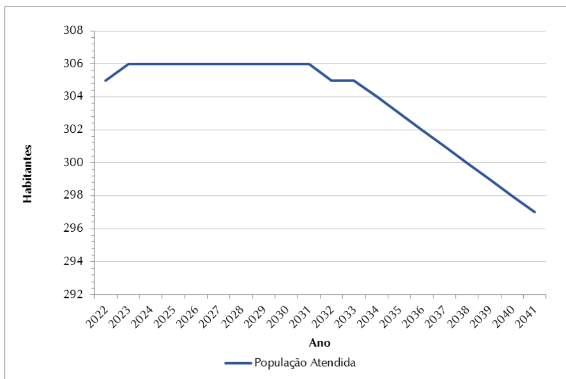
Figura 7.3 – Evolução da População Atendida (hab.) – SAA Dalas
