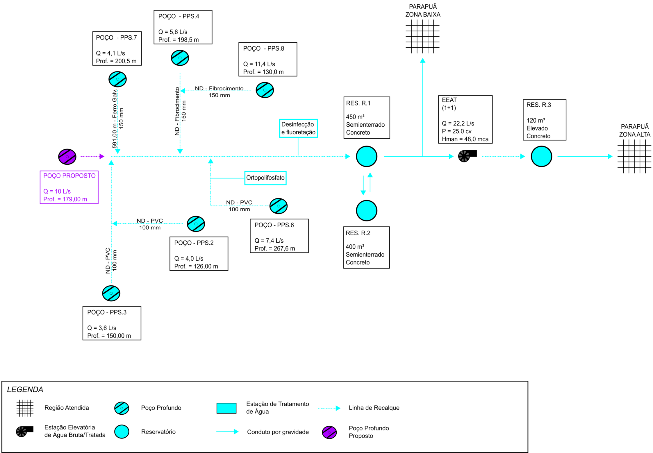
Figura 10.1 – Croqui das Intervenções Propostas para o Sistema de Abastecimento de Água Sede
