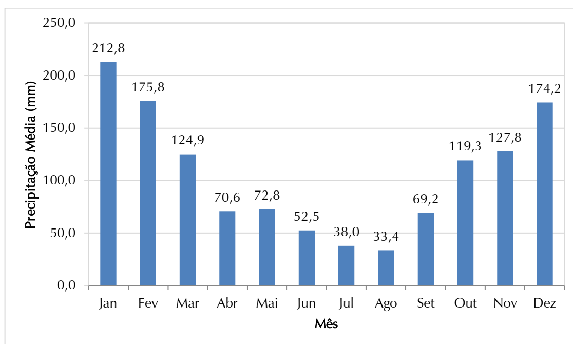
Figura 3.2 - Precipitação Média Mensal no Período de 1944 a 2021, Estação C7-001
