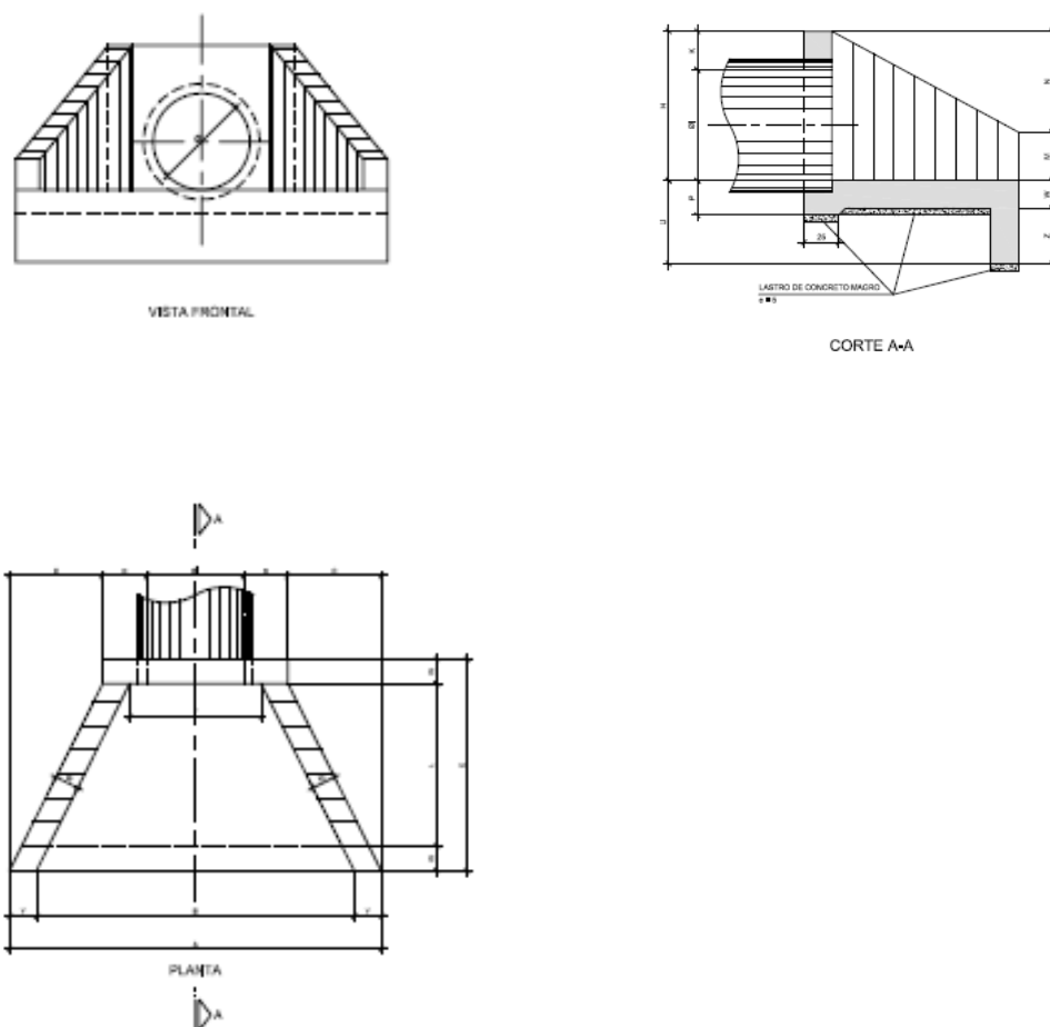
Ilustração 8.5 – Canal em gabião
