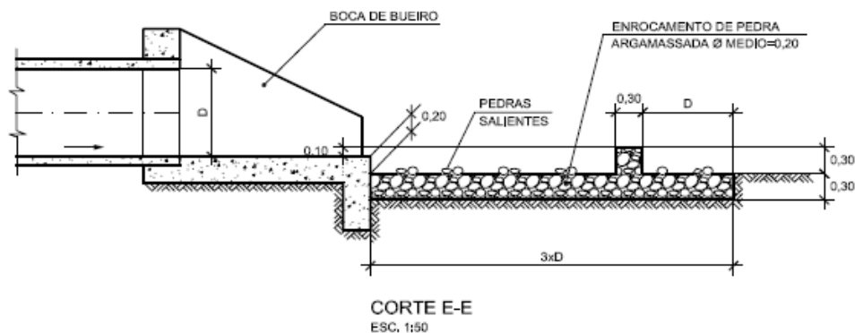
Ilustração 8.10 – Ala da saída com dissipador
