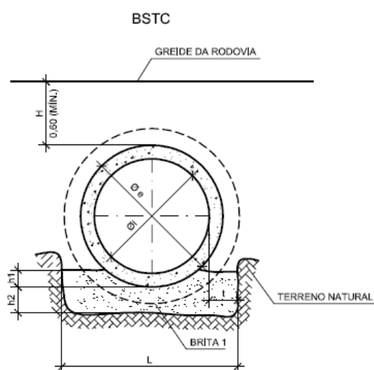
Ilustração 8.4 – Assentamento de tubos de concreto
