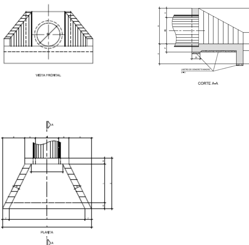
Ilustração 8.9 – Ala da saída com dissipador
