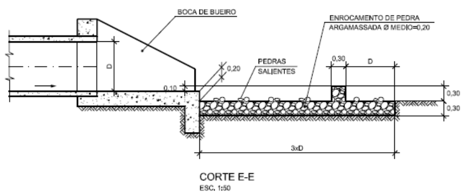
Ilustração 8.6 – Ala da saída com dissipador
