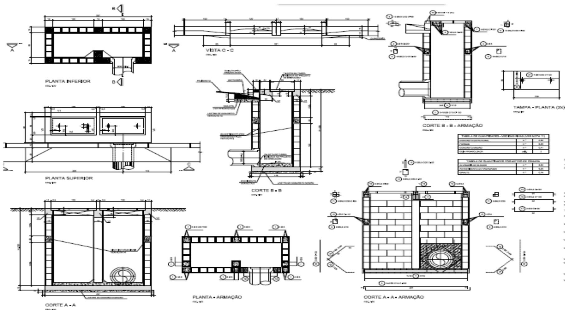
Ilustração 8.2 – Boca de Lobo Dupla
