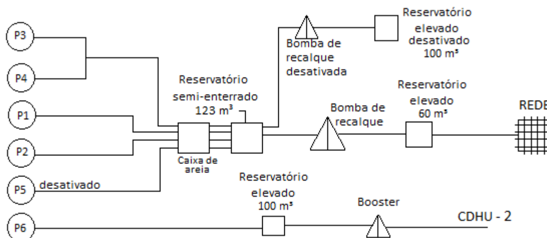
Figura 3.1 – Sistema do abastecimento de água de Parisi
