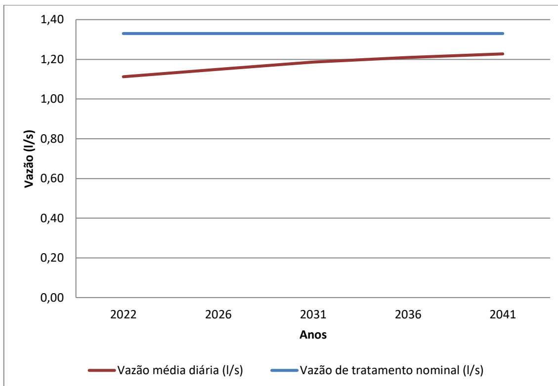
Gráfico 8.12 – Vazão Média Diária (l/s) x Capacidade nominal da ETE (l/s)
