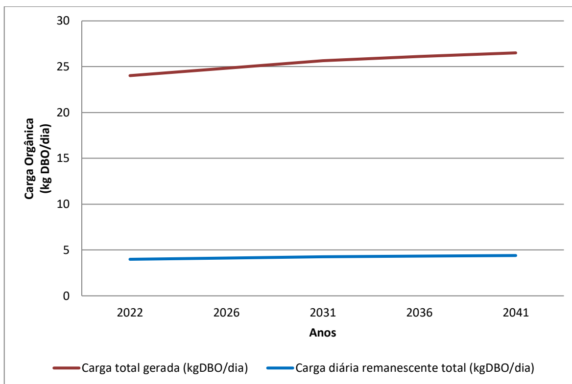
Gráfico 8.13 - Evolução de Cargas Orgânicas (Kg DBO/Dia)
