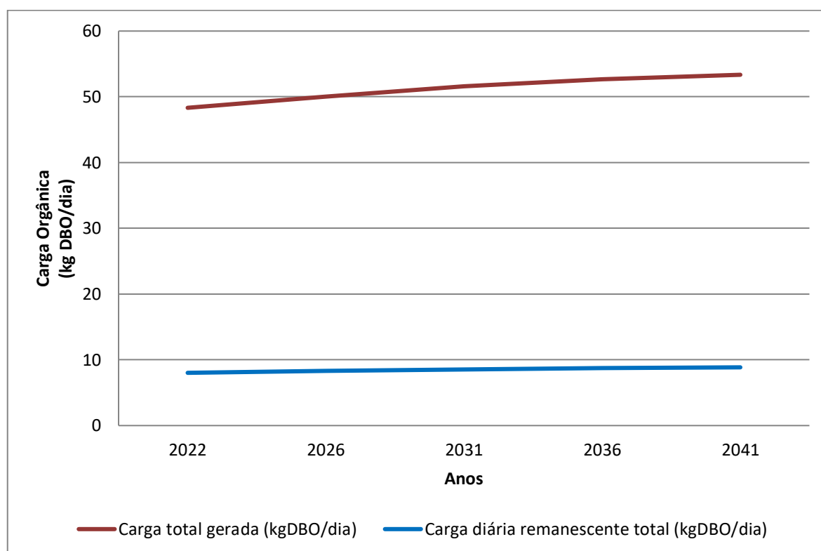
Gráfico 8.11 - Evolução de Cargas Orgânicas (Kg DBO/Dia)
