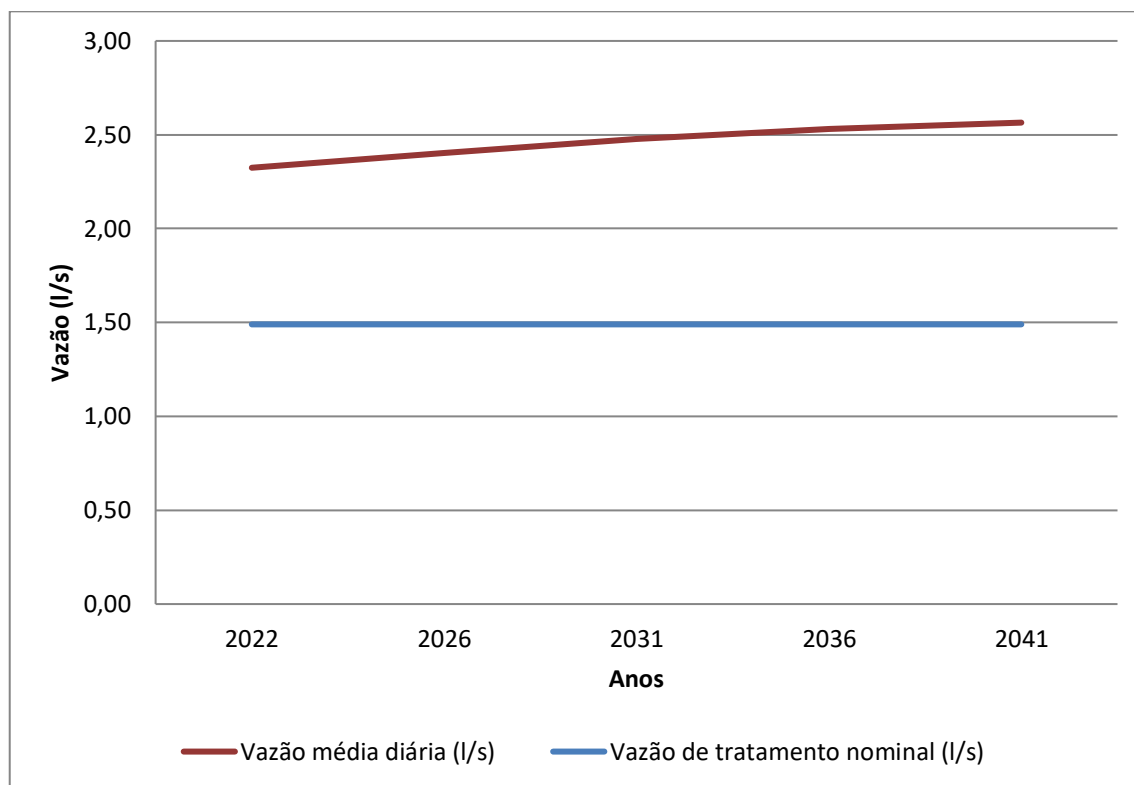
Gráfico 8.10 – Vazão Média Diária (l/s) x Capacidade nominal da ETE (l/s)
