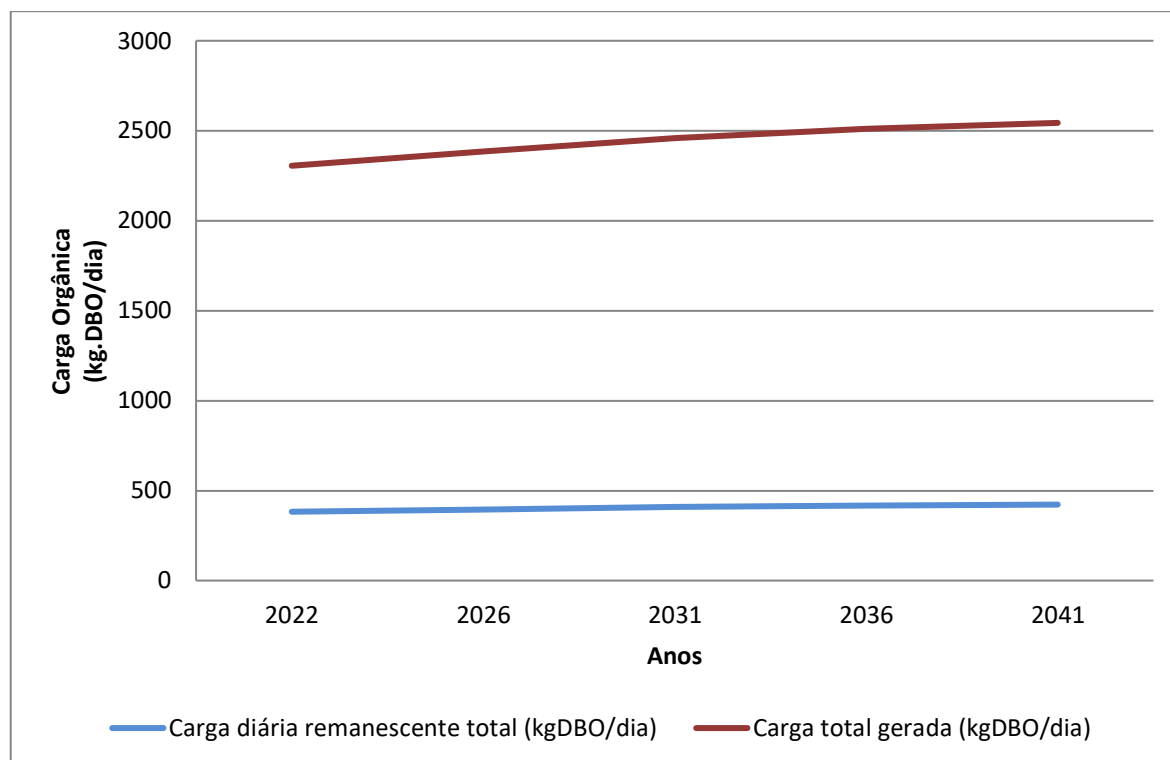
Gráfico 8.7 - Evolução de Cargas Orgânicas (Kg DBO/Dia)
