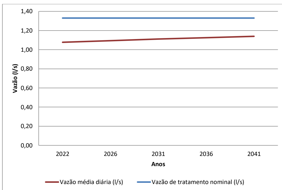
Gráfico 8.13 – Vazão Média Diária (l/s) x Vazão de Tratamento Nominal da ETE (l/s)
