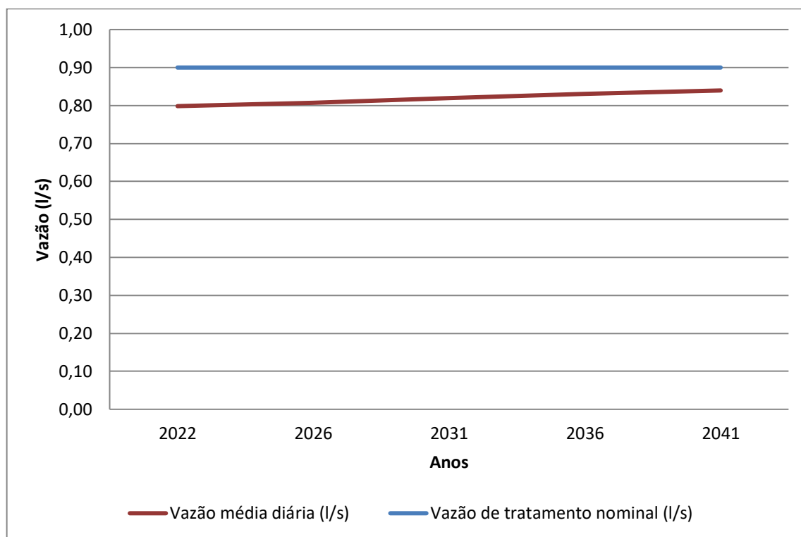
Gráfico 8.11 – Vazão Média Diária (l/s) x Vazão de Tratamento Nominal da ETE (l/s)
