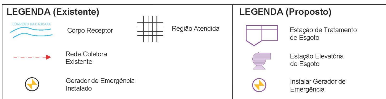
Figura 10.2 – Croqui do Sistema de Esgotamento Sanitário Proposto para o Subsistema da Sede Urbana
