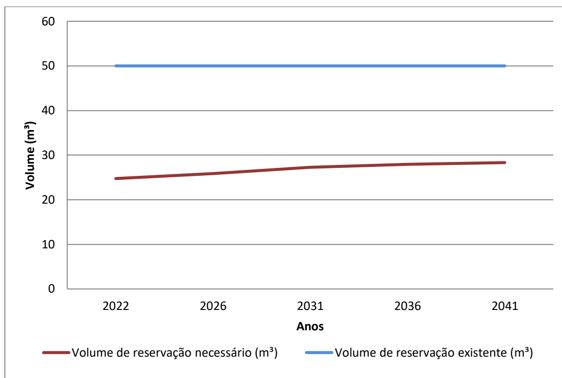
Gráfico 8.6 - Volume de Reservação Necessário (m³) x Volume de Reservação Existente (m³)
