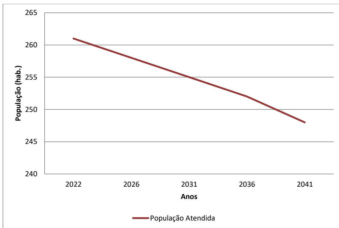
Gráfico 7.5 – População Atendida (hab.) x Anos de Planejamento – Vila Primavera
