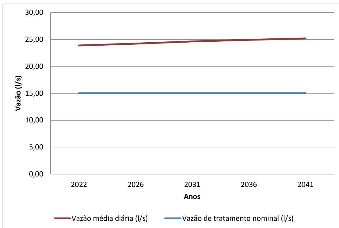
Gráfico 8.9 – Vazão Média Diária (l/s) x Vazão de Tratamento Nominal da ETE (l/s)
