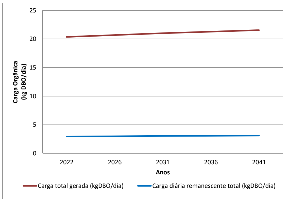
Gráfico 8.14 - Evolução de Cargas Orgânicas (Kg DBO/Dia)
