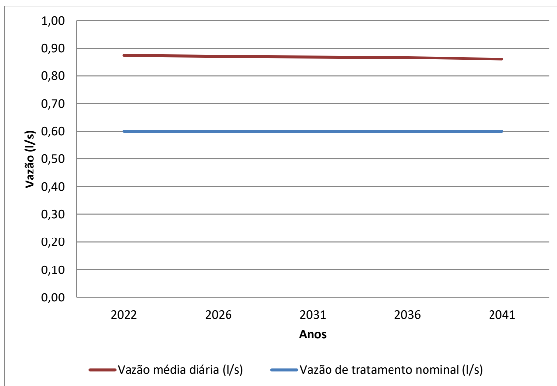
Gráfico 8.15 – Vazão Média Diária (l/s) x Vazão de Tratamento Nominal da ETE (l/s)
