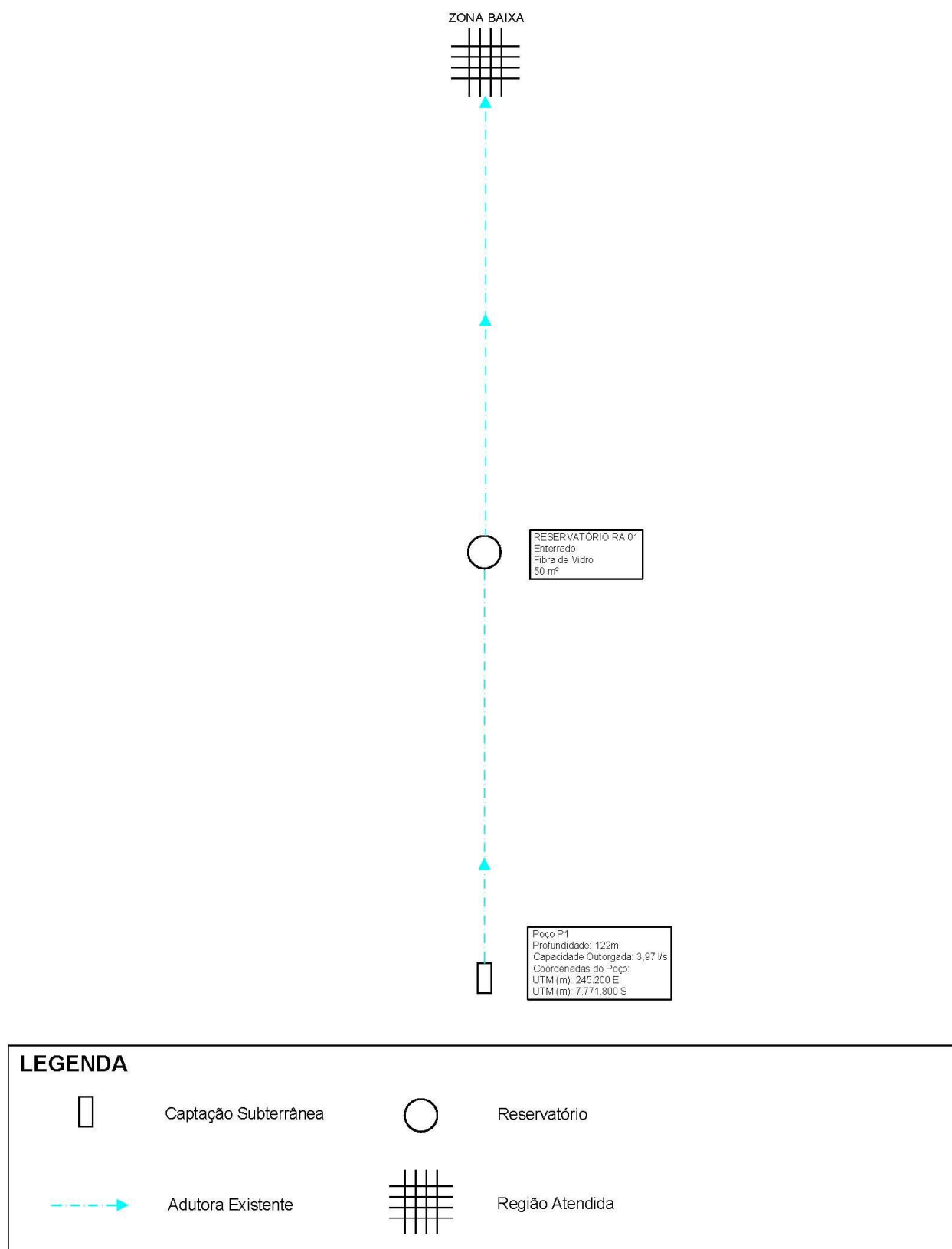
Figura 4.3 – Croqui do Sistema de Abastecimento de Água Existente – Iguaçu.
