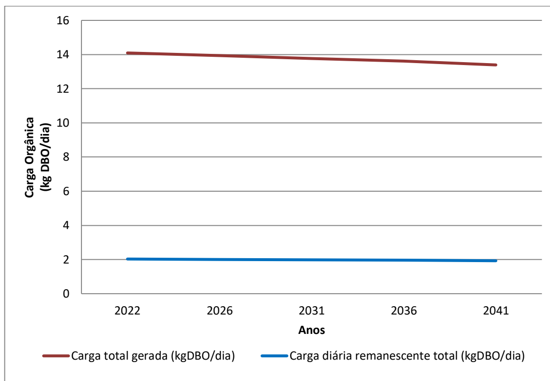
Gráfico 8.16 - Evolução de Cargas Orgânicas (Kg DBO/Dia)
