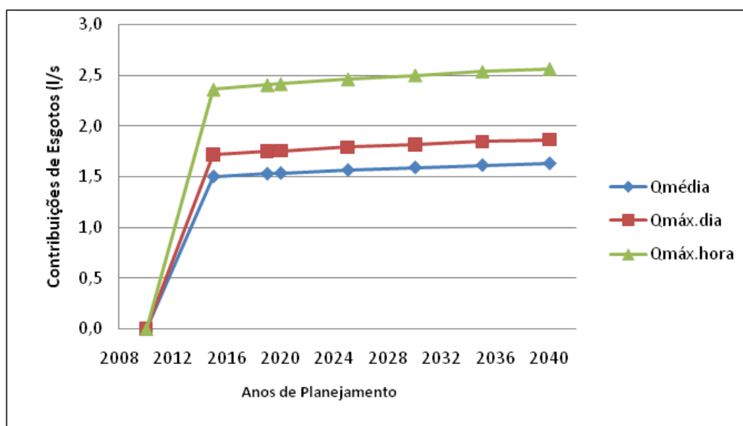
Gráfico 2.11 – Evolução das contribuições de esgotos - Bairro Jurupará
