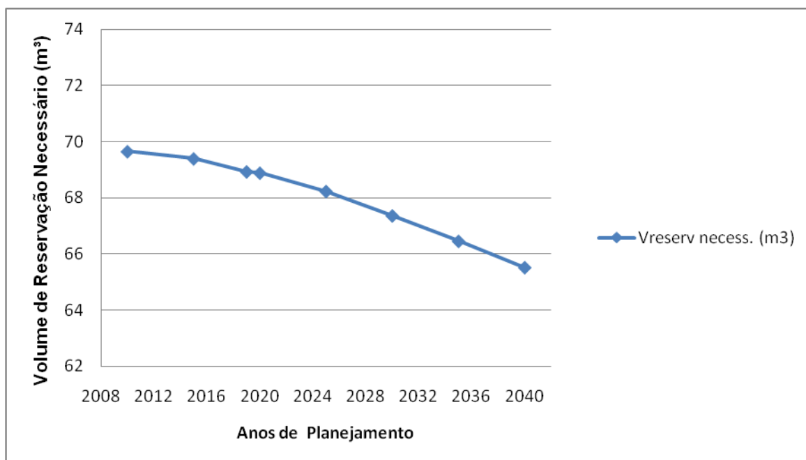
Gráfico 2.5 – Evolução dos Volumes de Reservação Necessários - Bairro Jurupará
