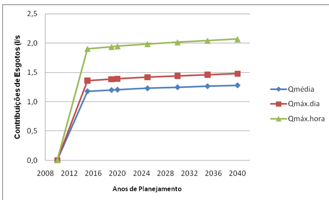
Gráfico 2.13 – Evolução das contribuições de esgotos – Bairro dos Leites
