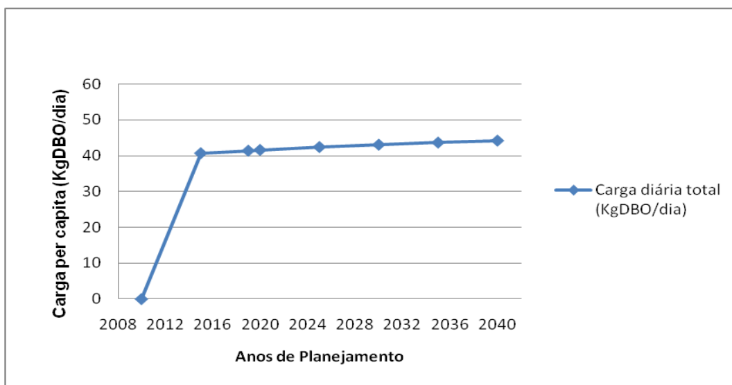
Gráfico 2.12 – Evolução das Cargas Orgânicas – Bairro Jurupará
