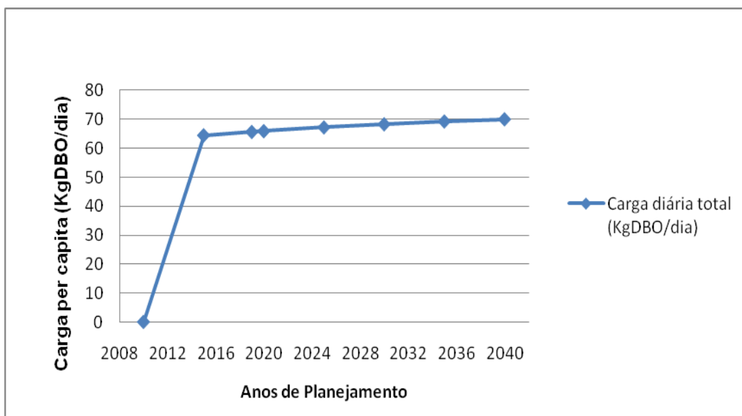
Gráfico 2.14 – Evolução das Cargas Orgânicas– Bairro dos Leites
