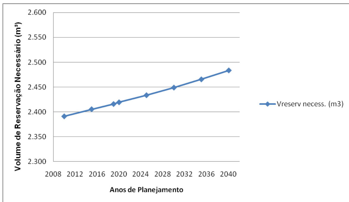
Gráfico 2.3 – Evolução dos Volumes de Reservação Necessários - Sede de Piedade
