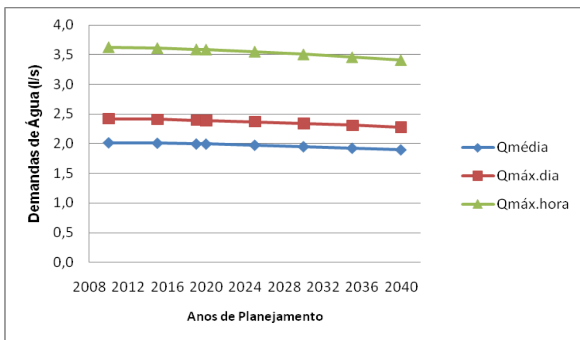
Gráfico 2.4 – Evolução das demandas/vazões disponibilizadas para distribuição – Bairro Jurupará
