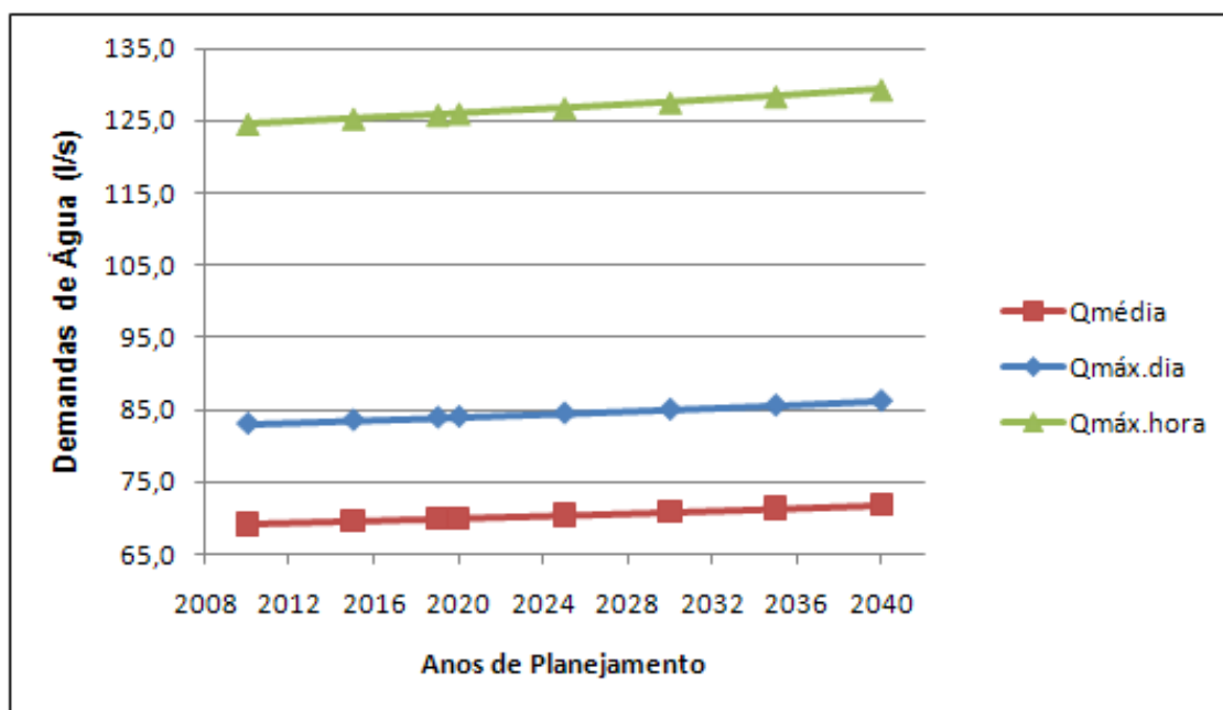
Gráfico 2.2 – Evolução das demandas/vazões disponibilizadas para distribuição – Sede de Piedade
