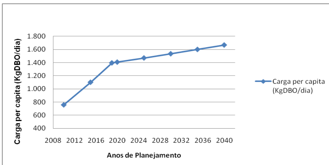
Gráfico 2.10 – Evolução das Cargas Orgânicas – Sede de Piedade
