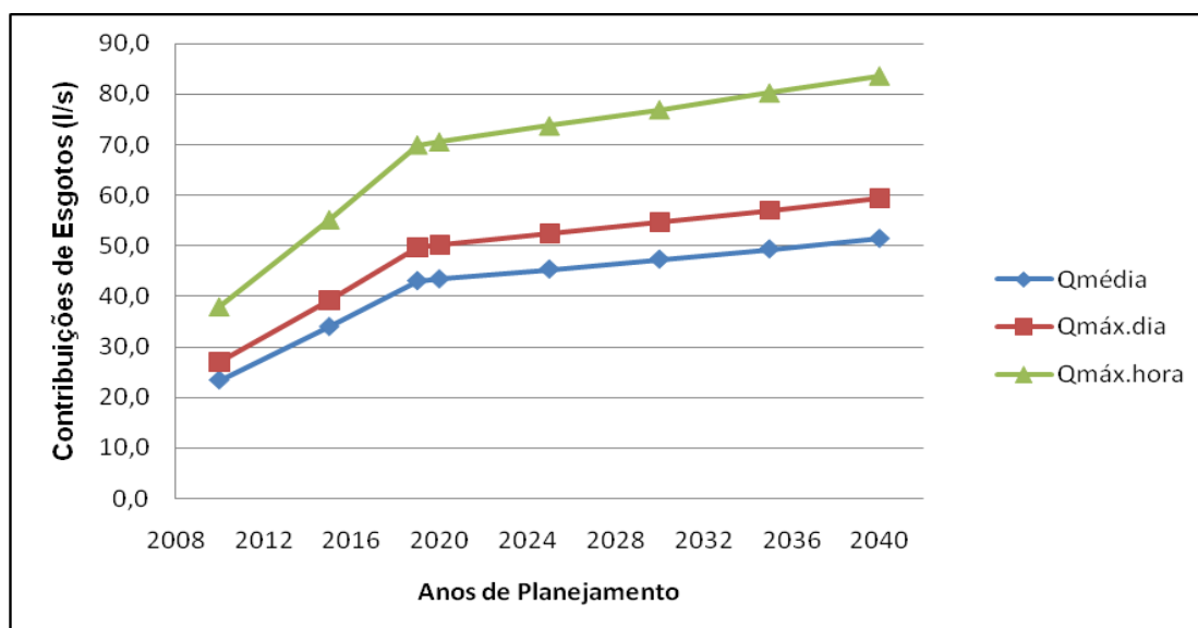
Gráfico 2.9 – Evolução das contribuições de esgotos – sede de Piedade
