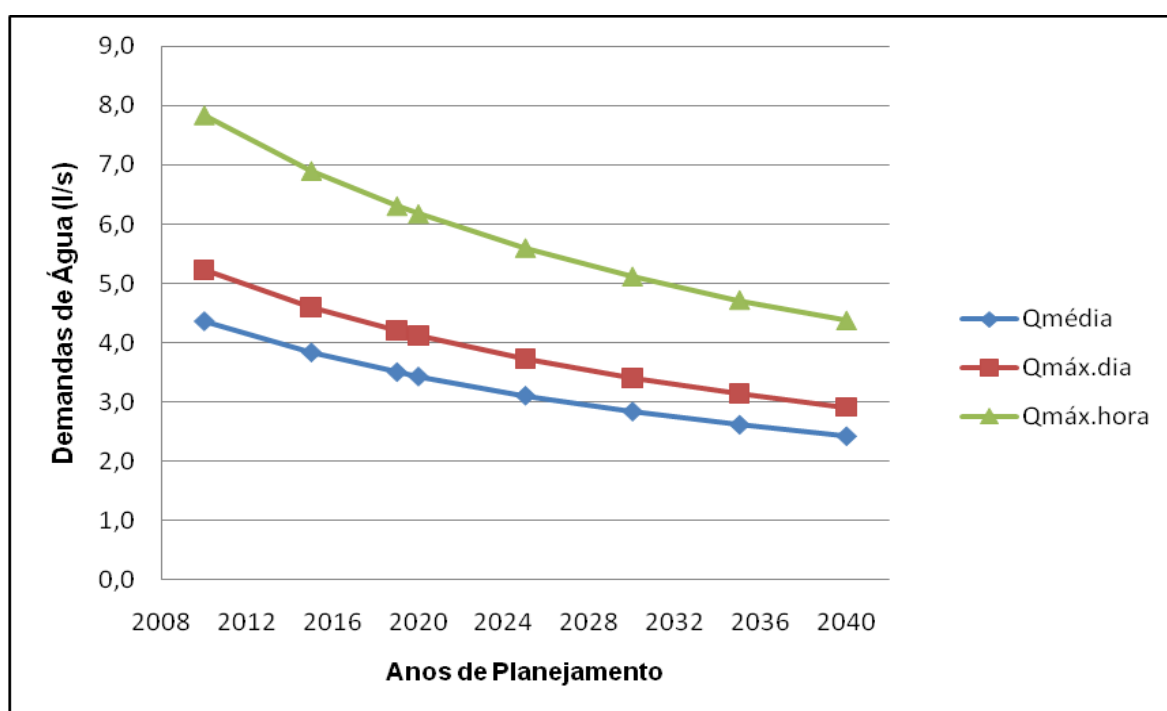
Gráfico 2.6 – Evolução das demandas/vazões disponibilizadas para distribuição – Bairro dos Leites
