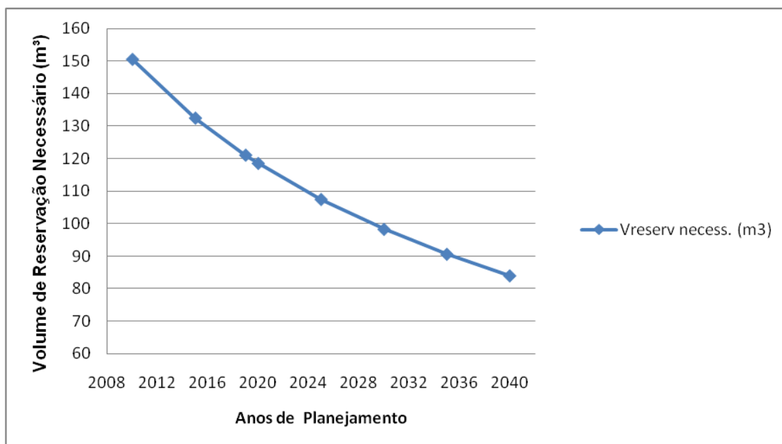
Gráfico 2.7 – Evolução dos Volumes de Reservação Necessários - Bairro dos Leites
