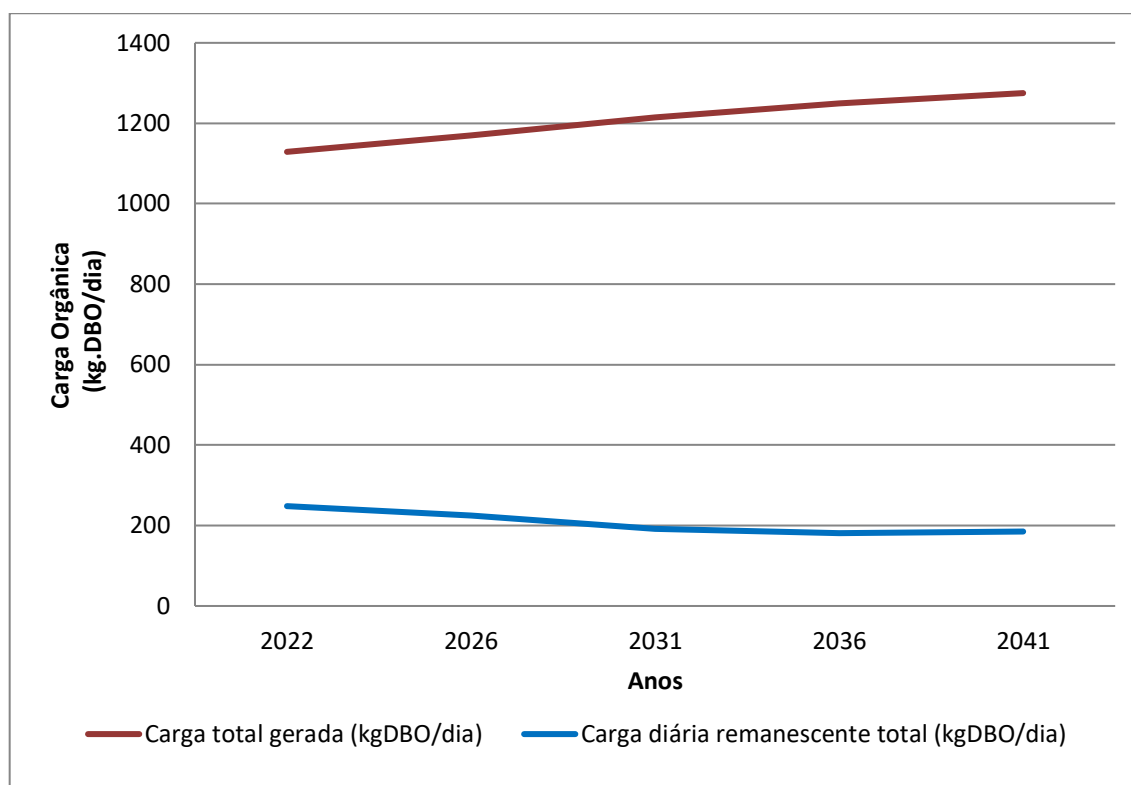
Gráfico 8.6 - Evolução de Cargas Orgânicas (Kg DBO/Dia)
