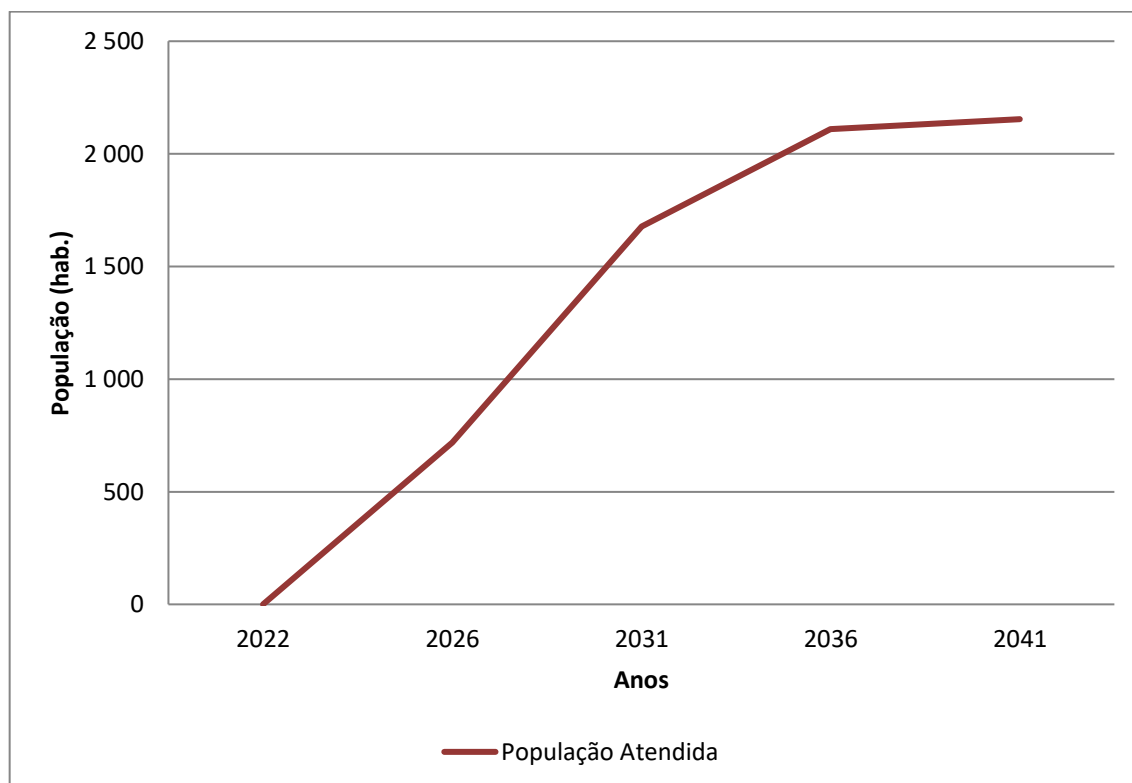
Gráfico 7.8 - População Atendida (hab.) x Anos de Planejamento – Jd. Cananeia e Chácaras Reunidas
