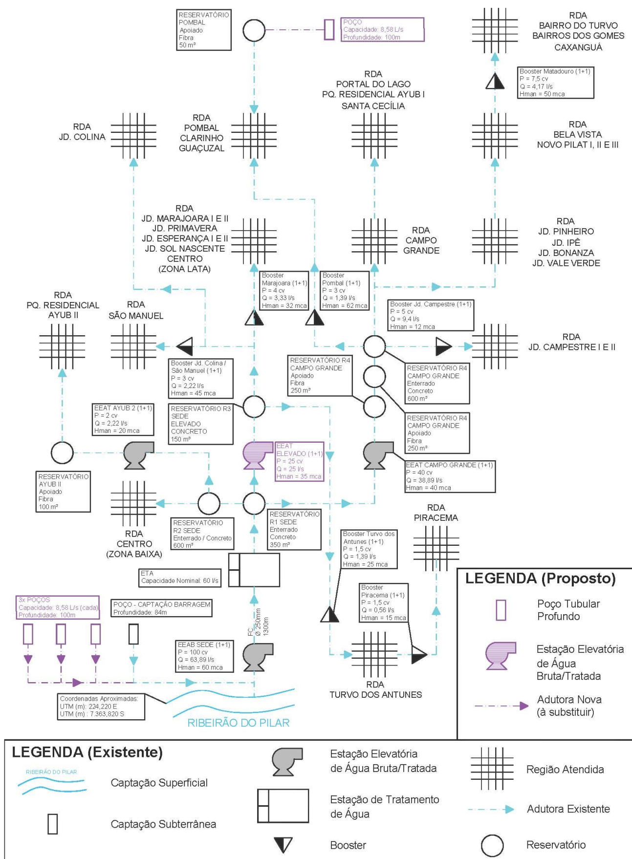
Figura 10.1 – Croqui do Sistema de Abastecimento de Água Proposto para o Sistema Sede Urbana
