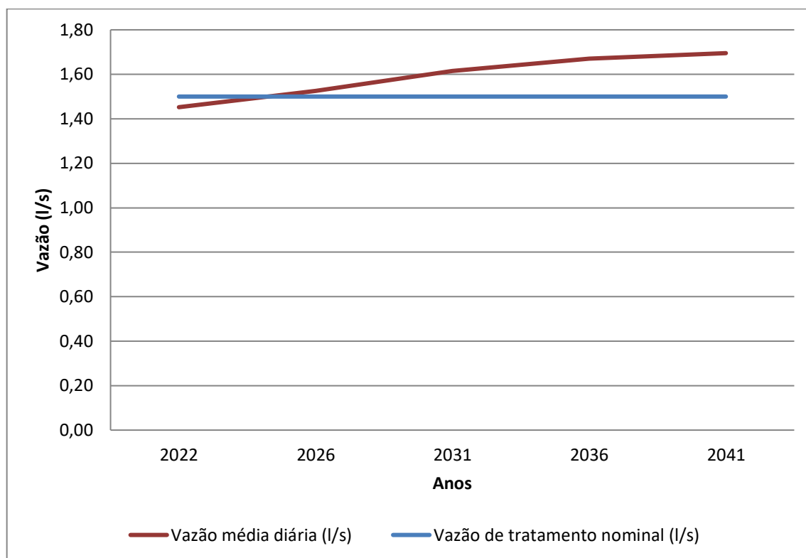
Gráfico 8.7 – Vazão Média Diária (l/s) x Vazão de Tratamento Nominal da ETE (l/s)
