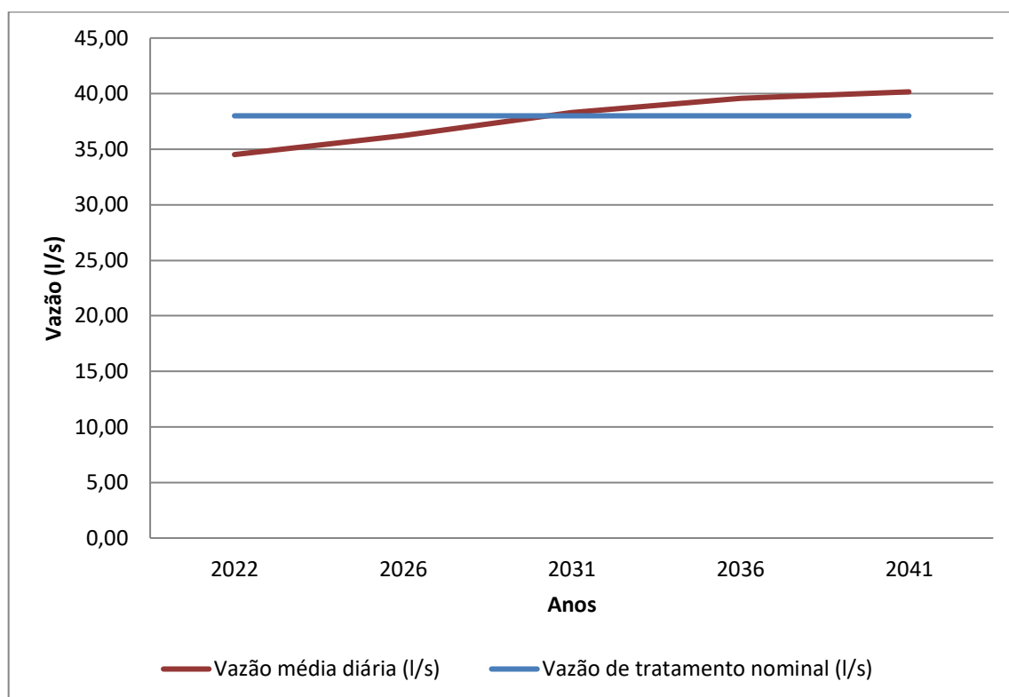
Gráfico 8.5 – Vazão Média Diária (l/s) x Vazão de Tratamento Nominal da ETE (l/s)
