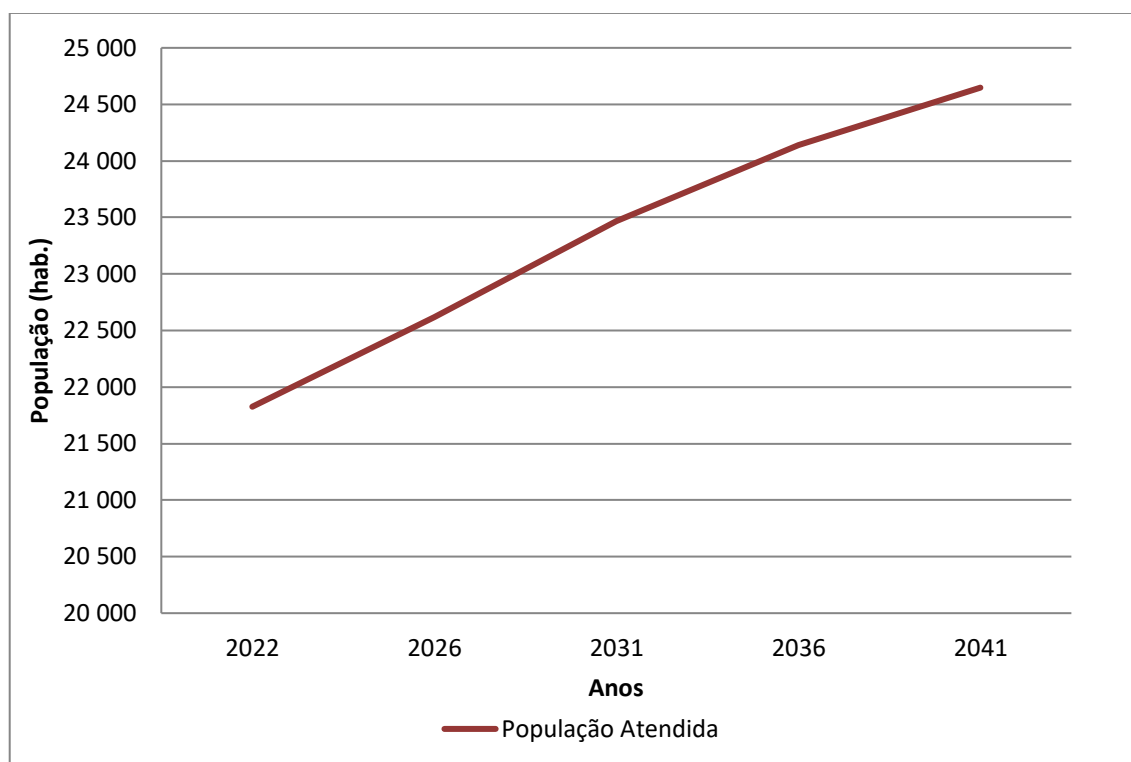
Gráfico 7.2 – População Atendida (hab.) x Anos de Planejamento – Sede Urbana+São Manoel
