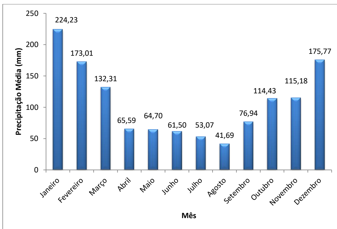
Gráfico 3.1 – Precipitação Média Mensal no Período de 1937 a 2020, Estação E4 028
