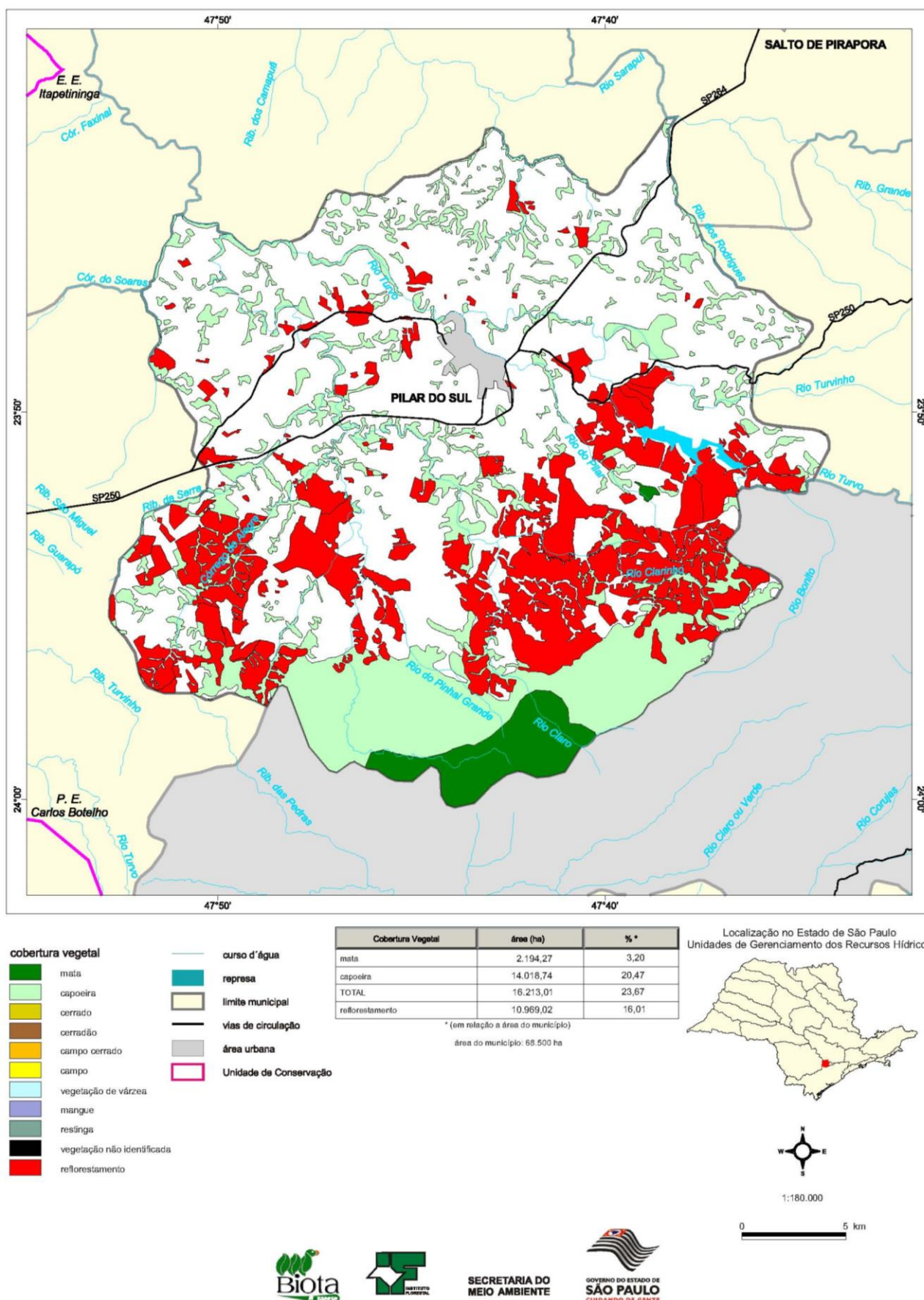
Figura 3.2 – Cobertura Vegetal no Município de Pilar do Sul
