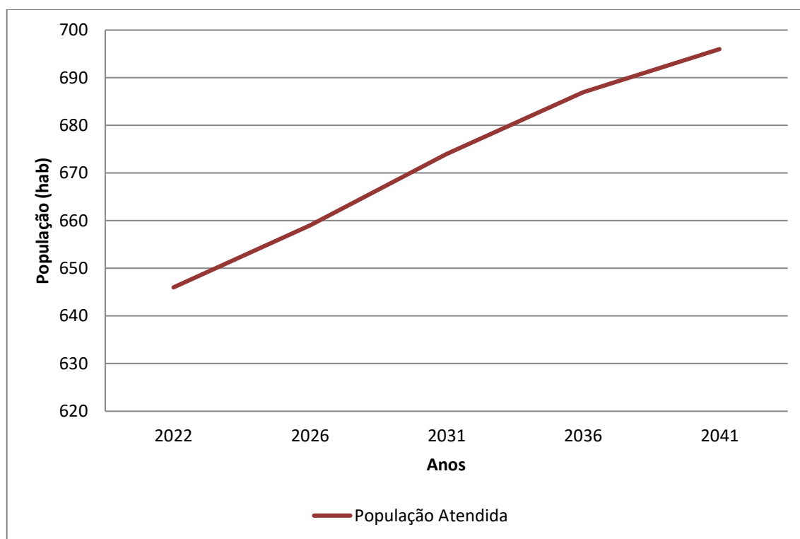
Gráfico 7.4 – População Atendida (hab.) x Anos de Planejamento – Paineiras
