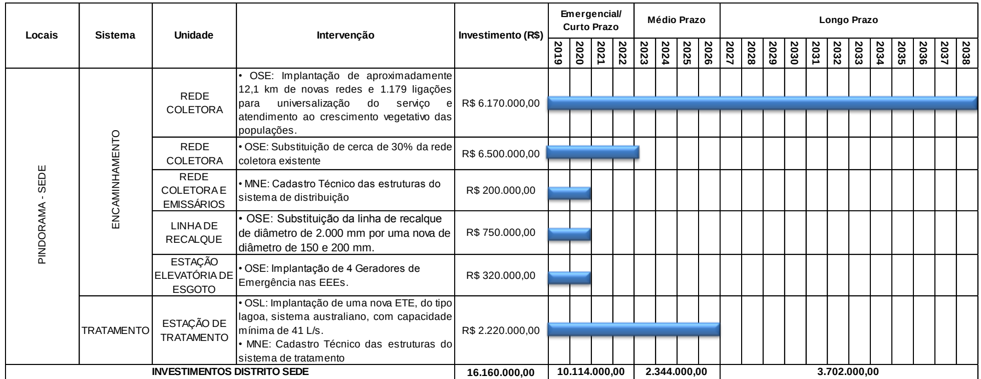
Figura 10.3 - Cronograma de Implantação das Intervenções Propostas no Sistema de Esgotos Sanitários
