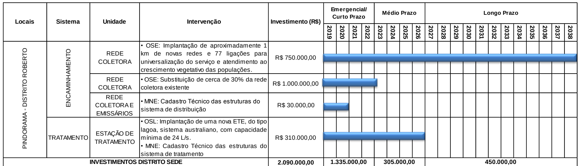
Figura 10.4 - Cronograma de Implantação das Intervenções Propostas no Sistema de Esgotos Sanitários
