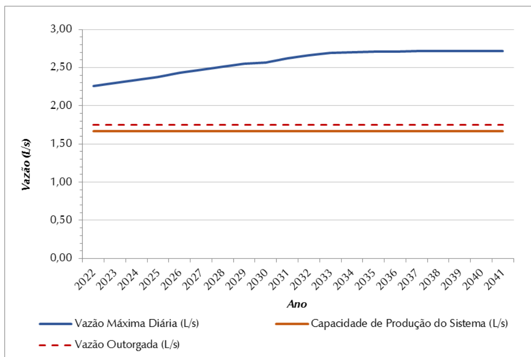
Figura 8.3 – Demandas Máximas Diárias (L/s) X Vazão Captada (L/s) – SAA Itororó do Paranapanema
