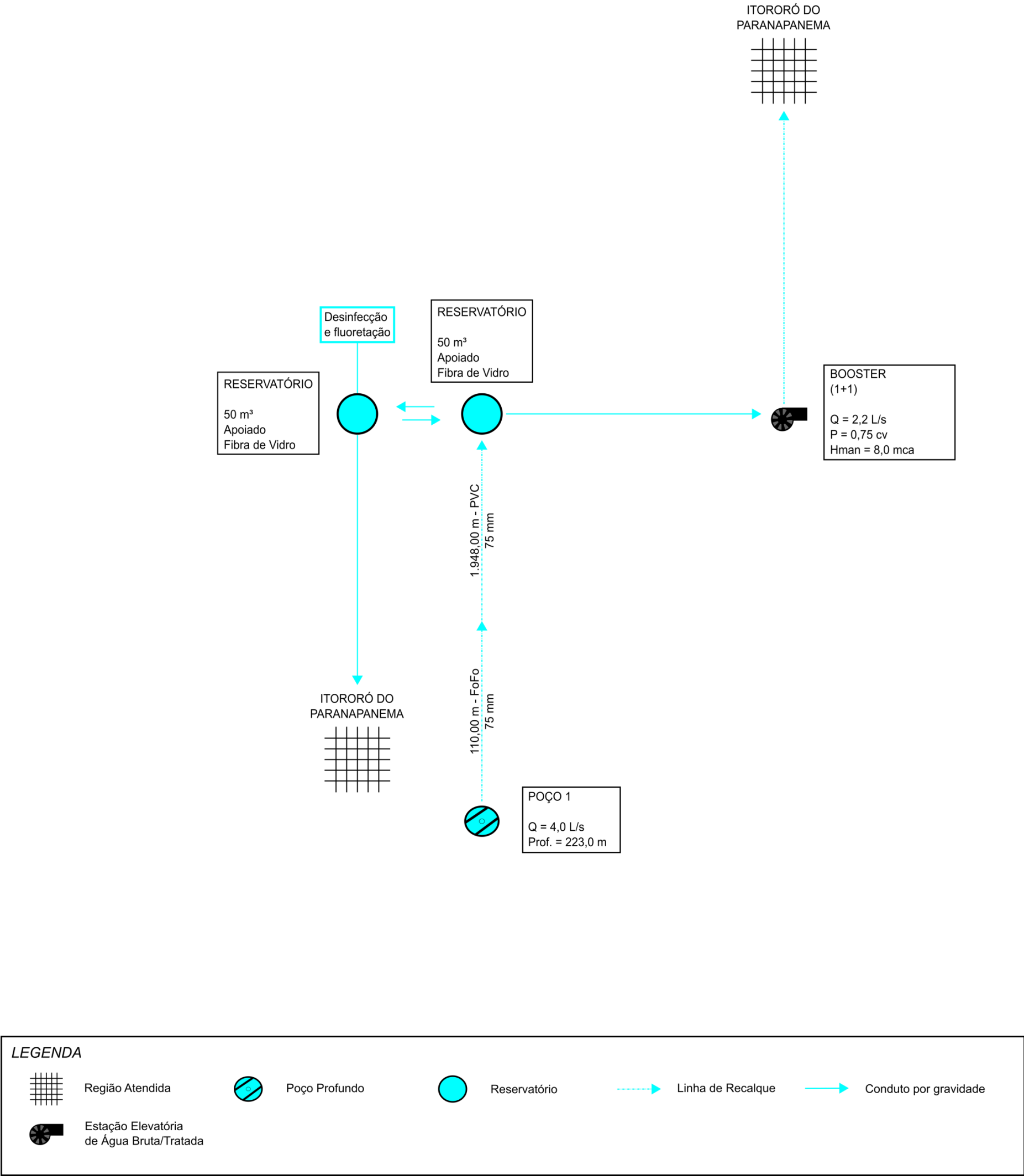
Figura 4.2 – Croqui do Sistema de Abastecimento de Água Itororó do Paranapanema
