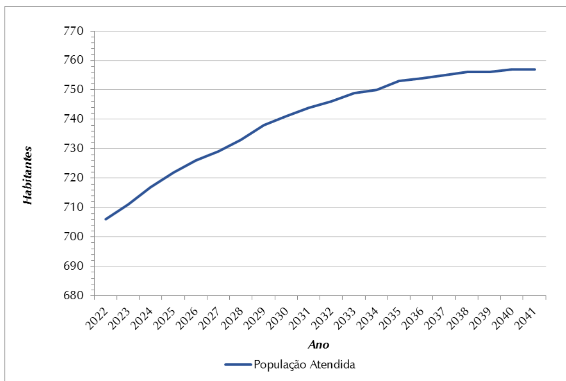
Figura 7.3 – Evolução da População Atendida (hab.) – SAA Itororó do Paranapanema
