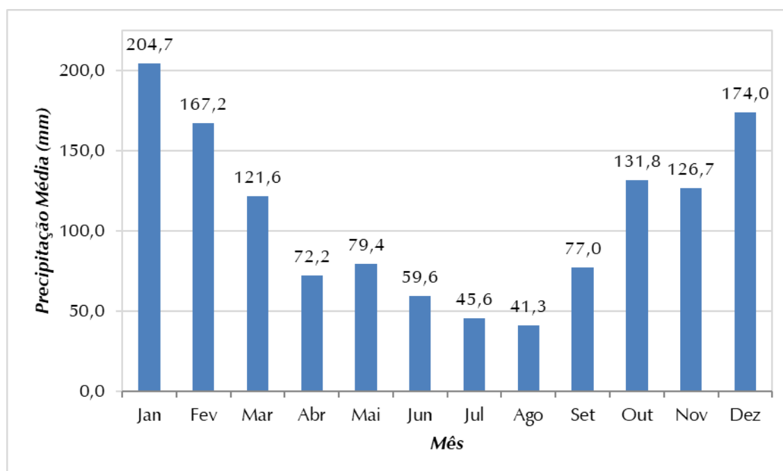
Figura 3.2 - Precipitação Média Mensal no Período de 1947 a 2021, Estação D8-025
