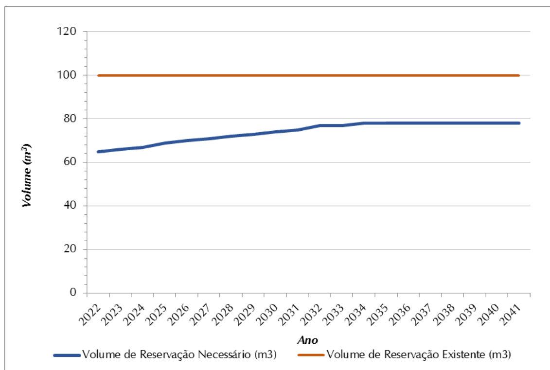
Figura 8.4 - Volume de Reservação Necessário (m³) x Volume de Reservação Atual (m³) – SAA Itororó do Paranapanema
