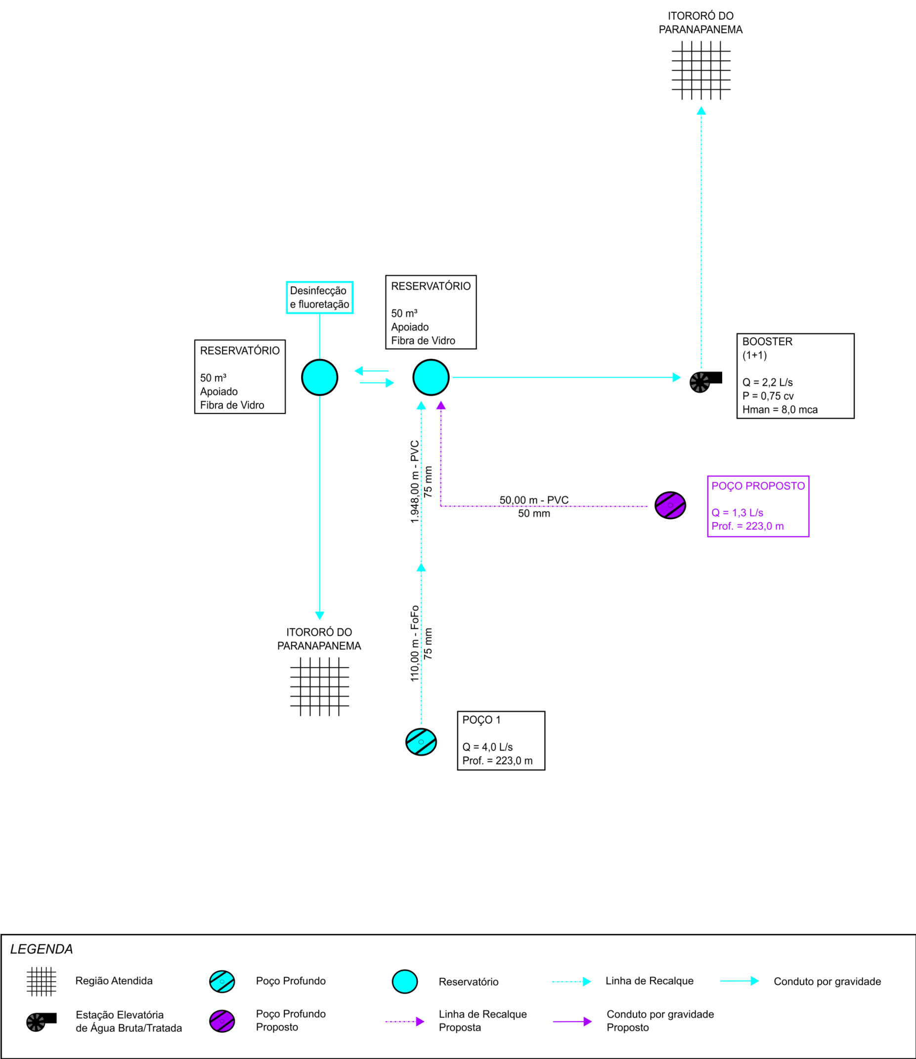
Figura 10.2 – Croqui das intervenções propostas para o sistema de abastecimento de água Itororó do Paranapanema
