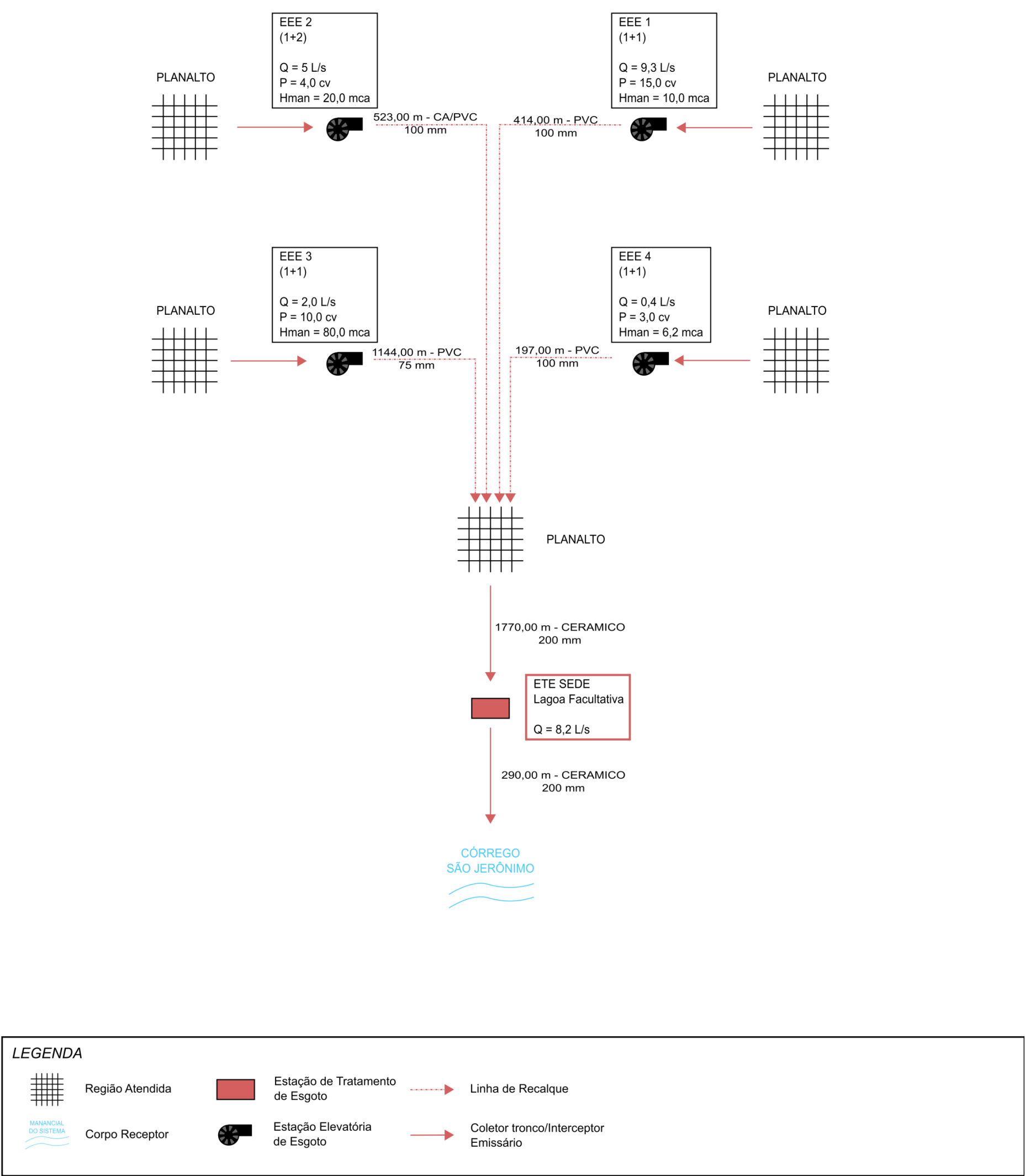
Figura 4.2 – Croqui do Sistema de Esgotamento Sanitário da Sede de Planalto Fonte: SABESP, 2021.
