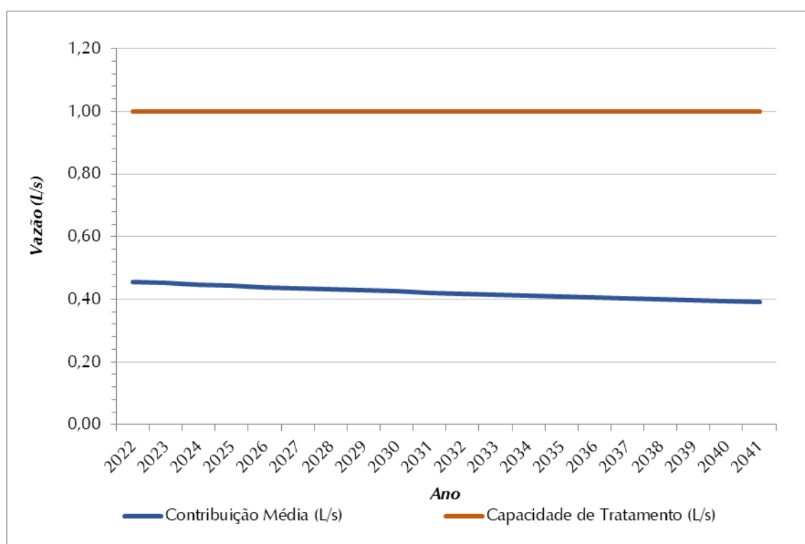
Figura 8.7 – Contribuição Média Total (L/s) x Capacidade de Tratamento de Esgoto (L/s) – SES Distrito Povoado do Sol
