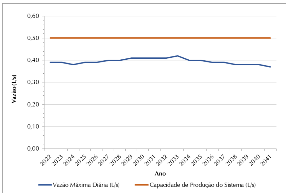
Figura 8.3 – Demandas Máximas Diárias (L/s) X Vazão Captada (L/s) – SAA Povoado do Sol
