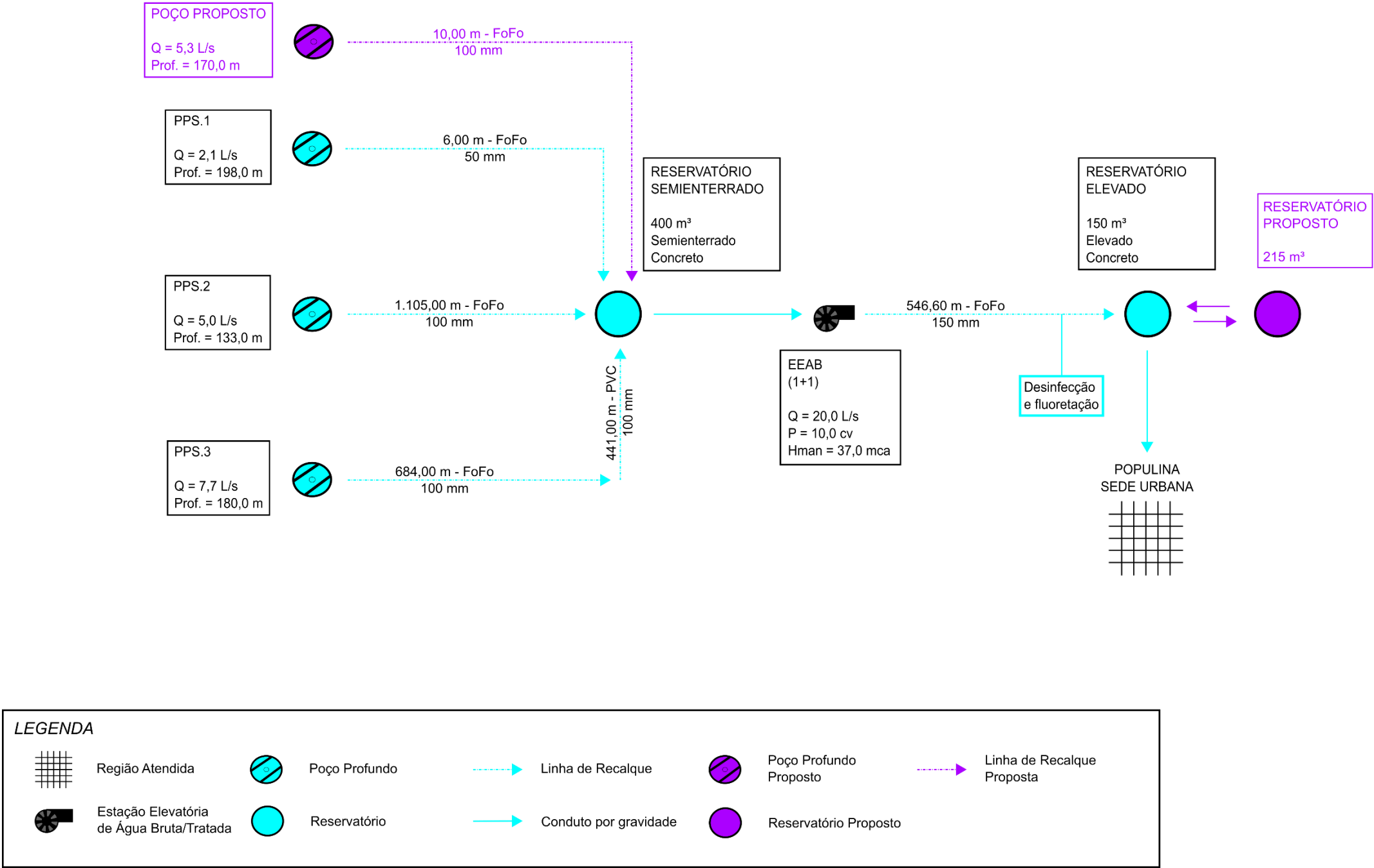
Figura 10.1 – Croqui das intervenções propostas para o sistema de abastecimento de água Sede.
