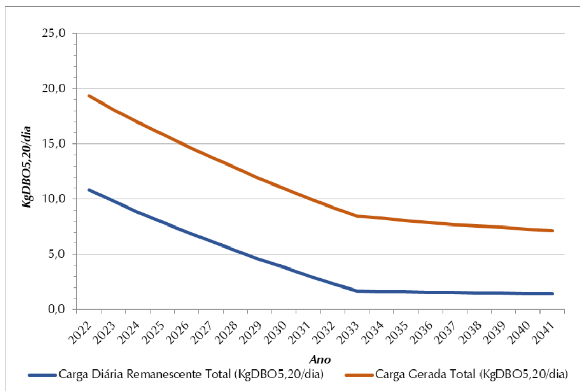
Figura 8.8 - Evolução de Cargas Orgânicas (Kg DBO 5,20 /Dia) – SES Distrito Povoado do Sol
