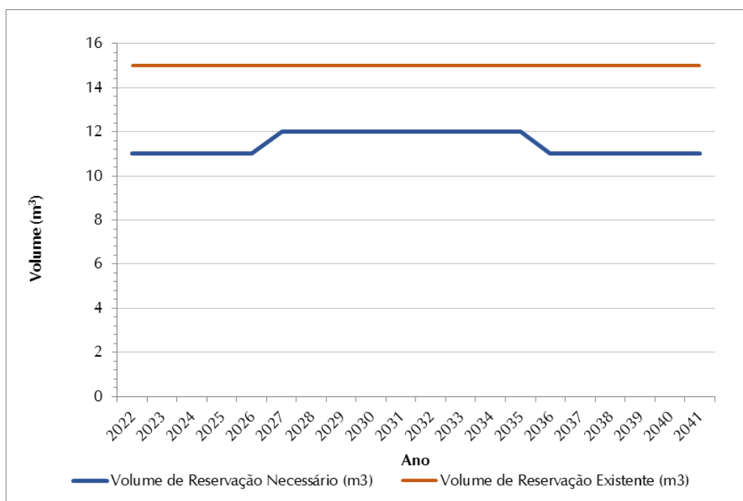
Figura 8.4 - Volume de Reservação Necessário (m³) x Volume de Reservação Atual (m³) – SAA Povoado do Sol
