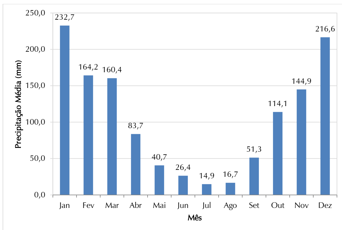
Figura 3.2 - Precipitação Média Mensal no Período de 1959 a 2001, Estação A7-001
