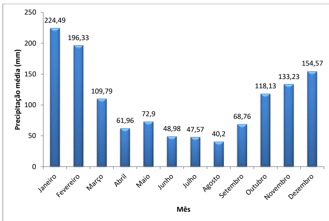
Gráfico 3.1 – Precipitação Média Mensal no Período de 1939 a 2020, Estação ES-014
