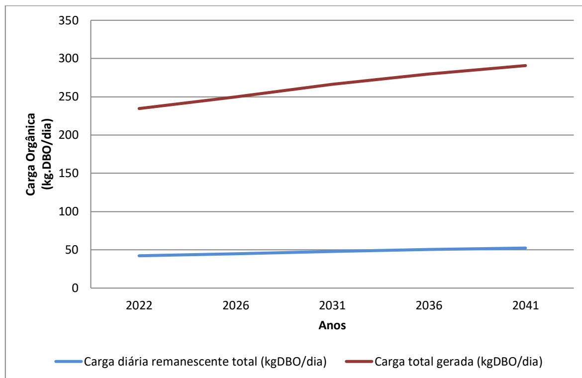
Gráfico 8.3 - Evolução de Cargas Orgânicas (Kg DBO/Dia)
