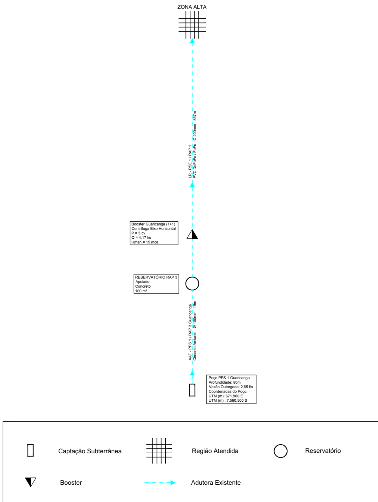
Figura 4.2 – Croqui do Sistema de Abastecimento de Água Existente – Distrito São Luiz do Guaricanga.
