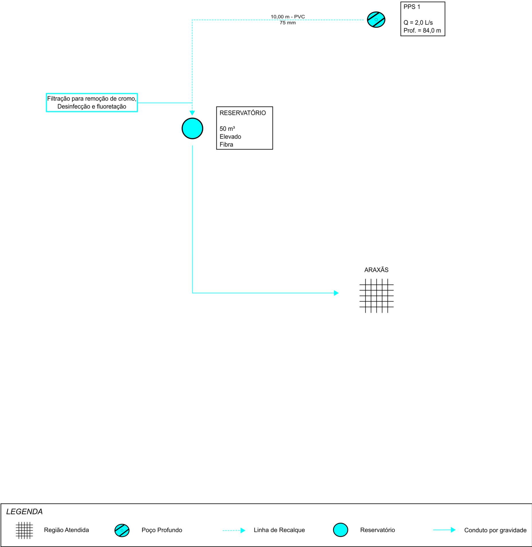
Figura 4.2 – Croqui do Sistema de Abastecimento de Água Araxás
