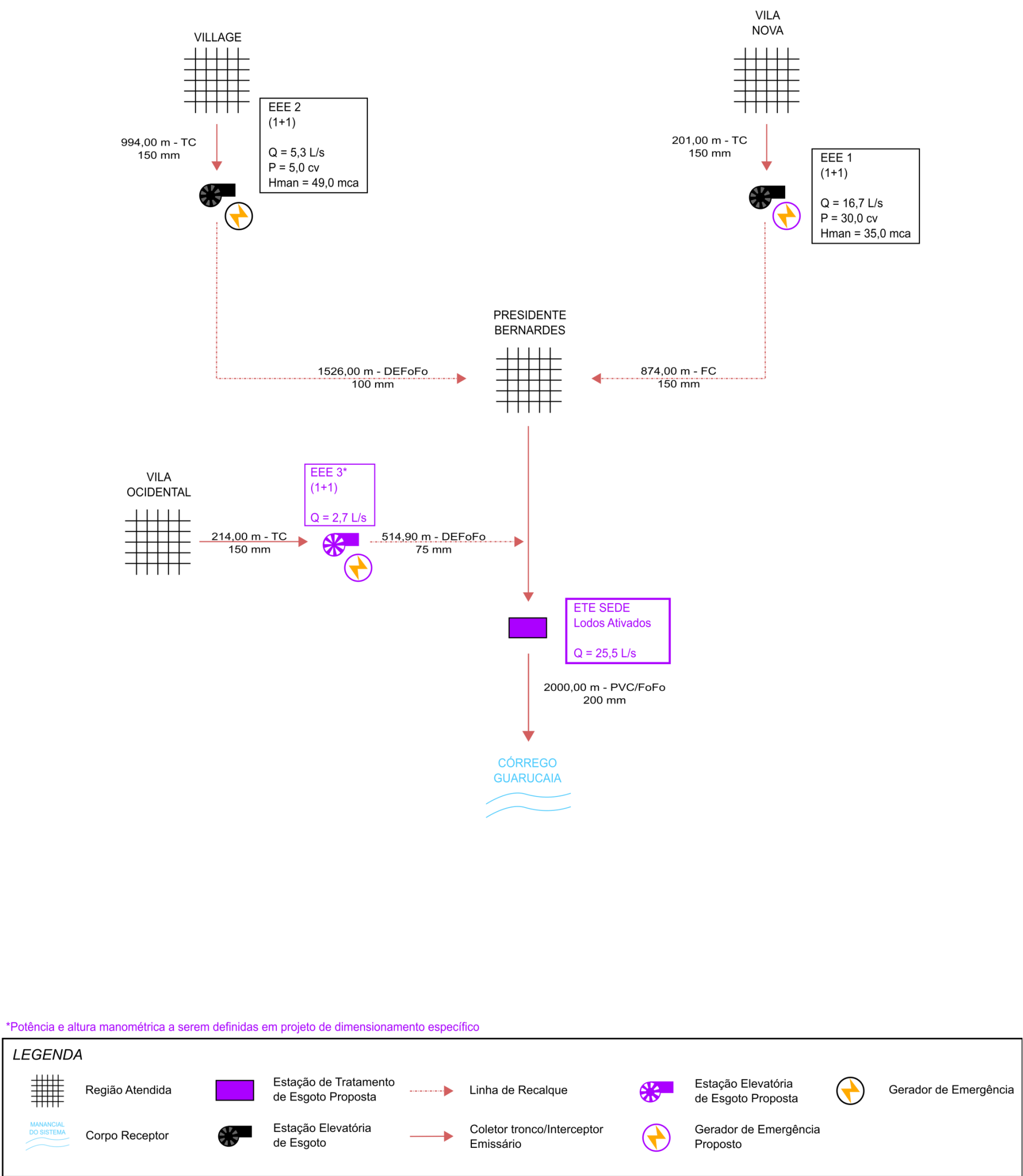
Figura 10.4 – Croqui das intervenções propostas para o sistema de esgotamento sanitário Sede
