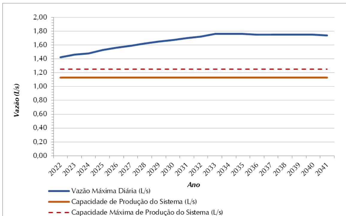
Figura 8.5 – Demandas Máximas Diárias (L/s) X Vazão Captada (L/s) – SAA Nova Pátria
