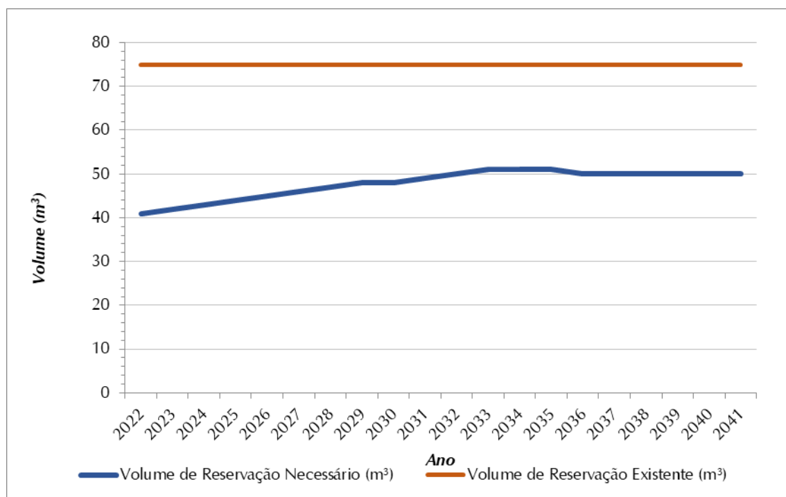
Figura 8.6 - Volume de Reservação Necessário (m³) x Volume de Reservação Atual (m³) SAA Nova Pátria
