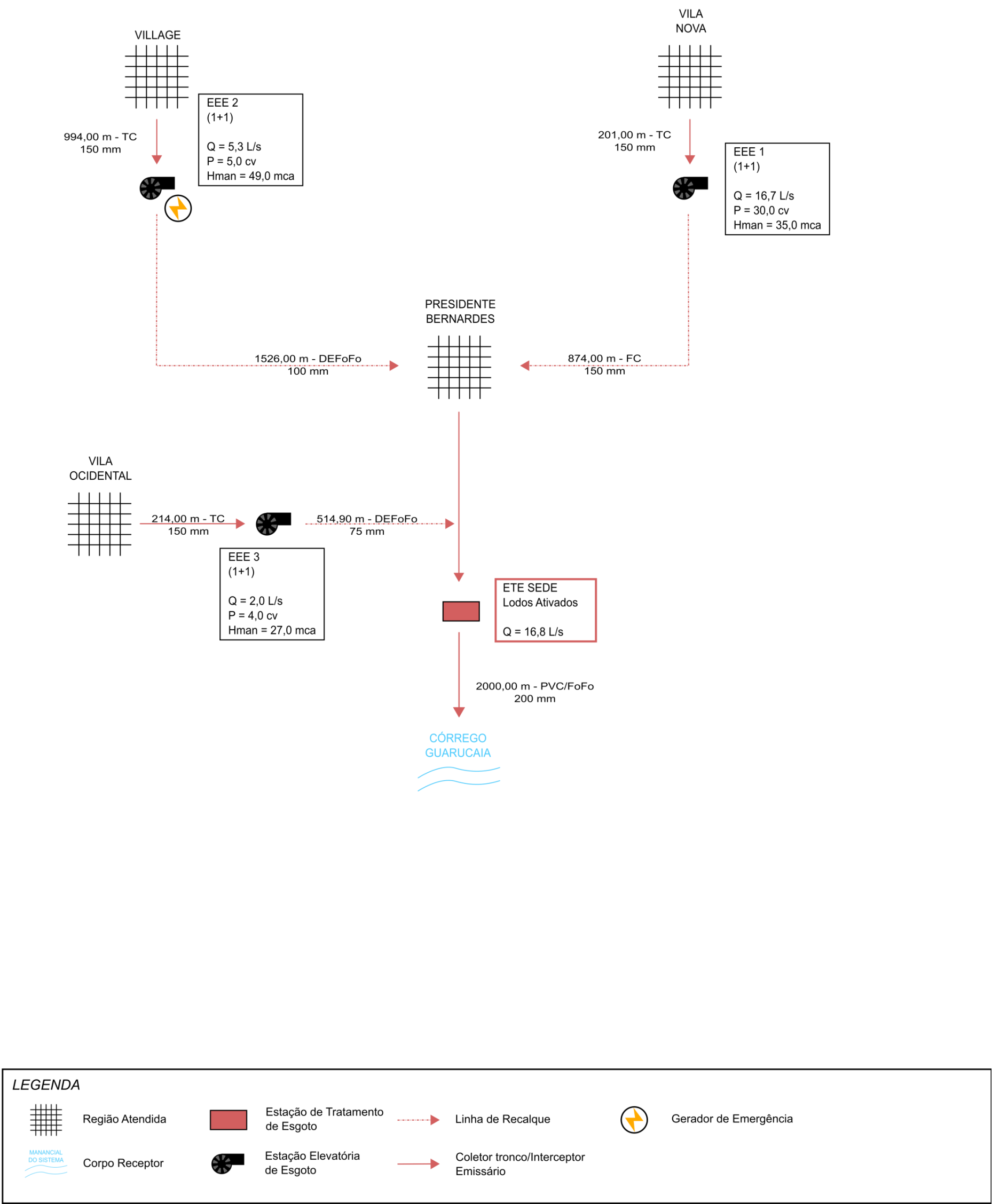
Figura 4.4 – Croqui do Sistema de Esgotamento Sanitário da Sede de Presidente Bernardes Fonte: SABESP, 2021.
