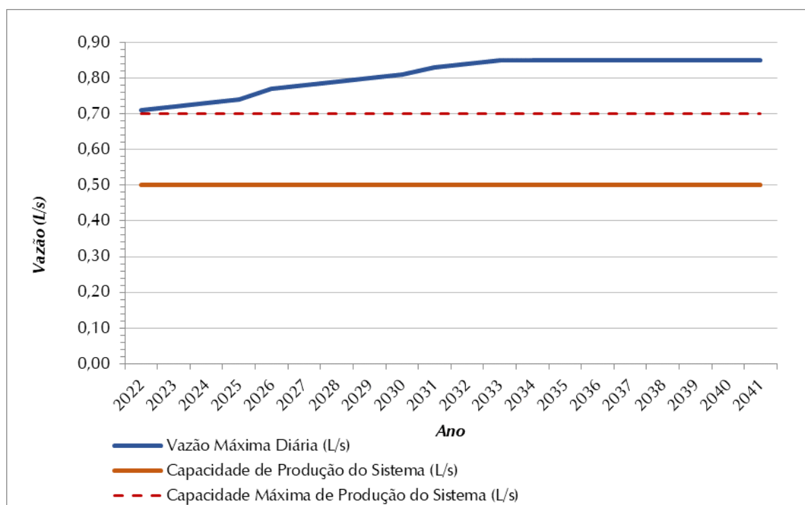
Figura 8.3 – Demandas Máximas Diárias (L/s) X Vazão Captada (L/s) – SAA Araxãs
