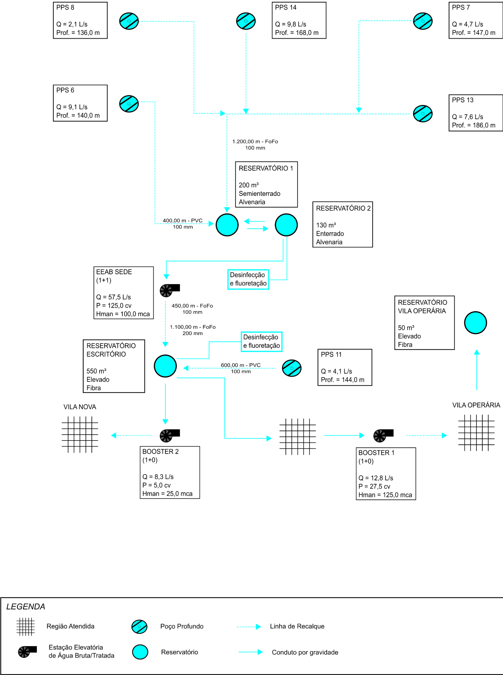
Figura 4.1 – Croqui do Sistema de Abastecimento de Água Sede Fonte: SABESP, 2021.
