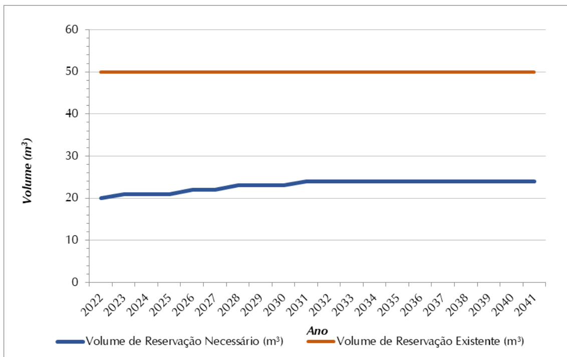
Figura 8.4 - Volume de Reservação Necessário (m³) x Volume de Reservação Atual (m³) SAA Araxãs
