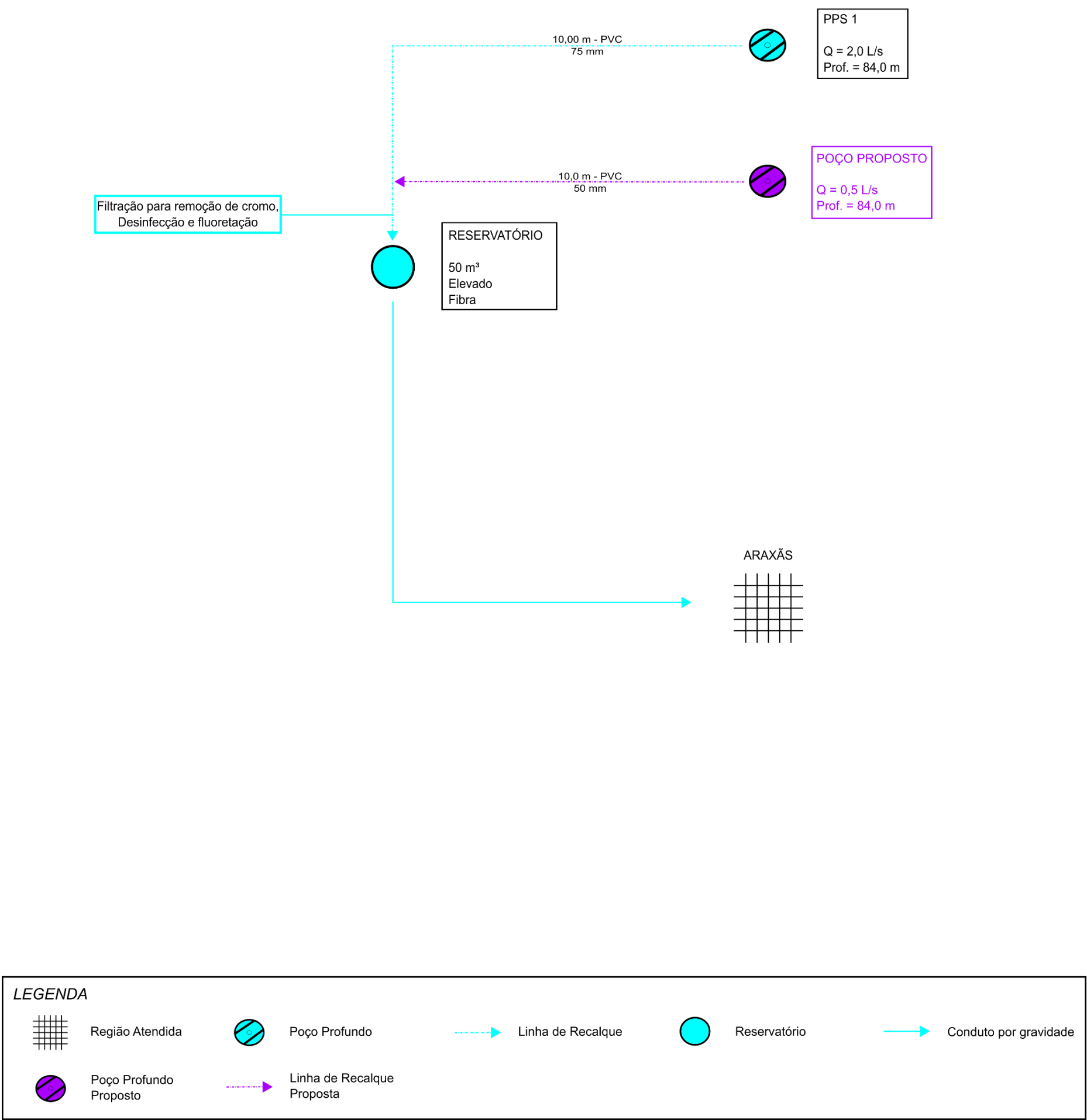
Figura 10.2 – Croqui das intervenções propostas para o sistema de abastecimento de água Araxás
