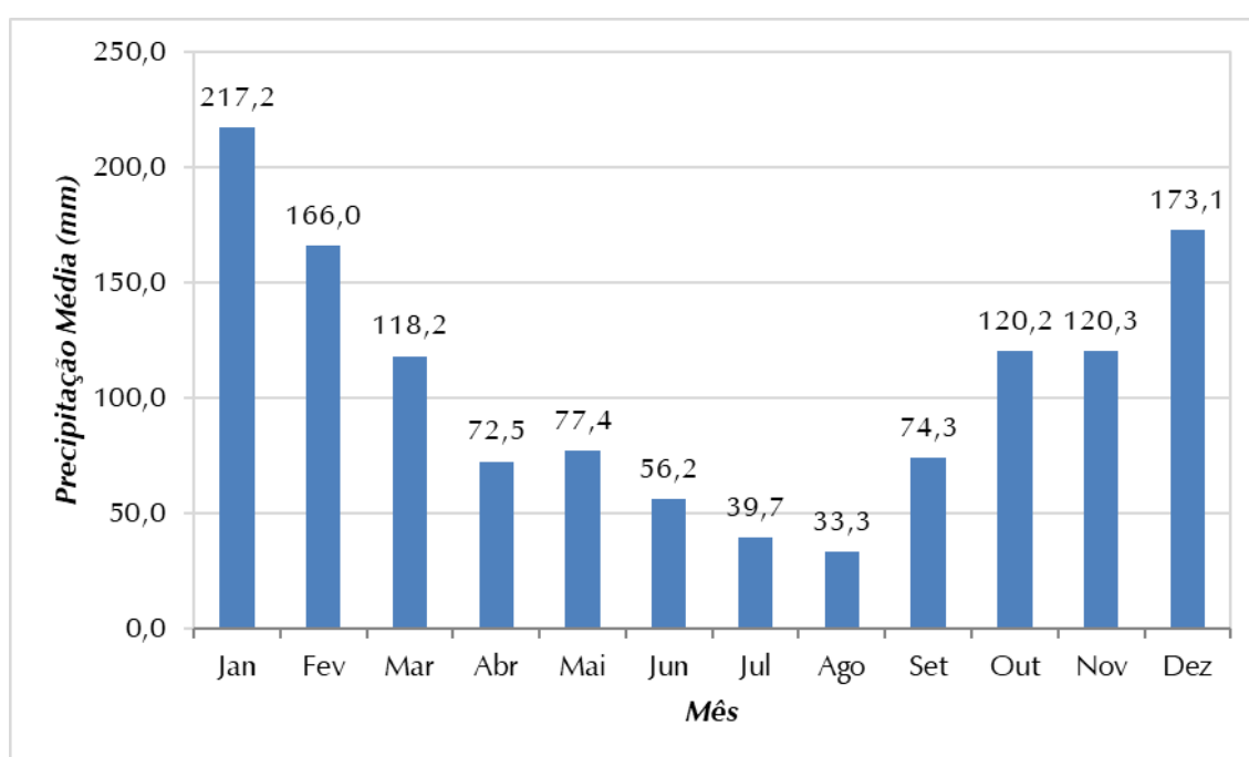
Figura 3.2 - Precipitação Média Mensal no Período de 1942 a 2021, Estação C8-009
