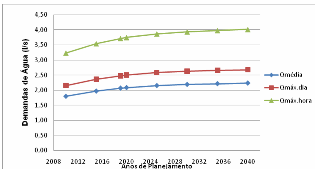
Gráfico 2.2 – Evolução das Demandas – Vazões Disponibilizadas para Distribuição – Quadra
