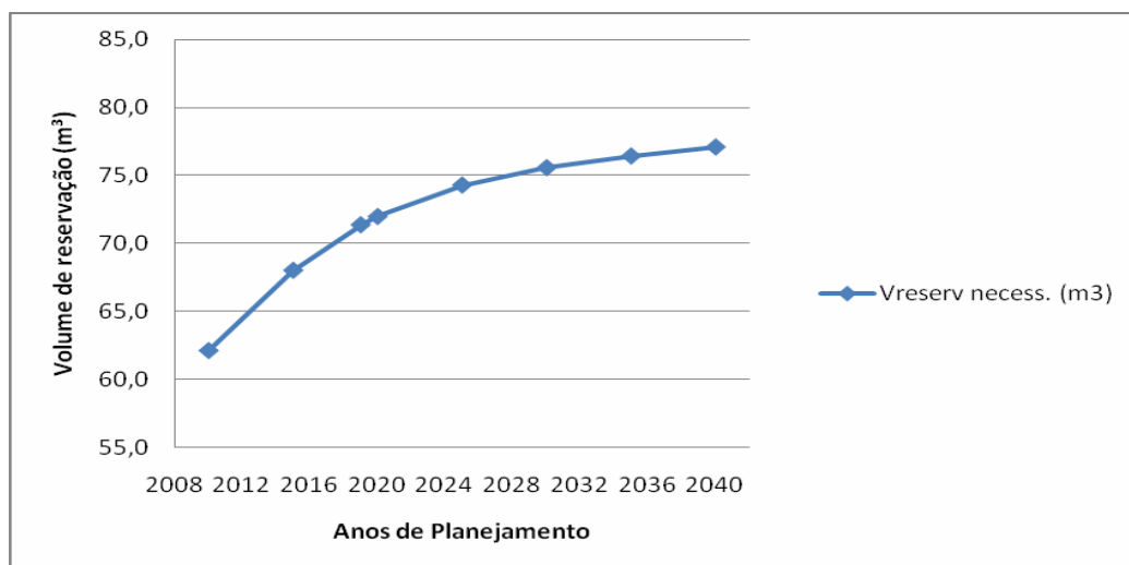
Gráfico 2.3 – Evolução dos Volumes de Reservação Necessários – m³ - Quadra
