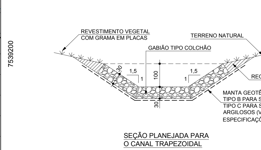
SEÇÃO PLANEJADA PARA O CANAL TRAPEZOIDAL
