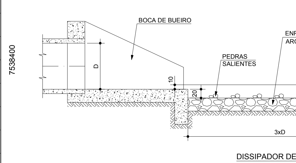
DISSIPADOR DE ENERGIA
