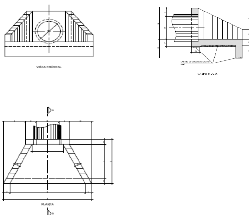
Ilustração 8.9 – Ala de Saída.
