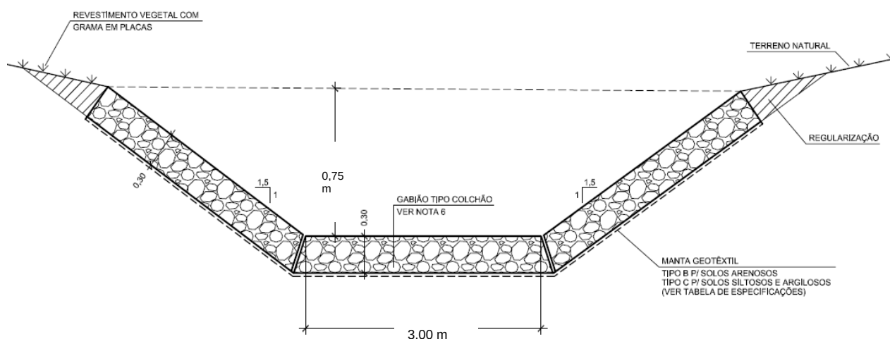
Ilustração 8.12 – Ilustração da seção planejada para o canal trapezoidal .
