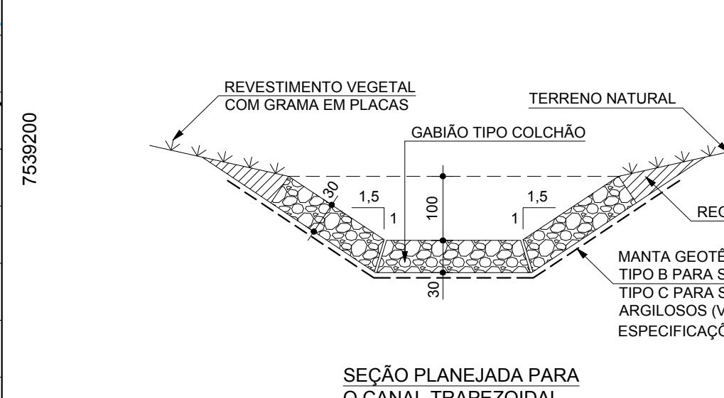
SEÇÃO PLANEJADA PARA O CANAL TRAPEZOIDAL
