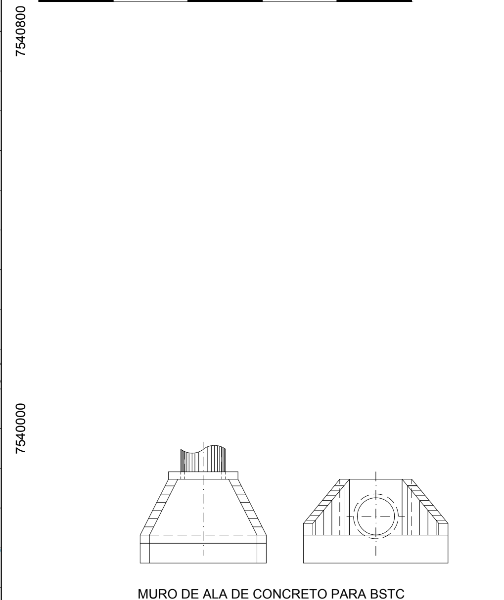
MURO DE ALA DE CONCRETO PARA BSTC
