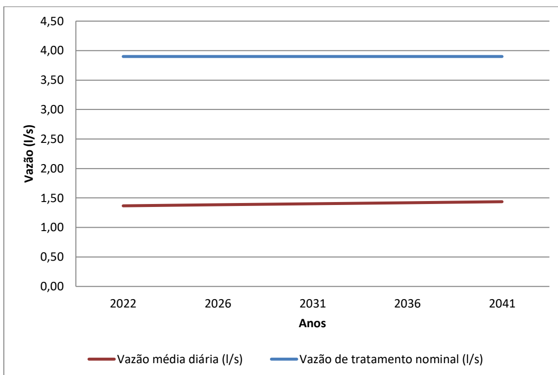
Gráfico 8.8 – Contribuição Média Diária (l/s) x Capacidade nominal da ETE (l/s)
