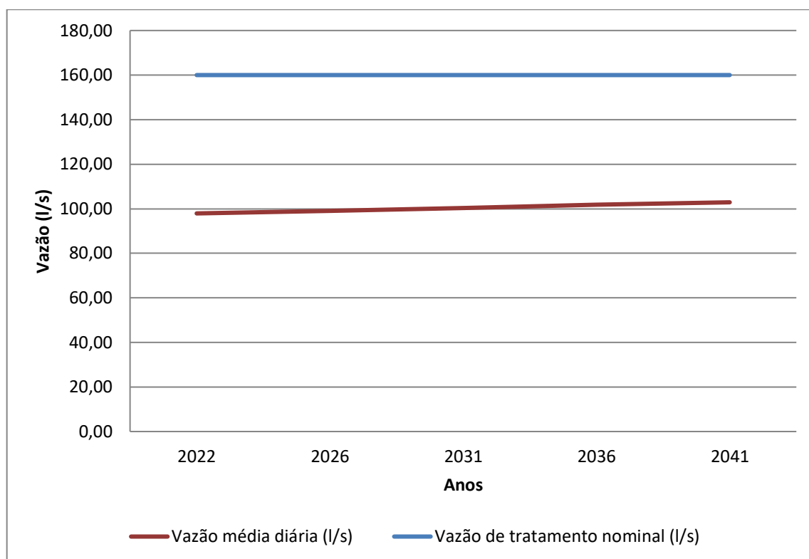
Gráfico 8.5 – Contribuição Média Diária (l/s) x Capacidade Nominal da ETE (l/s)
