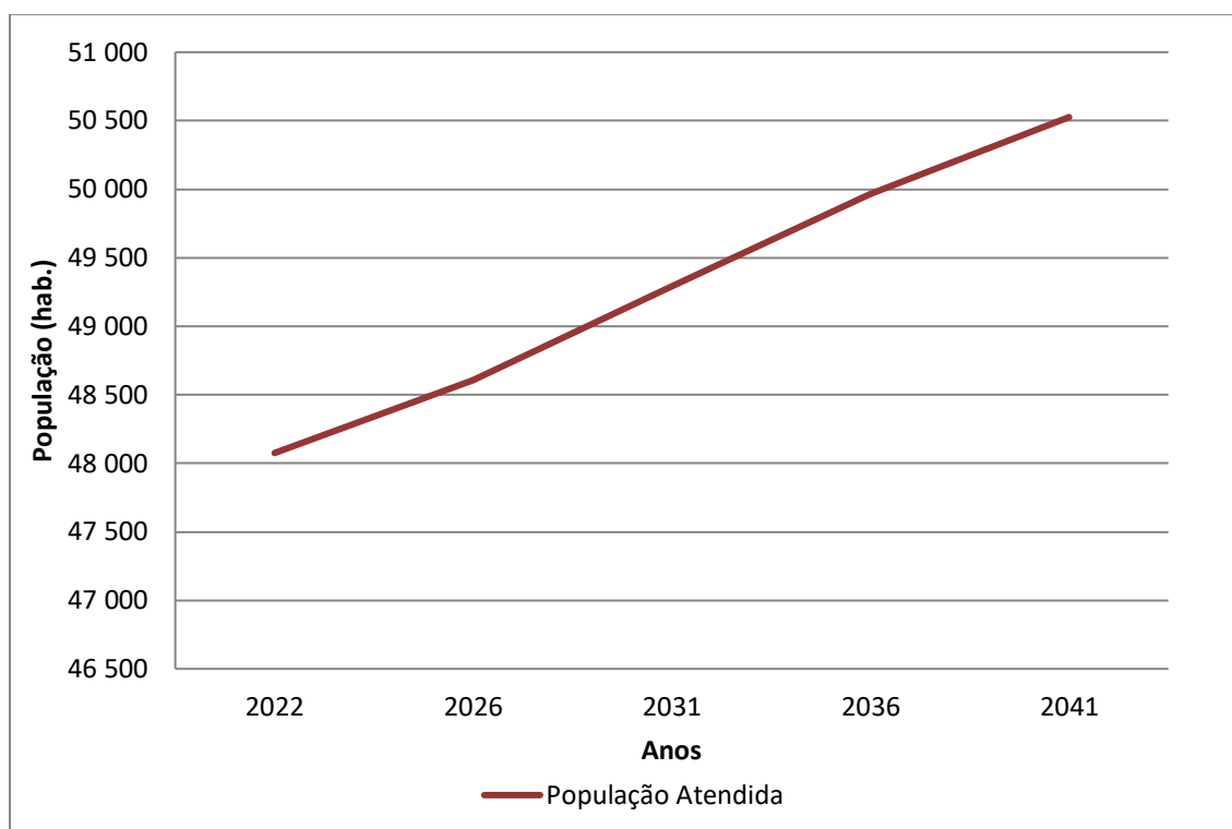
Gráfico 7.2 – População Atendida (hab.) x Anos de Planejamento – Sede Urbana + Bairro Arapongal
