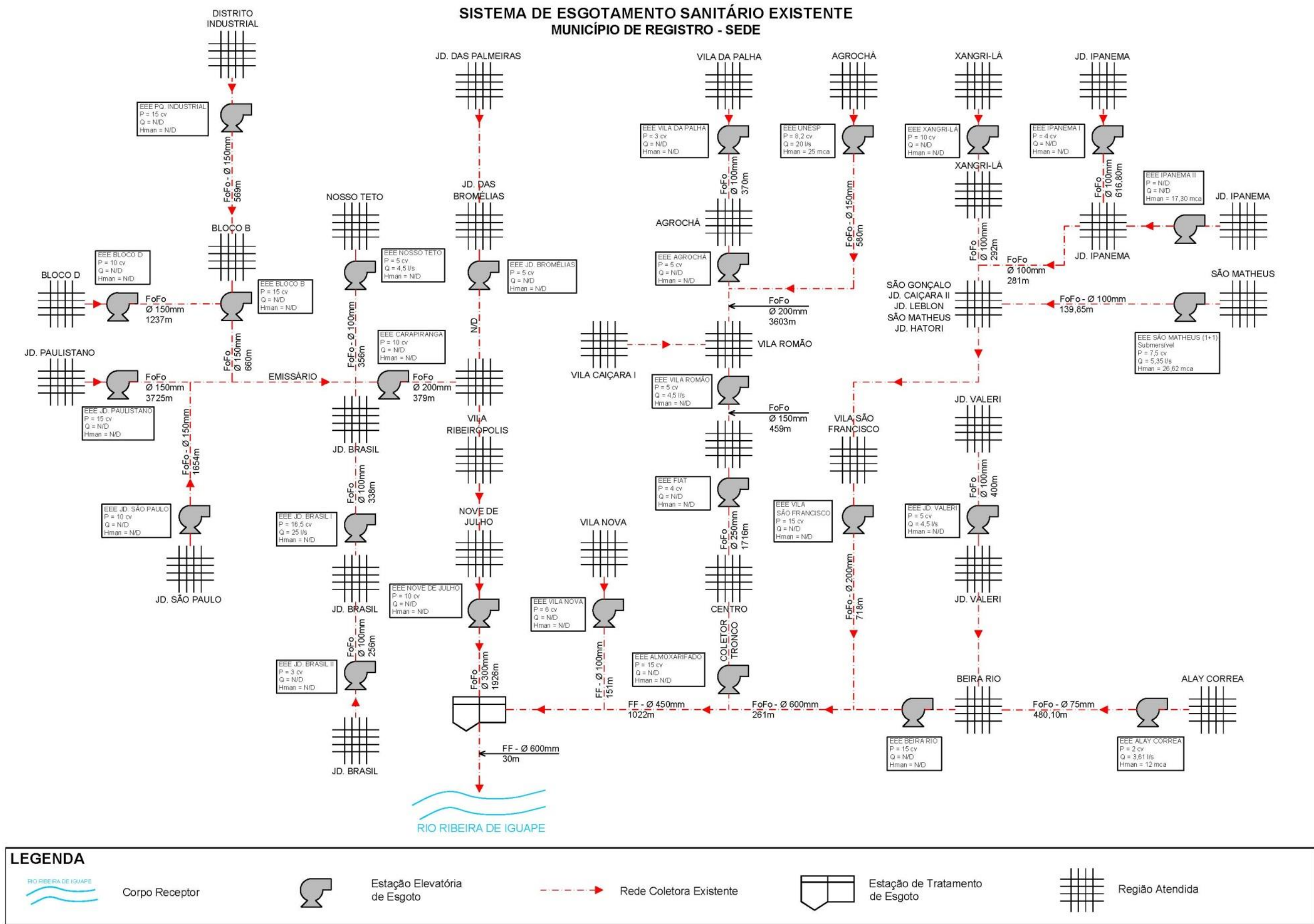
Figura 4.3 – Croqui do Sistema de Esgotamento Sanitário Existente – Sede Urbana
