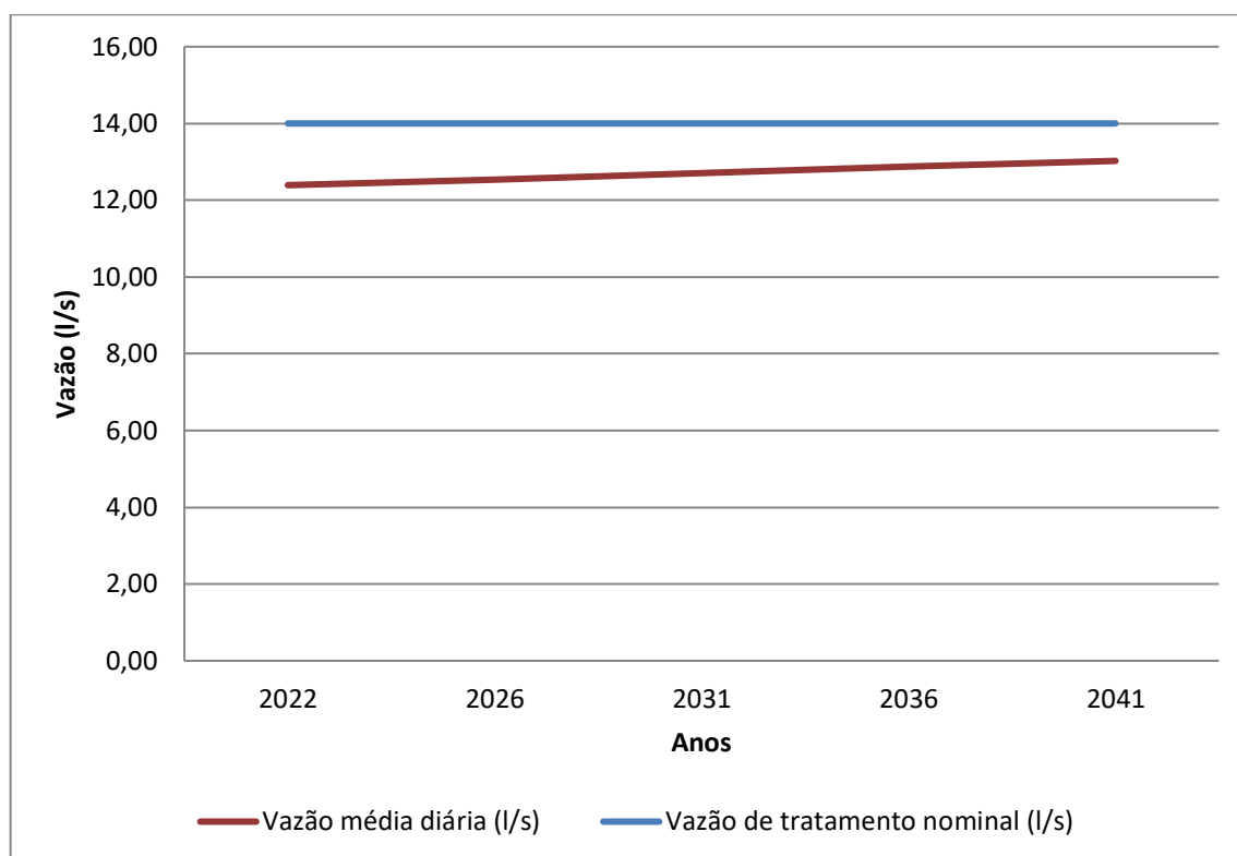
Gráfico 8.7 – Contribuição Média Diária (l/s) x Capacidade nominal da ETE (l/s)
