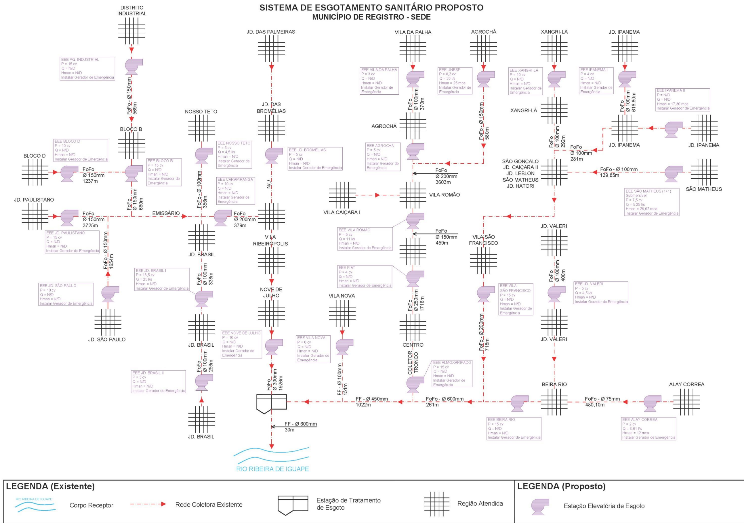
Figura 10.2 – Croqui do Sistema de Esgotamento Sanitário Proposto para o Subsistema da Sede Urbana
