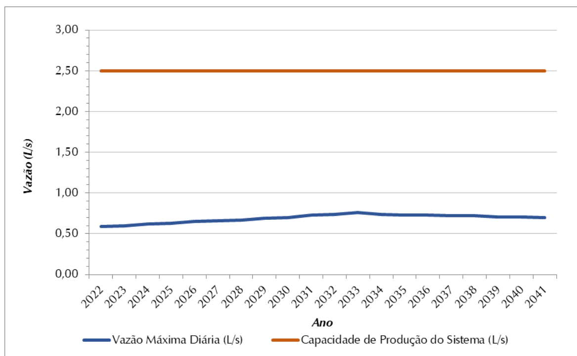
Figura 8.3 – Demandas Máximas Diárias (L/s) X Vazão Captada (L/s) – SAA Saltinho
