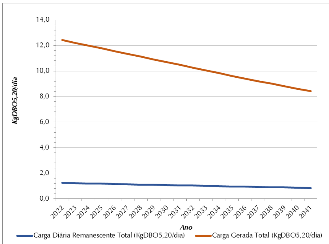
Figura 8.10 - Evolução de Cargas Orgânicas (Kg DBO 5,20 /Dia)
