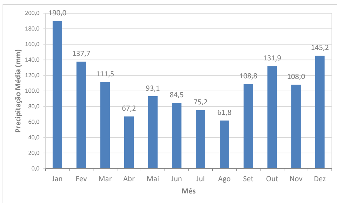
Figura 3.2 - Precipitação Média Mensal no Período de 1975 a 2020, Estação F-012
