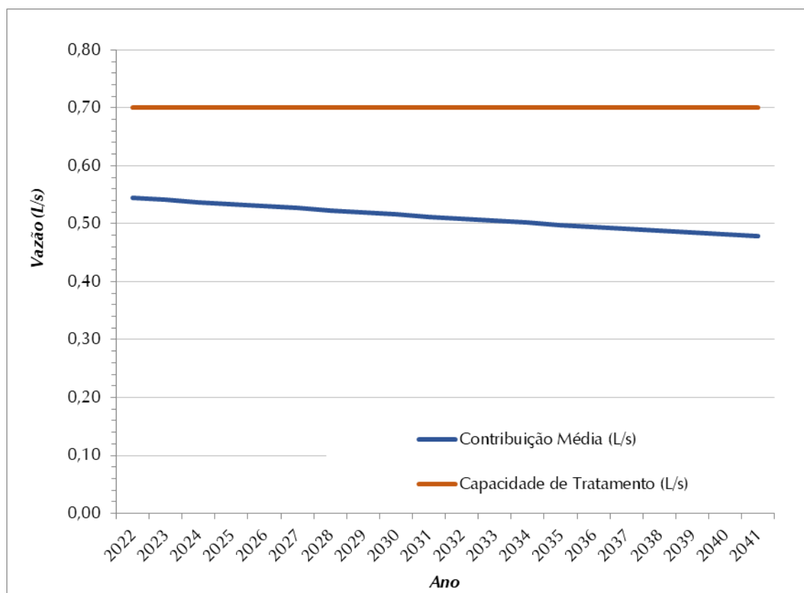
Figura 8.9 – Contribuição Média Total (L/s) x Capacidade de Tratamento de Esgoto (L/s) – SES Saltinho
