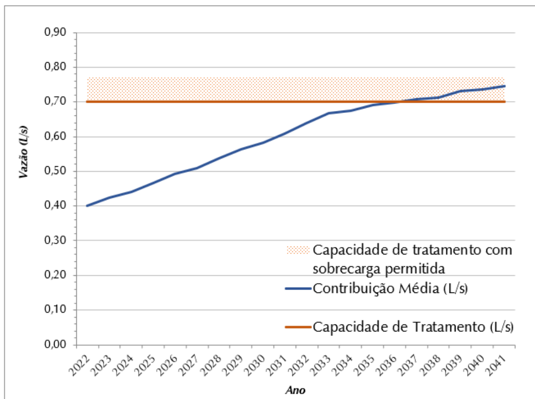
Figura 8.7 – Contribuição Média Total (L/s) x Capacidade de Tratamento de Esgoto (L/s) – SES Vila Ito
