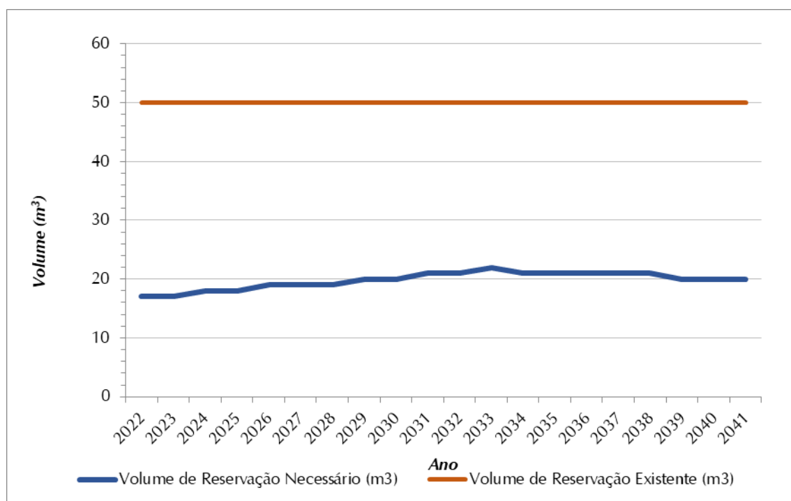
Figura 8.4 - Volume de Reservação Necessário (m³) x Volume de Reservação Atual (m³) SAA Saltinho
