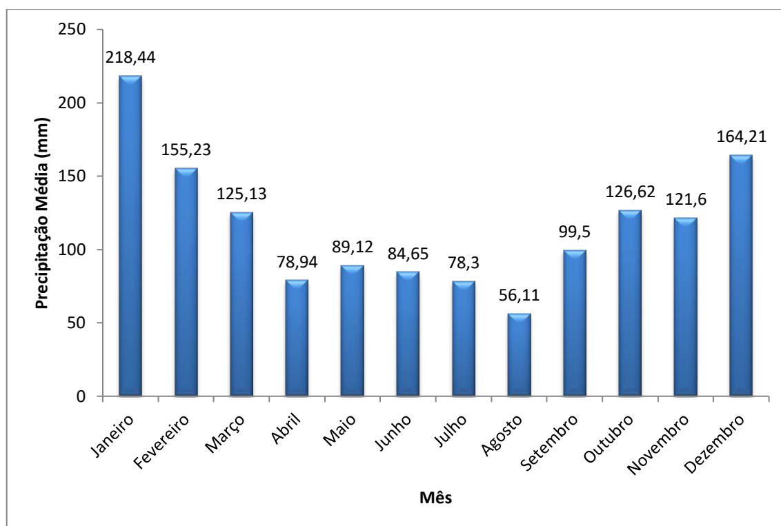
Gráfico 3.1 – Precipitação Média Mensal no Período de 1966 a 2020, Estação F5-027
