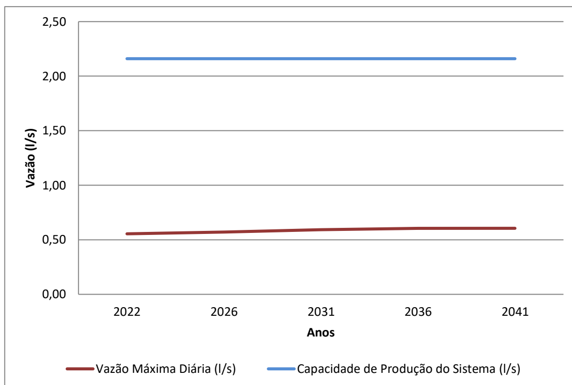
Gráfico 8.2 – Demandas Máximas Diárias (l/s) X Capacidade de Produção do Sistema (l/s)
