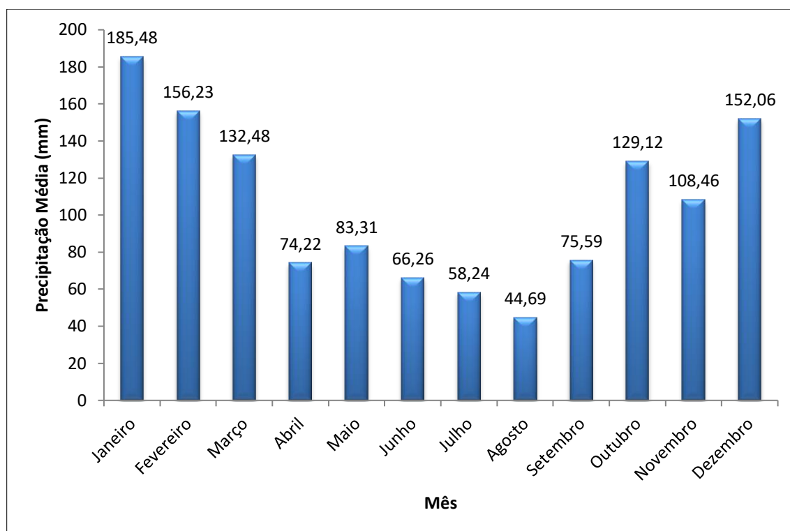
Gráfico 3.1 – Precipitação Média Mensal no Período de 1947 a 2004, Estação F5-025
