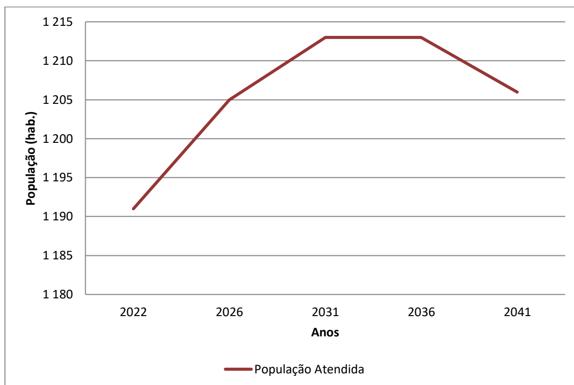
Gráfico 7.6 - População Atendida (hab.) x Anos de Planejamento – Bairro Boa Vista
