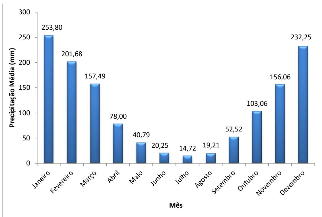
Gráfico 3.1 – Precipitação Média Mensal no Período de 1939 a 2000, Estação A6-001
