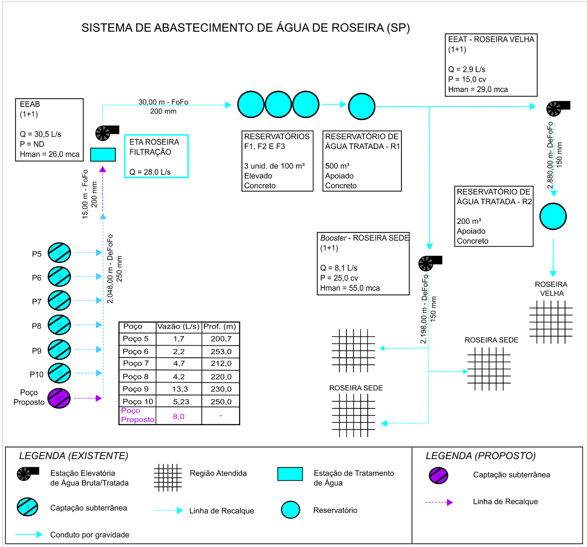
Figura 10.1 – Croqui do sistema de abastecimento de água proposto para Sede
