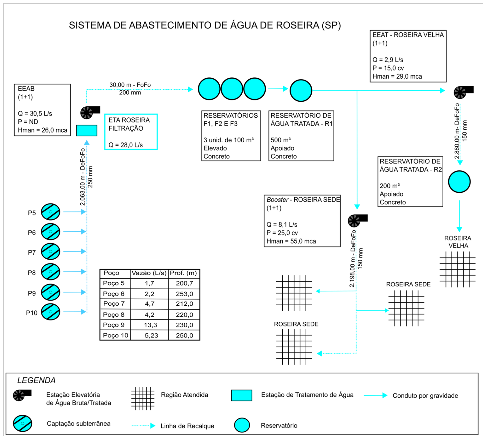
Figura 4.1 – Croqui do Sistema de Abastecimento de Água Sede
