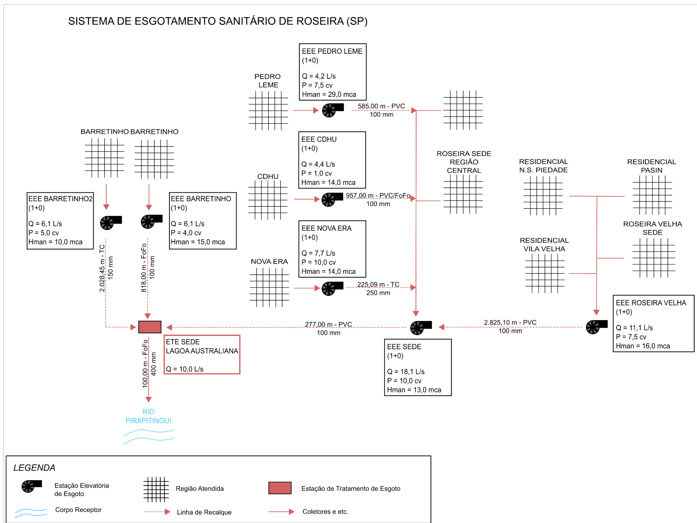
Figura 4.2 – Croqui do Sistema de Esgotamento Sanitário da Sede de Roseira.
