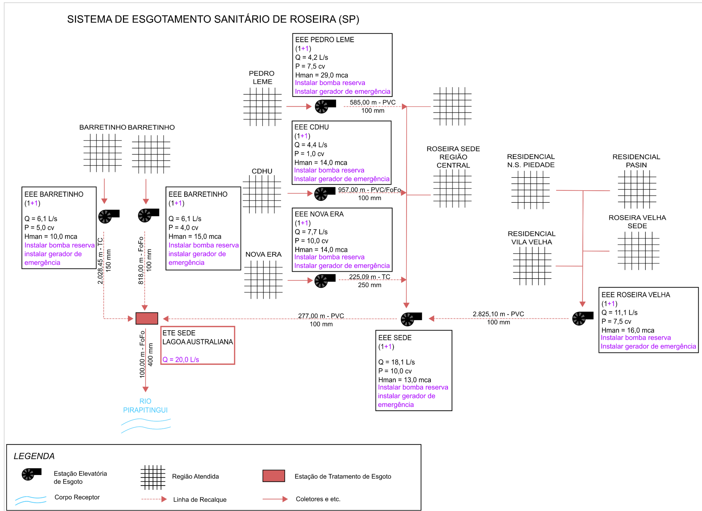
Figura 10.2 – Croqui das intervenções propostas para o sistema de esgotamento sanitário Sede
