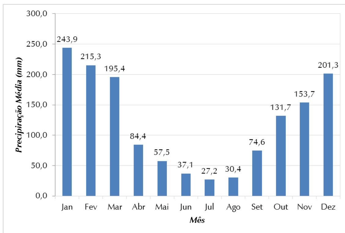
Figura 3.2 - Precipitação Média Mensal no Período de 1943 a 2016, Estação E2-025
