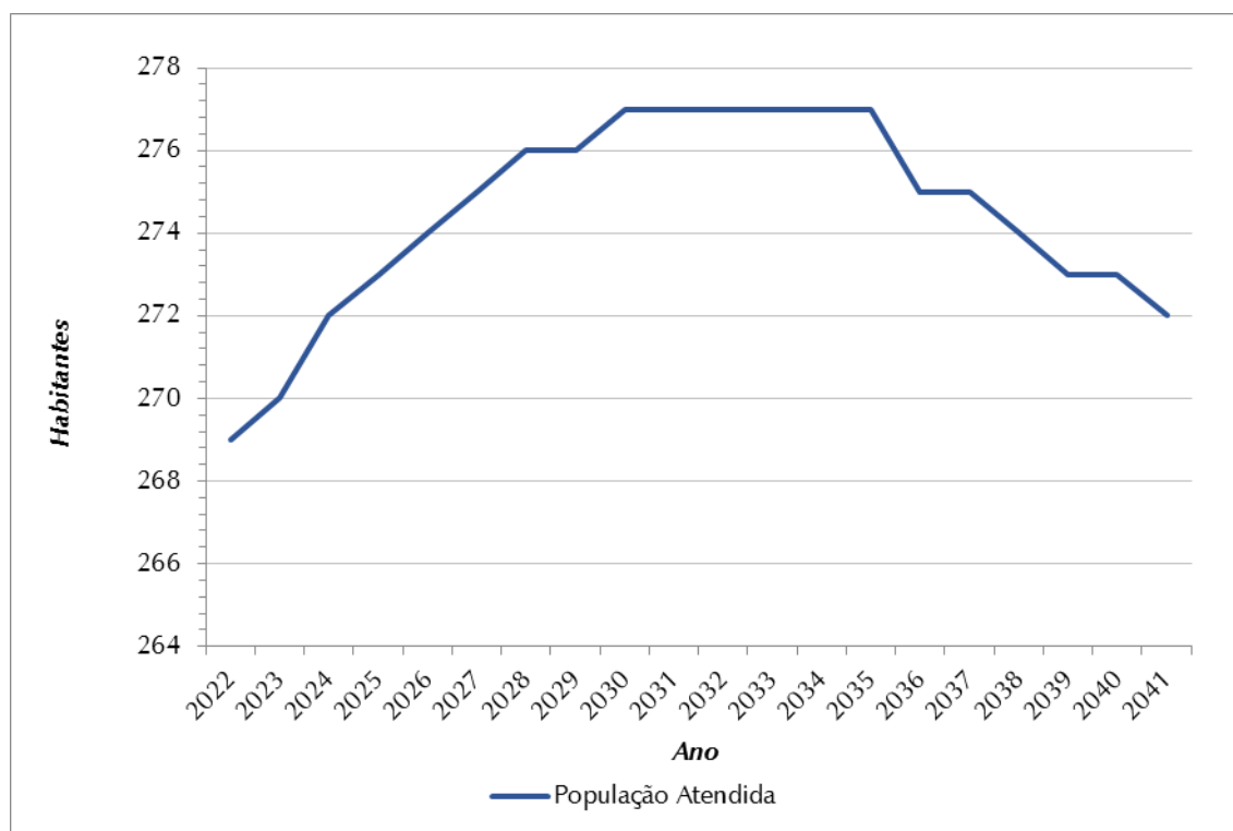
Figura 7.3 – Evolução da População Atendida (hab.) – SAA Esmeralda
