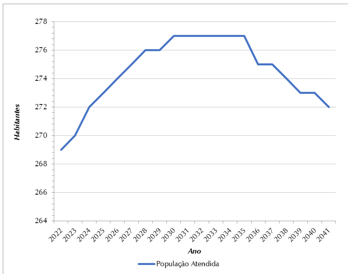
Figura 7.5 - Evolução da População Atendida (hab.) – SES Esmeralda
