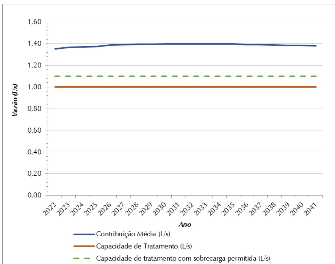
Figura 8.7 – Contribuição Média Total (L/s) x Capacidade de Tratamento de Esgoto (L/s) – SES Esmeralda
