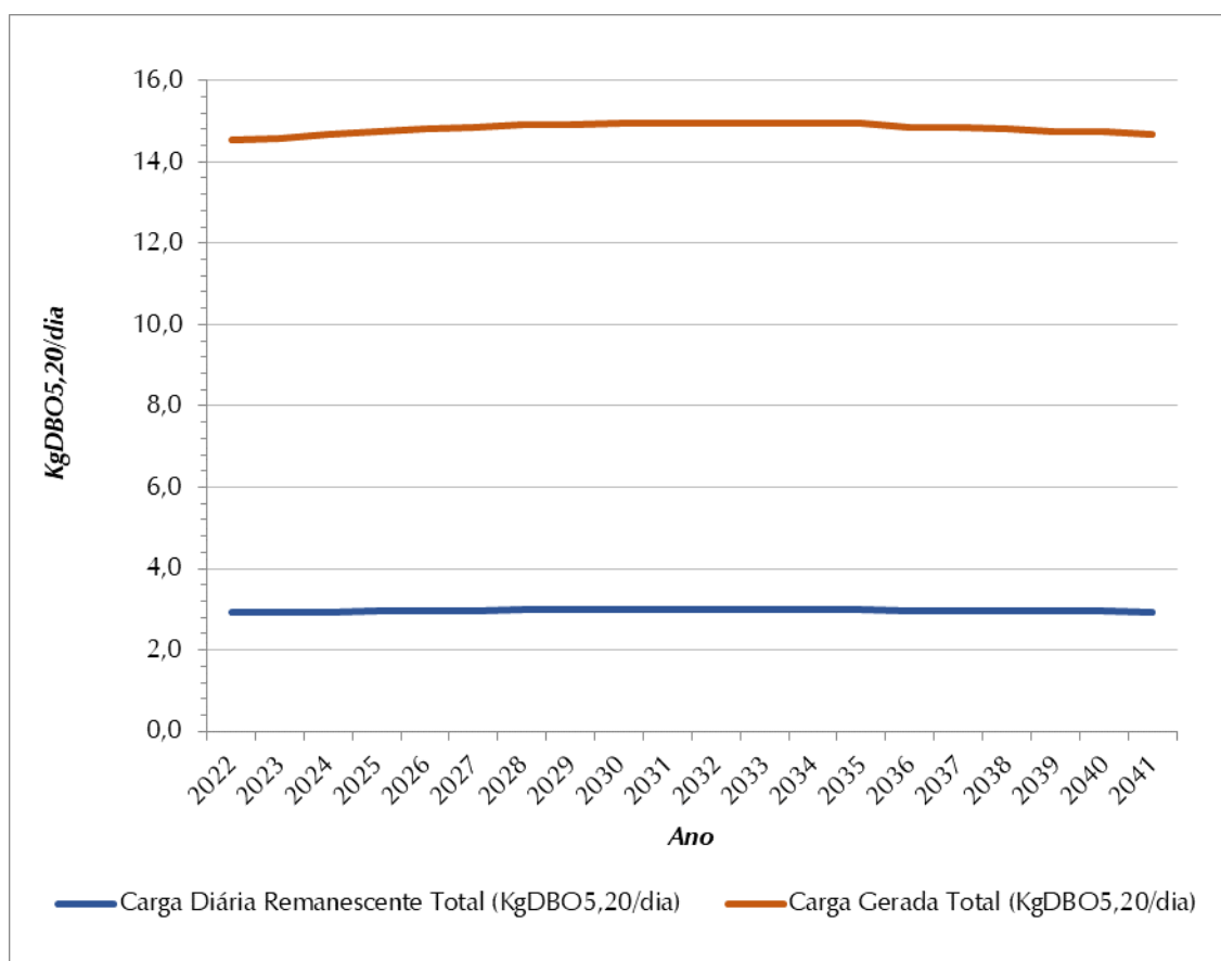
Figura 8.8 - Evolução de Cargas Orgânicas (Kg DBO 5,20 /Dia) – SES Esmeralda
