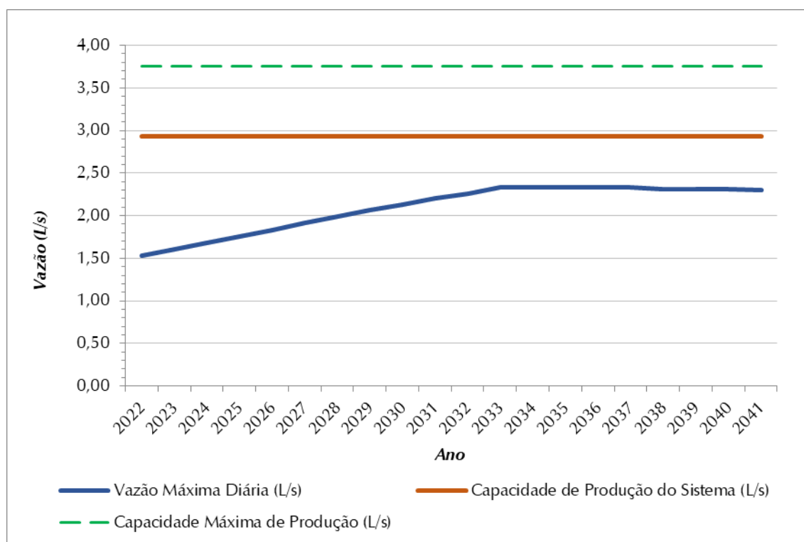
Figura 8.3 – Demandas Máximas Diárias (L/s) X Vazão Captada (L/s) – SAA Esmeralda
