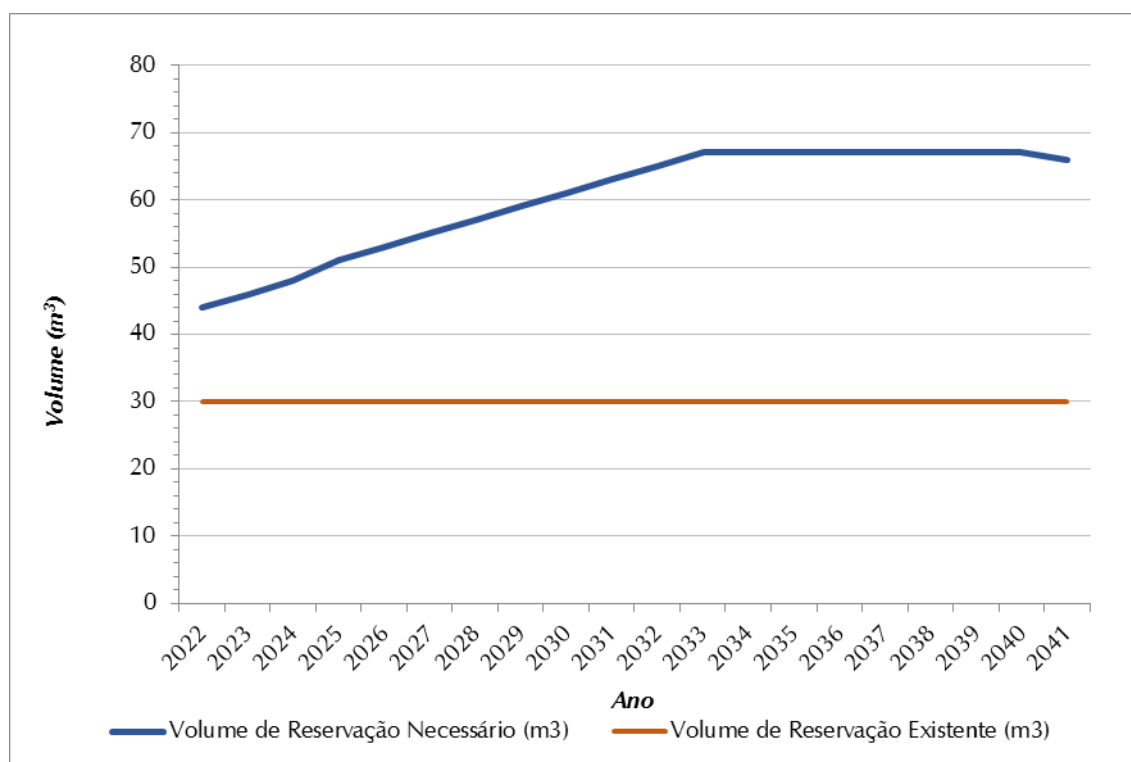
Figura 8.4 - Volume de Reservação Necessário (m³) x Volume de Reservação Atual (m³) - SAA Esmeralda
