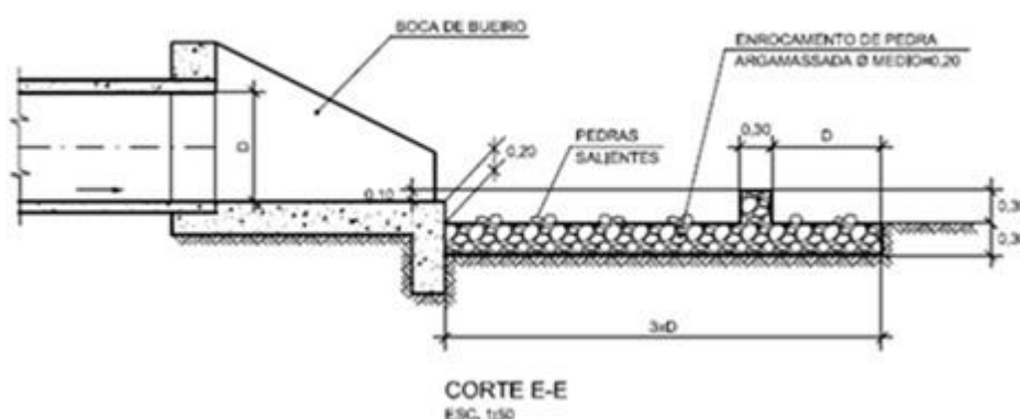
Ilustração 8.8 - Dissipador
