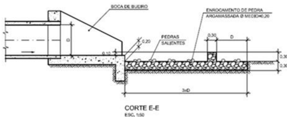
Ilustração 8.9 - Dissipador
