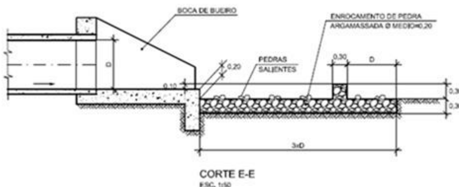
Ilustração 8.7 – Dissipador.
