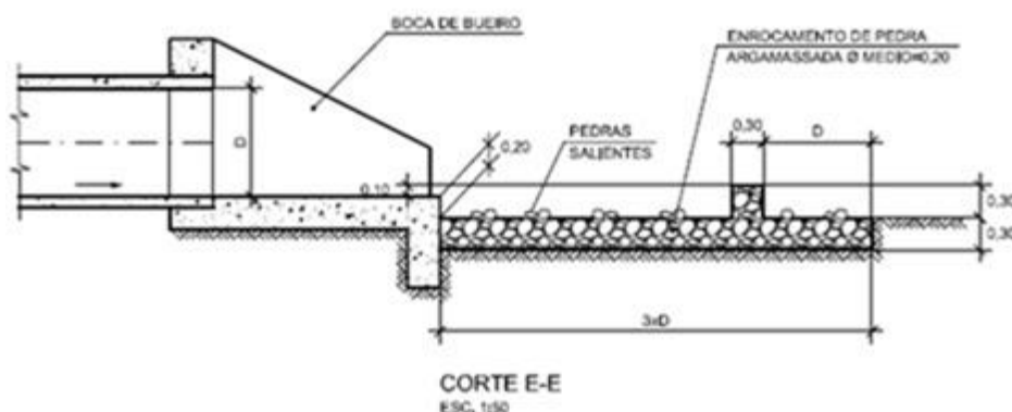
Ilustração 8.4- – Dissipador previsto.
