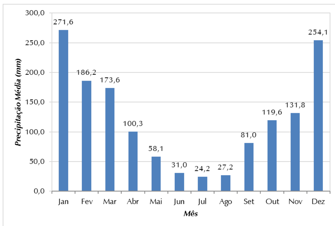
Figura 3.2 - Precipitação Média Mensal no Período de 1971 a 2001, Estação B7-052
