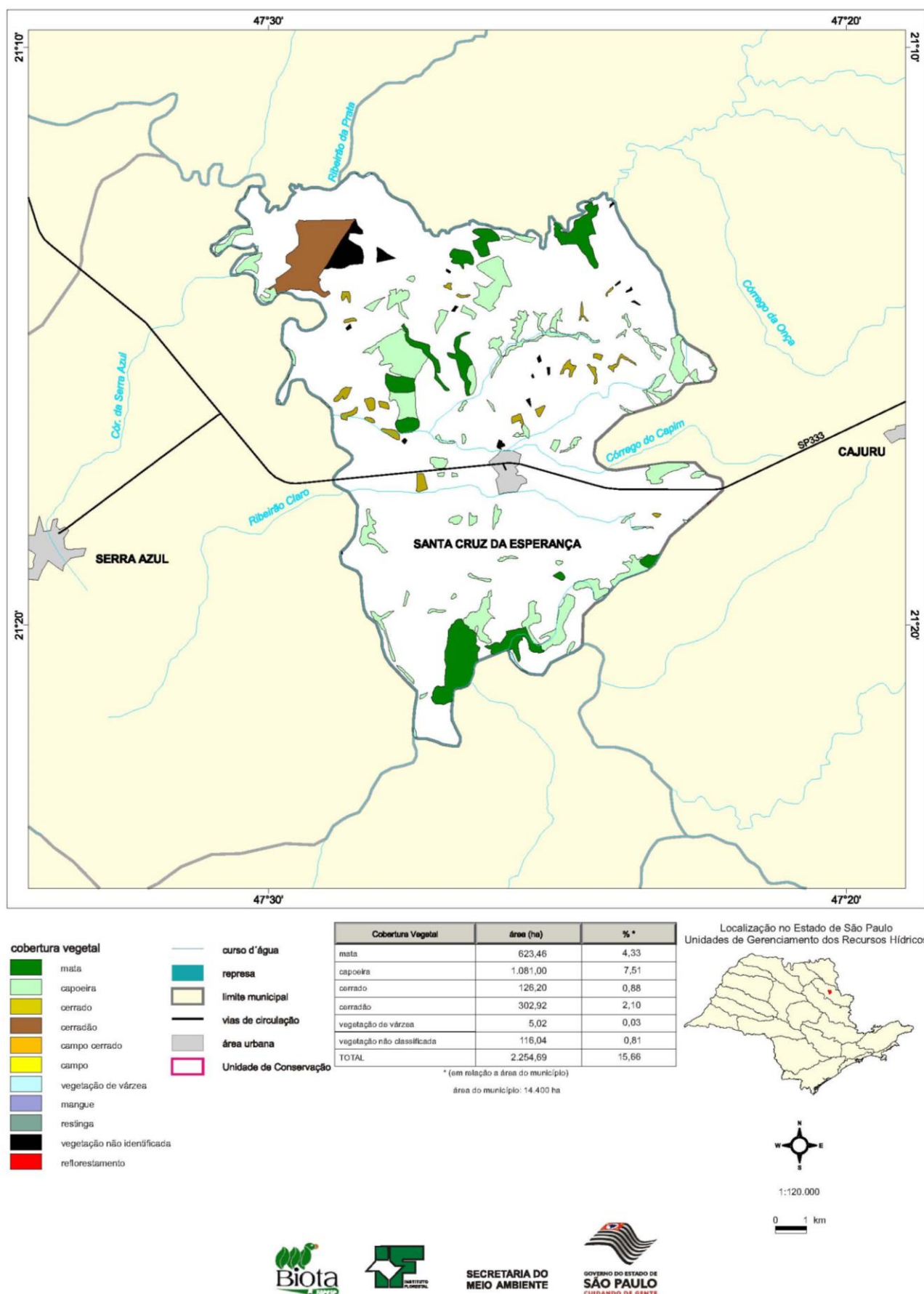
Figura 3.2 – Cobertura Vegetal no Município de Santa Cruz da Esperança
