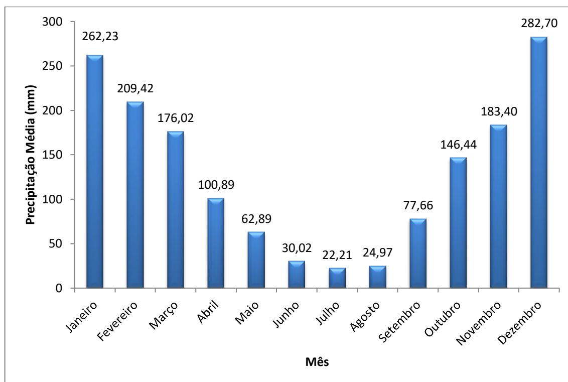
Gráfico 3.1 – Precipitação Média Mensal no Período de 1973 a 2000, Estação C4 105
