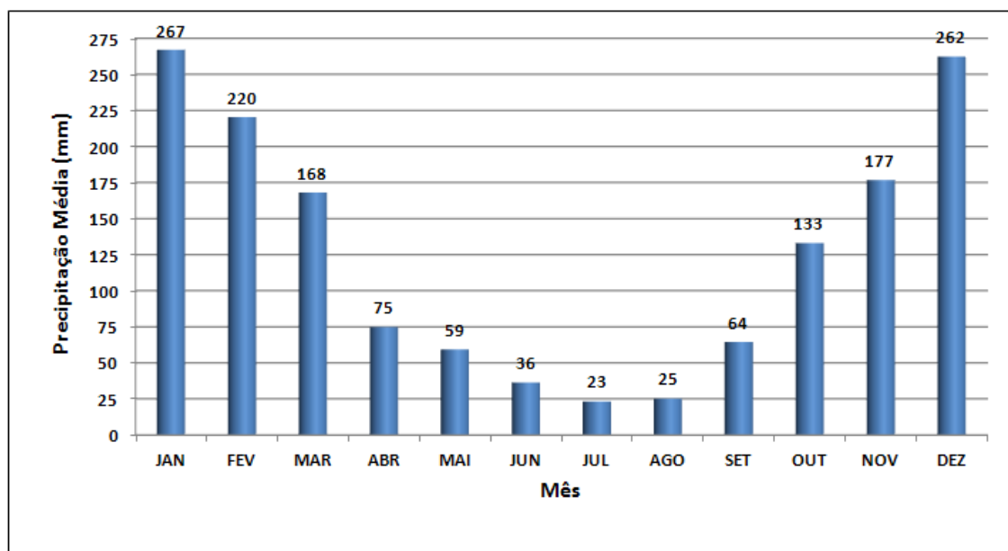
Gráfico 2.1 - Precipitação Média Mensal no Período de 1936 a 2000, Estação C4-029
