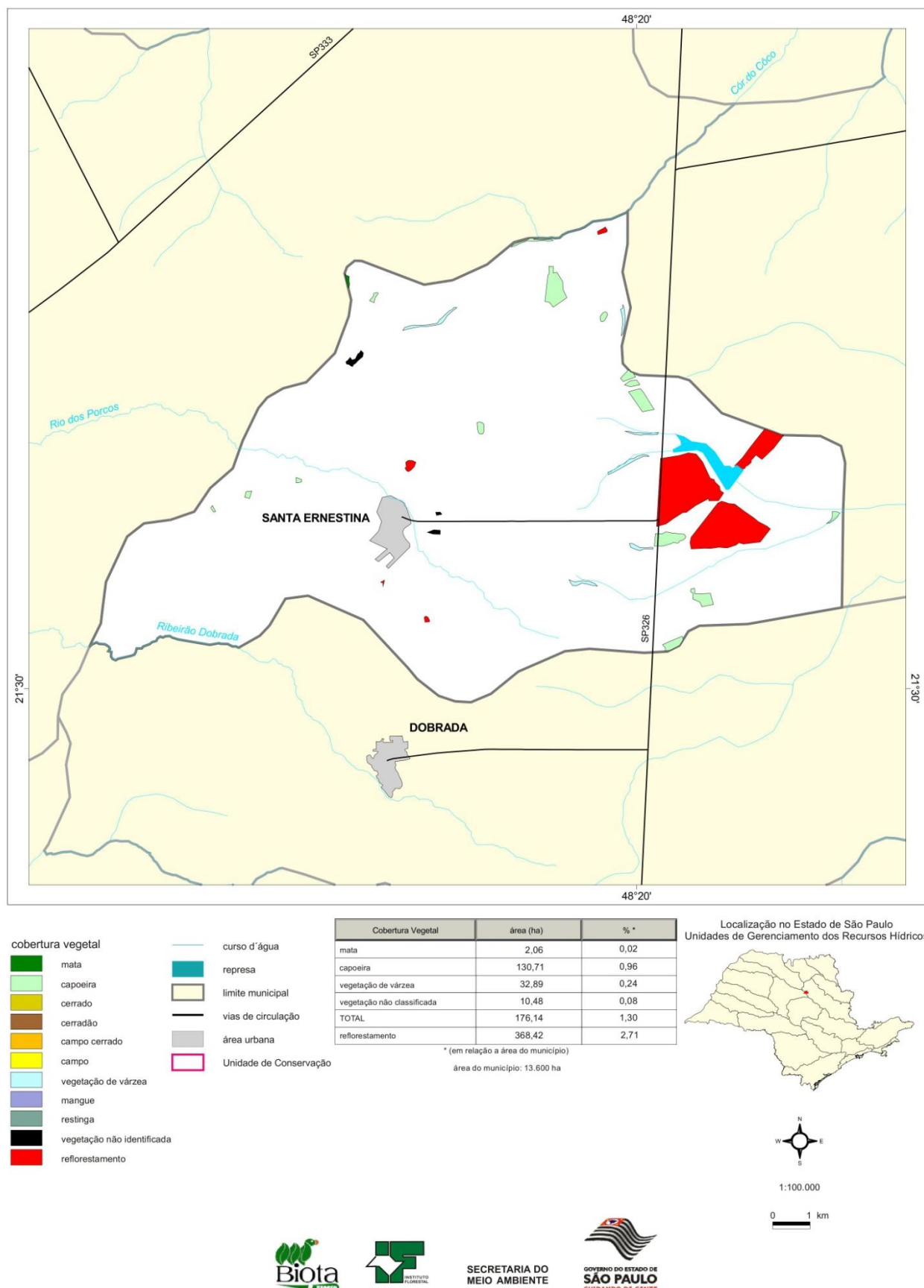
Figura 3.2 – Cobertura Vegetal no Município de Santa Ernestina
