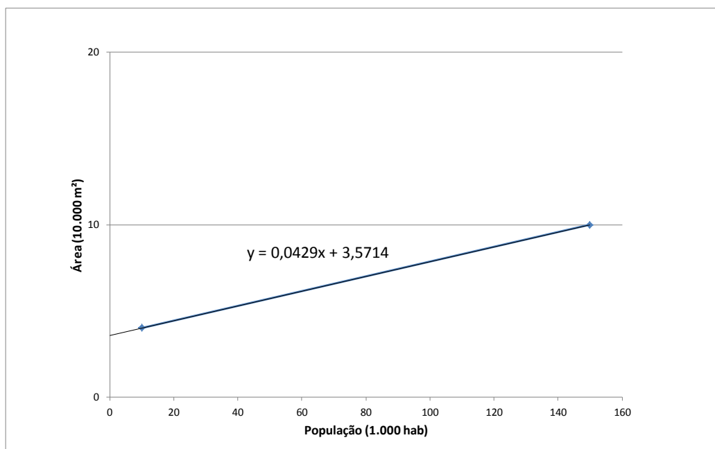
Gráfico 6.2 – Variação da área do terreno do ATS em função da população
