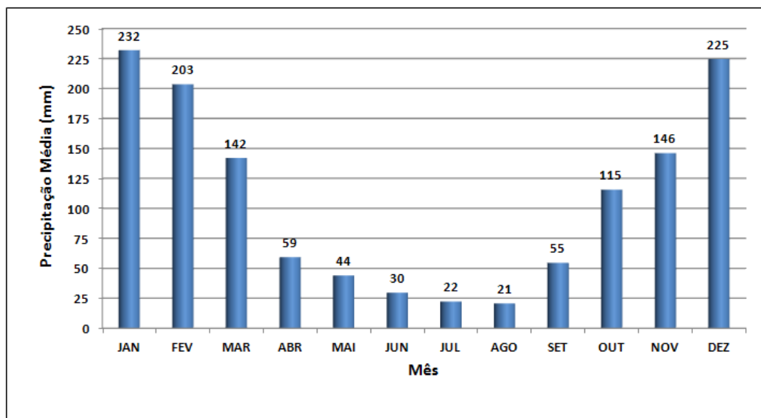
Gráfico 2.1 - Precipitação Média Mensal no Período de 1936 a 2004, Estação C5-011
