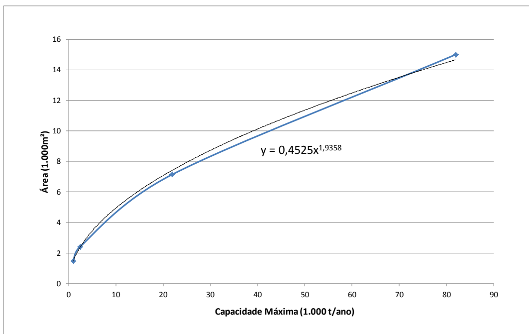
Gráfico 6.1 – Variação da área do terreno da UC em função da capacidade
