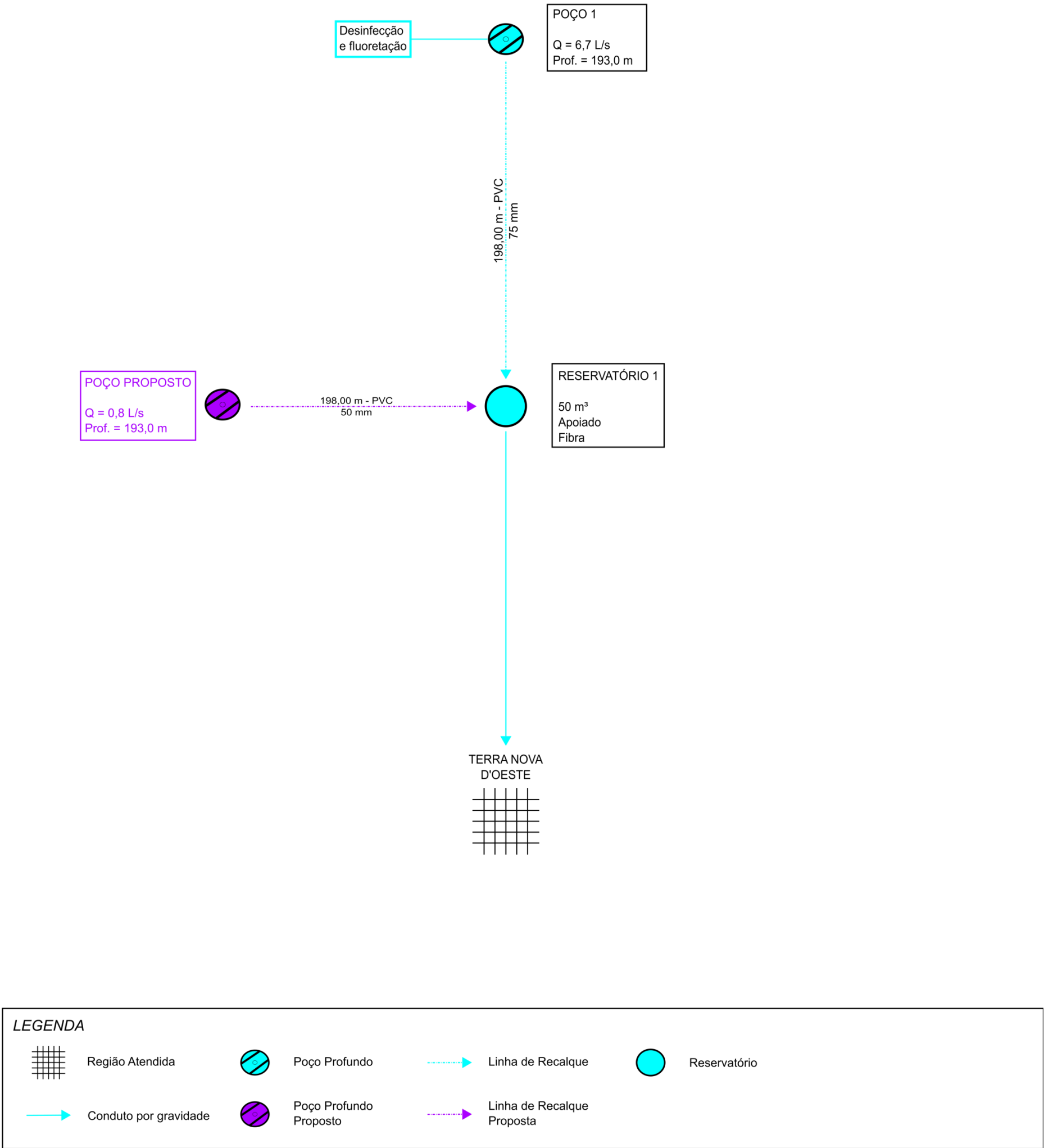
Figura 10.2 – Croqui das intervenções propostas para o sistema de abastecimento de água Terra Nova d'Oeste
