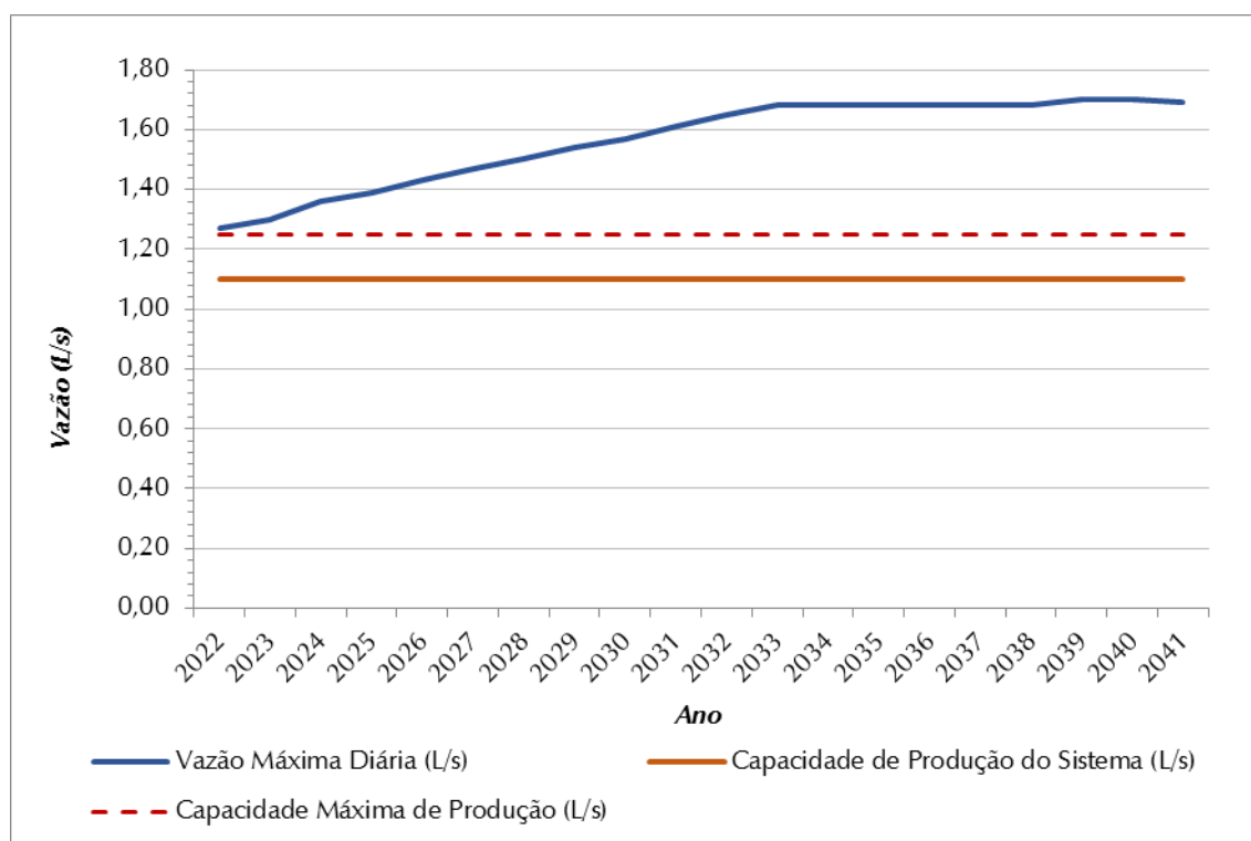
Figura 8.3 – Demandas Máximas Diárias (L/s) X Vazão Captada (L/s) – SAA Terra Nova d'Oeste
