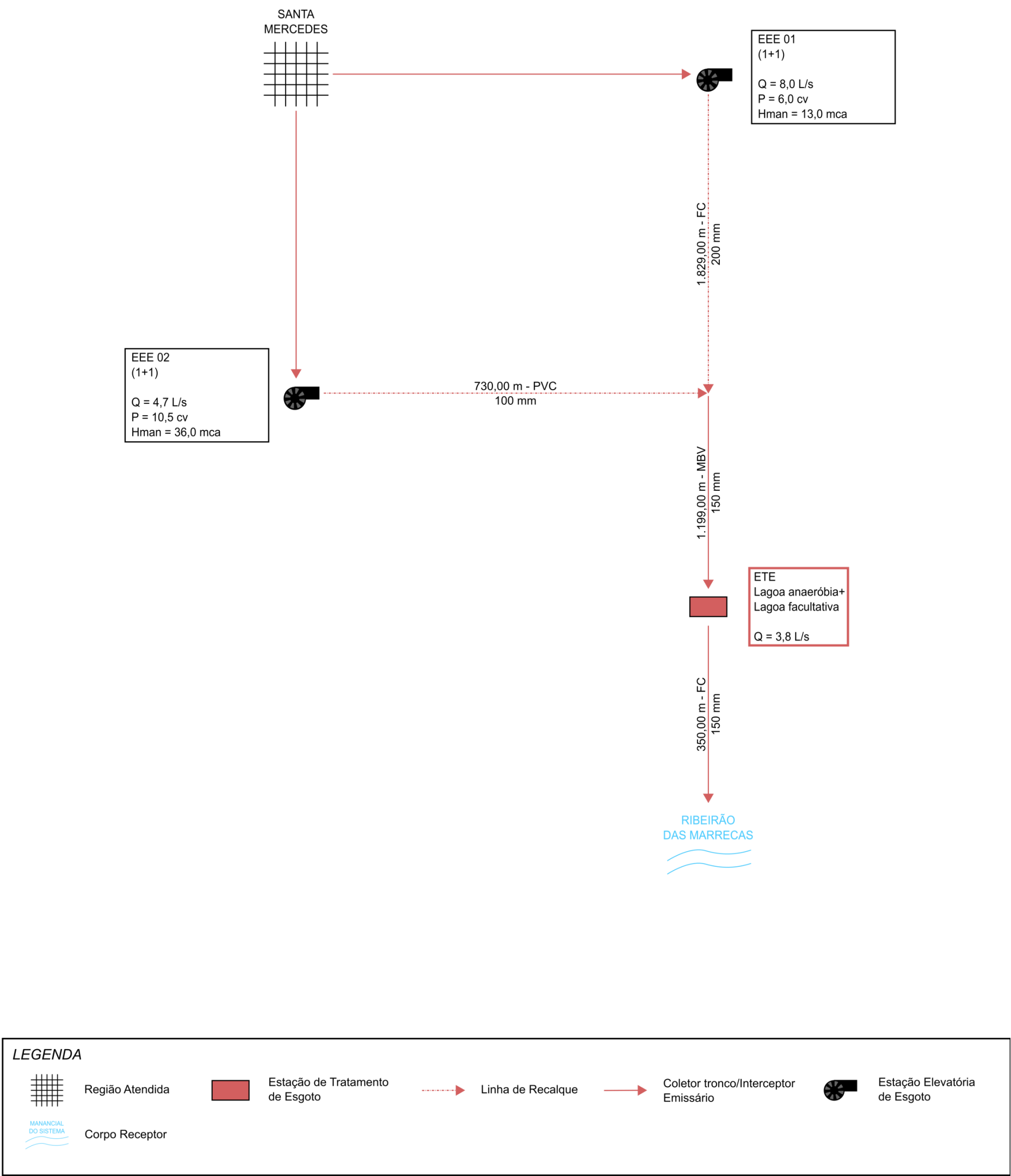
Figura 4.3 – Croqui do Sistema de Esgotamento Sanitário da Sede de Santa Mercedes
