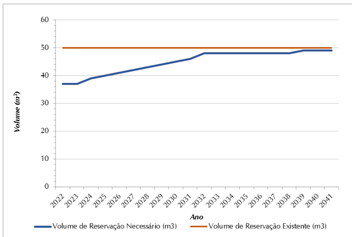
Figura 8.4 - Volume de Reservação Necessário (m³) x Volume de Reservação Atual (m³) - SAA Terra Nova d'Oeste
