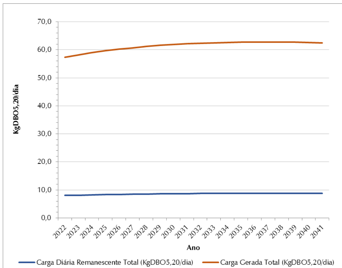
Figura 8.3 - Evolução de Cargas Orgânicas (Kg DBO 5,20 /Dia)
