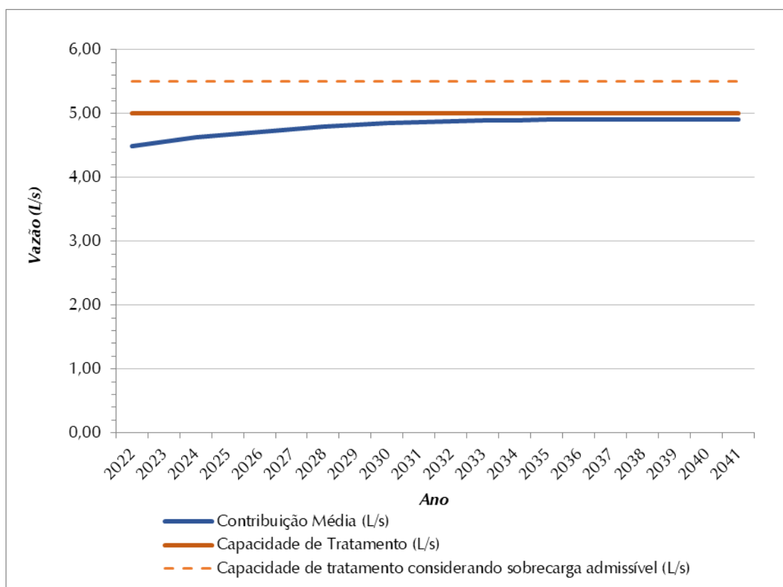
Figura 8.2 – Contribuição Média Total (L/s) x Capacidade de Tratamento de Esgoto (L/s) – SES Sede
