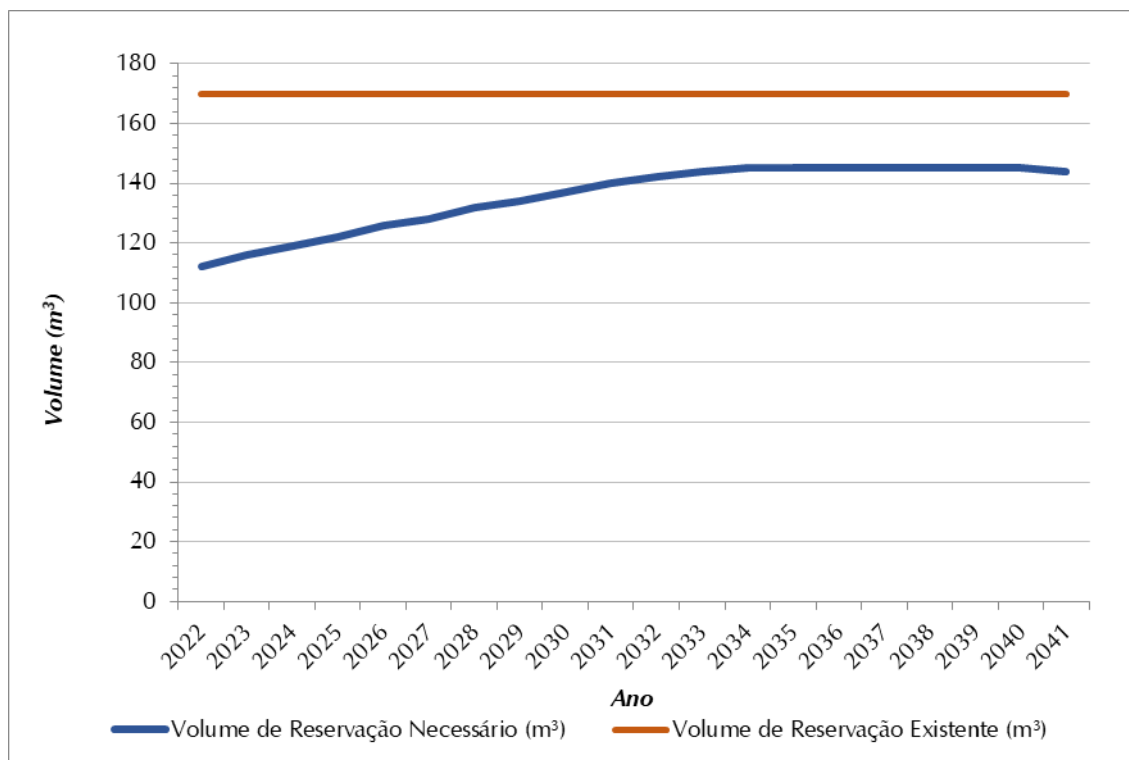
Figura 8.1 - Volume de Reservação Necessário (m³) x Volume de Reservação Atual (m³) SAA Sede
