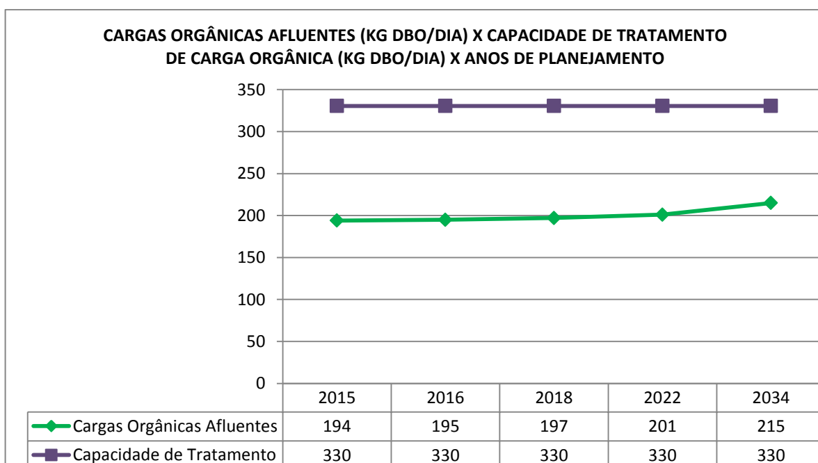
Gráfico 3.6 – Cargas Orgânicas Afluentes (Kg DBO/dia) x Capacidade de Tratamento de Carga Orgânica (kg DBO/dia) x Anos de Planejamento
