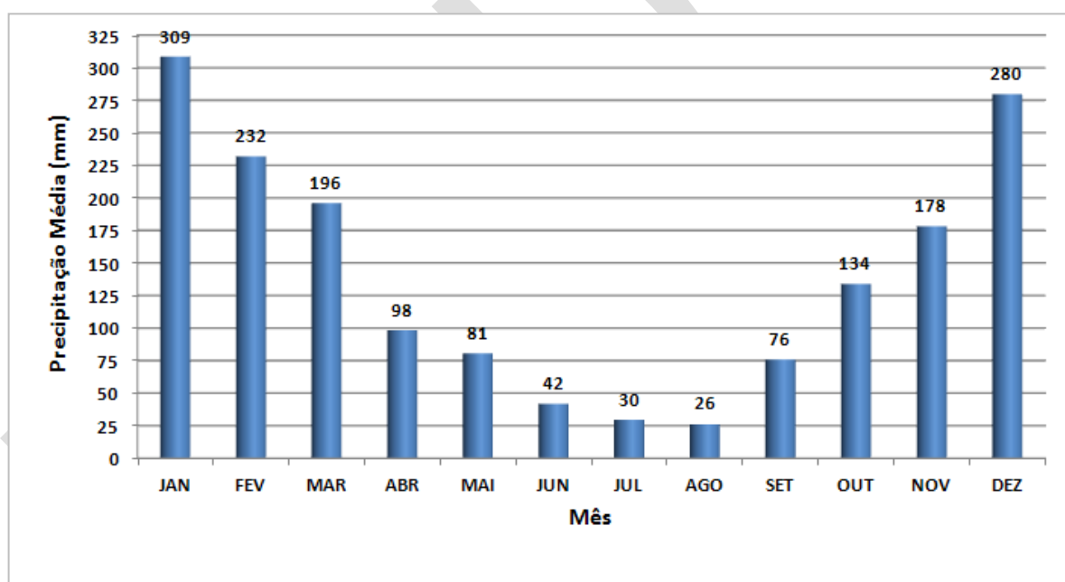
Gráfico 2.1 - Precipitação Média Mensal no Período de 1972 a 2006, Estação D3-071
