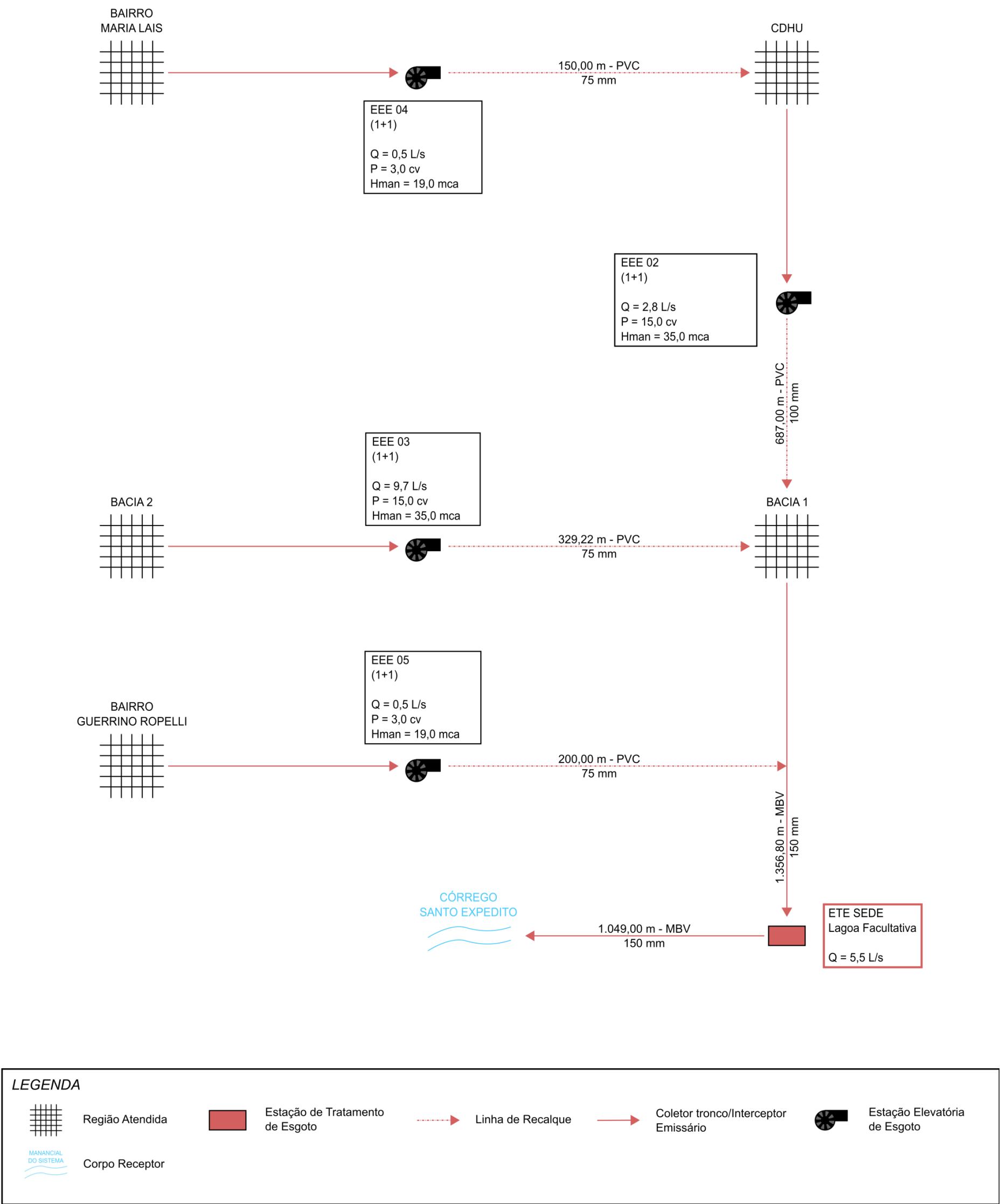
Figura 4.2 – Croqui do Sistema de Esgotamento Sanitário da Sede de Santo Expedito
