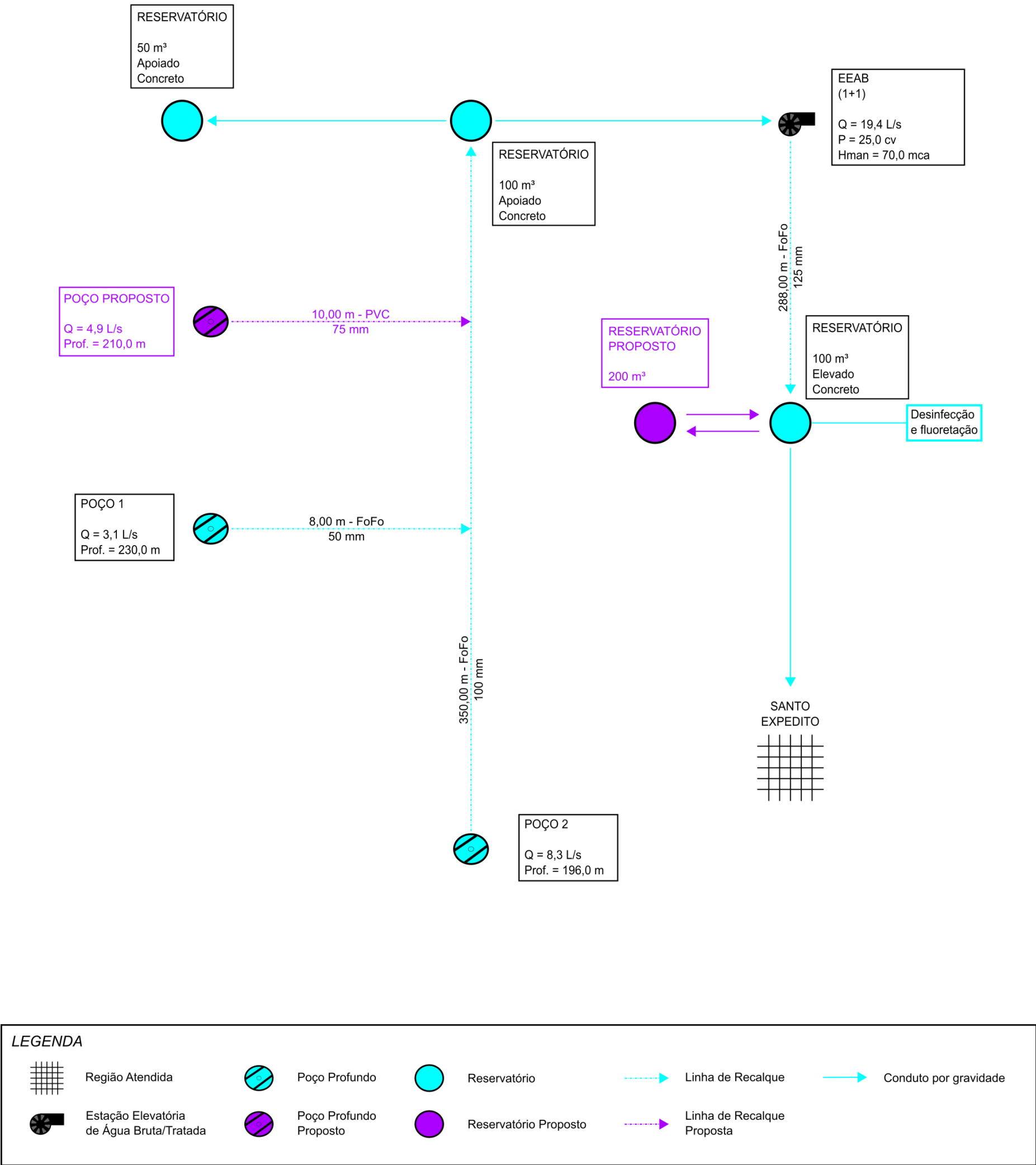
Figura 10.1 – Croqui das intervenções propostas para o Sistema de Abastecimento de Água Sede
