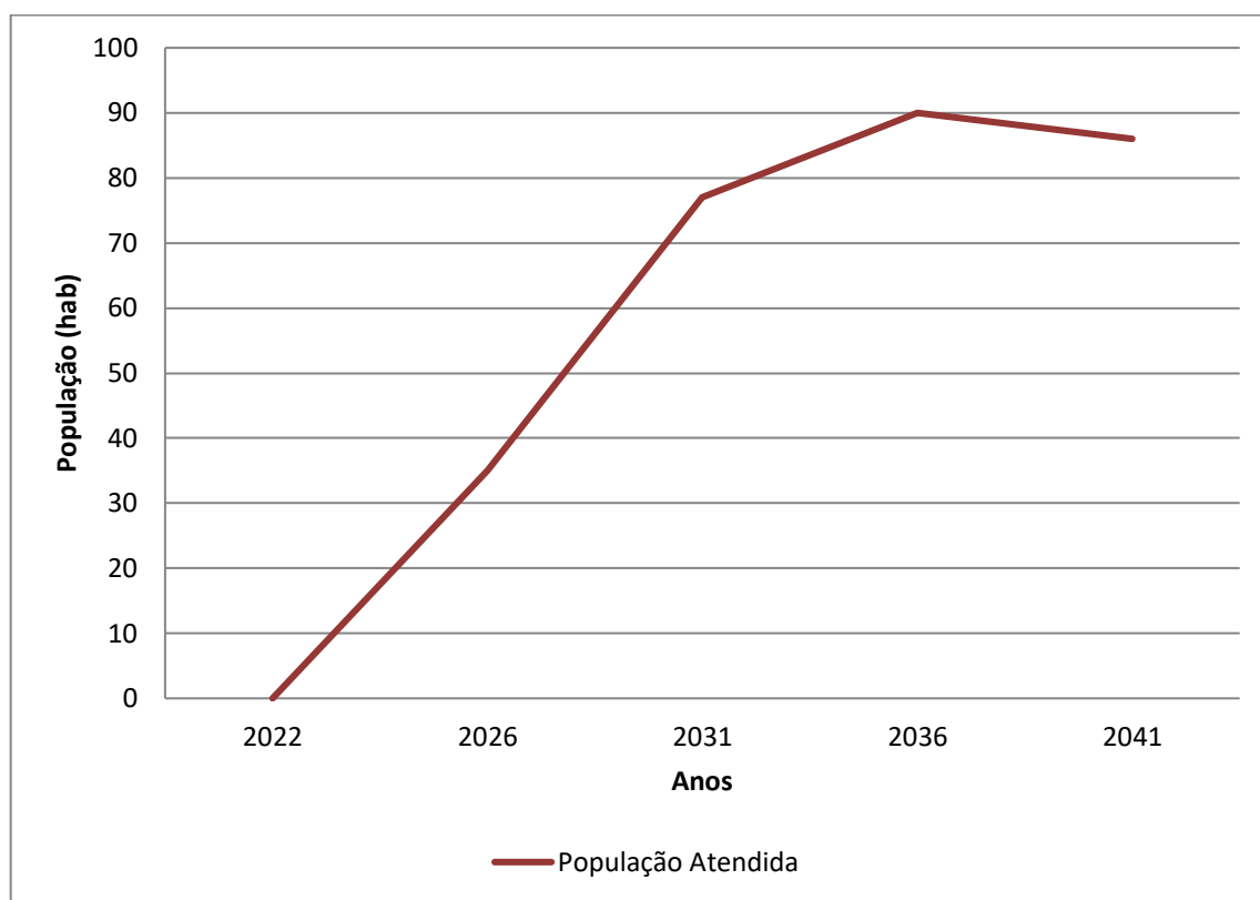
Gráfico 7.13 - População Atendida (hab.) x Anos de Planejamento – Bairro do Dias
