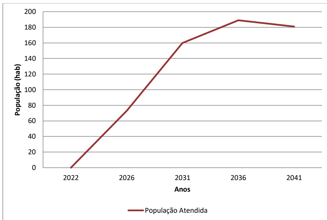
Gráfico 7.7 – População Atendida (hab.) x Anos de Planejamento – Bairro dos Pinheiros
