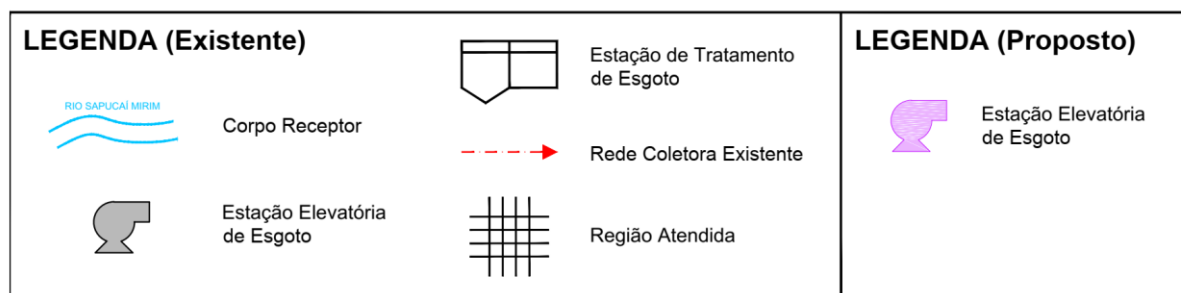
Figura 10.9 – Croqui do Sistema de Esgotamento Sanitário Proposto para o Sistema Sede Urbana/Bairro Quilombo
