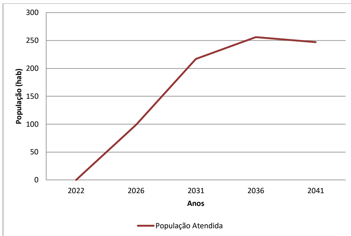
Gráfico 7.9 – População Atendida (hab.) x Anos de Planejamento – Bairro Zé da Rosa
