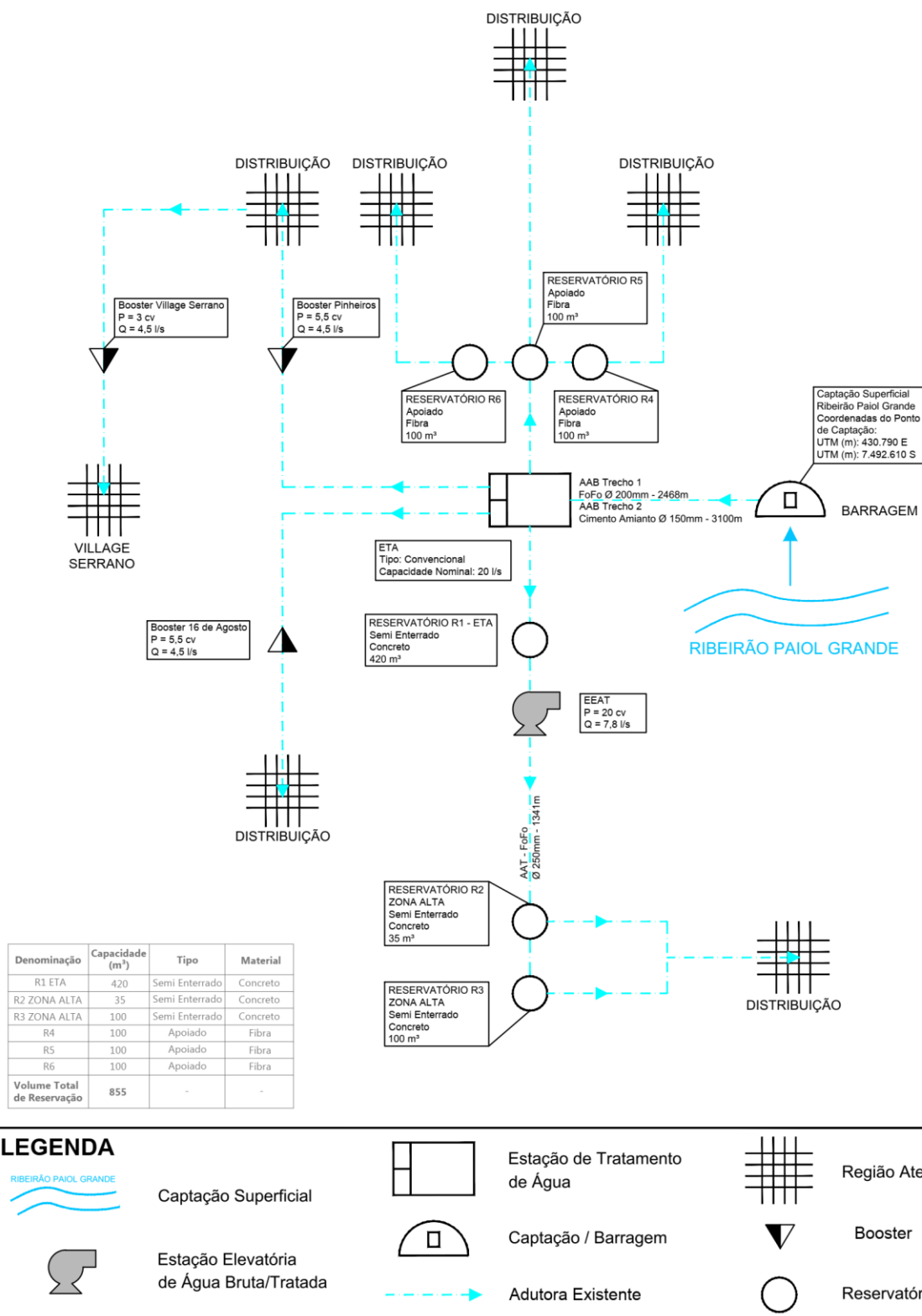
Figura 4.1 – Croqui do Sistema de Abastecimento de Água Existente – Sede Urbana/Bairro Quilombo, Paiol Grande, Serrano e Village Serrano.
