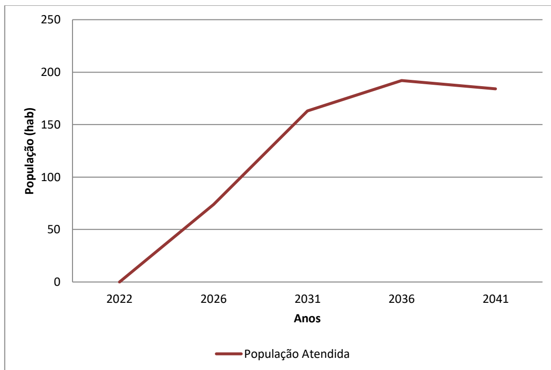
Gráfico 7.8 – População Atendida (hab.) x Anos de Planejamento – Bairro do Sítio
