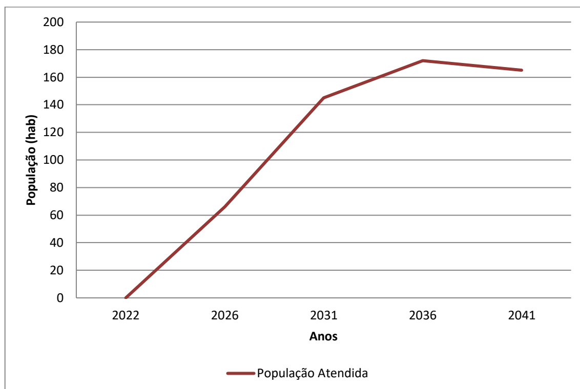
Gráfico 7.17 - População Atendida (hab.) x Anos de Planejamento – Bairro dos Pinheiros
