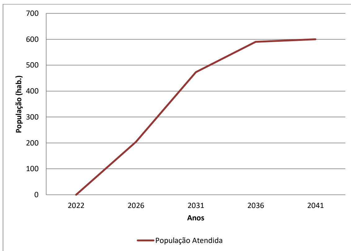
Gráfico 7.12 - População Atendida (hab.) x Anos de Planejamento – Bairro Serrano/Village Serrano
