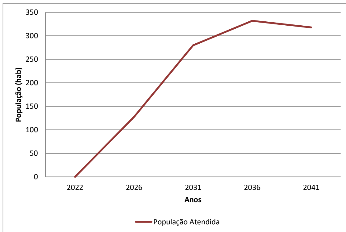
Gráfico 7.4 – População Atendida (hab.) x Anos de Planejamento – Bairro do Dias
